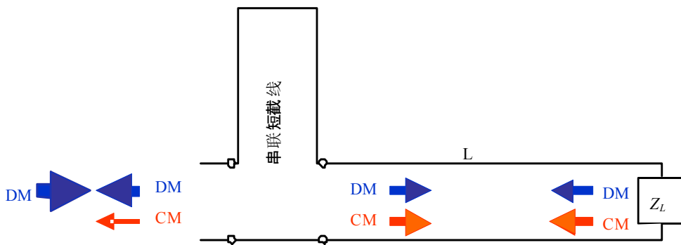
b) 开关支路的串联短截线模型
