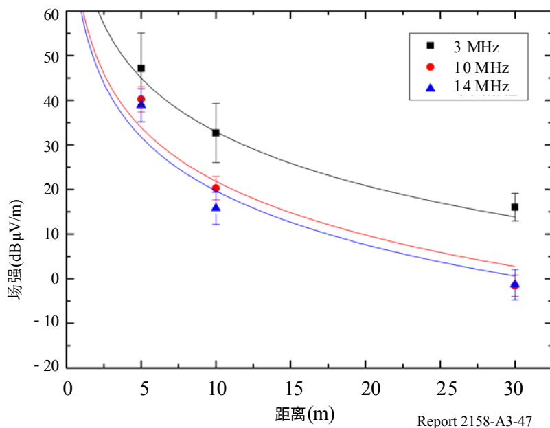
电场强度分布和模型曲线的举例
