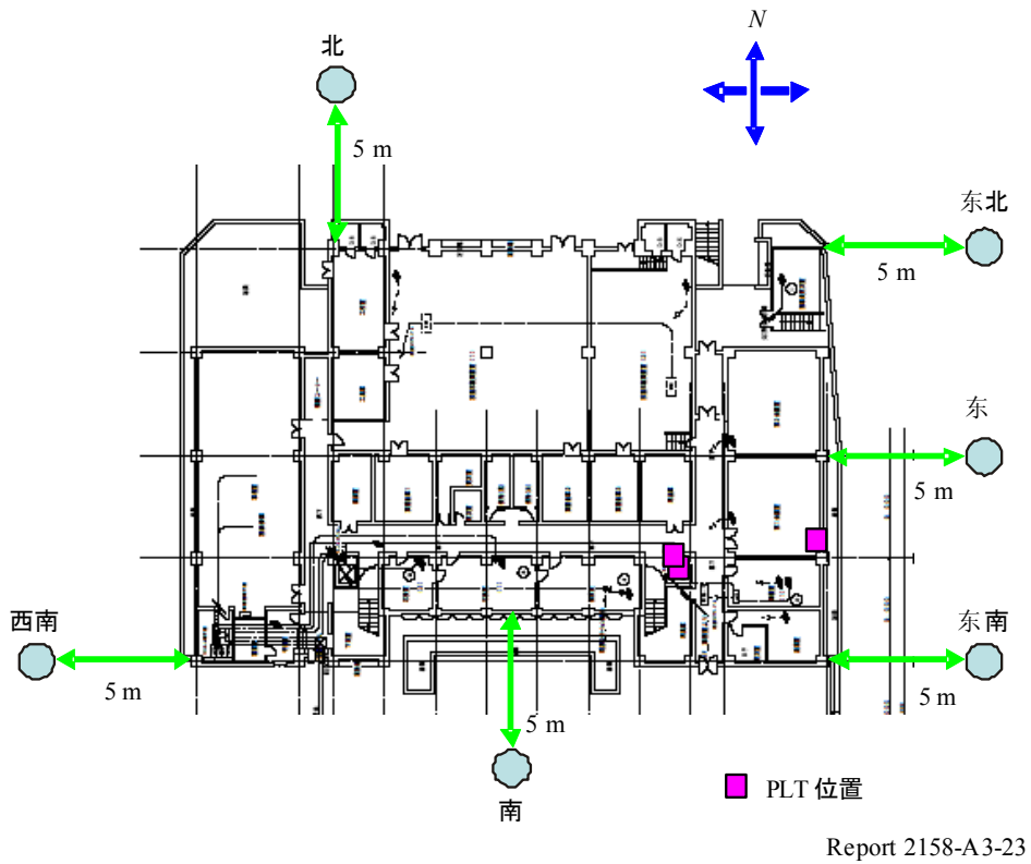
图A3-23 测量条件(2)
