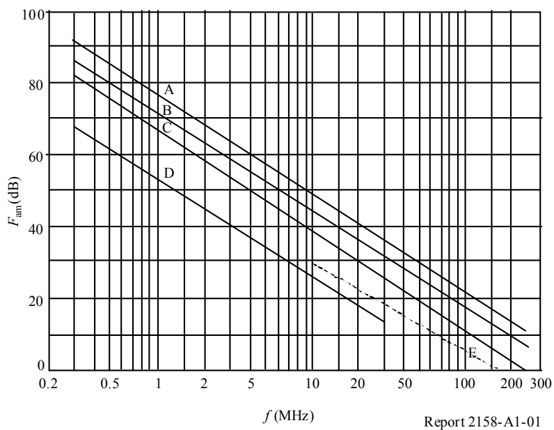
地面垂直无损单极短天线人为噪声中值 (ITU-R P.372建议书, 图10)
