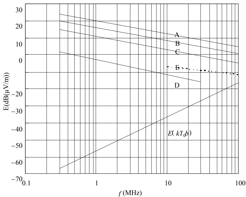
人为噪声的等效场强 ( b = 9\,000 Hz)
