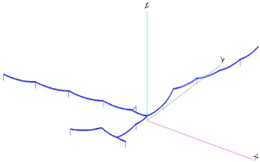
图A2-14 精细架空电力线模型的角度视图
