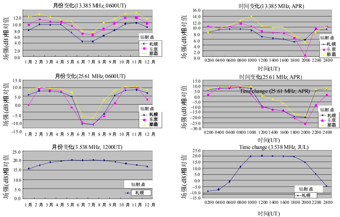
电场强度随月份/时间变化的实例
