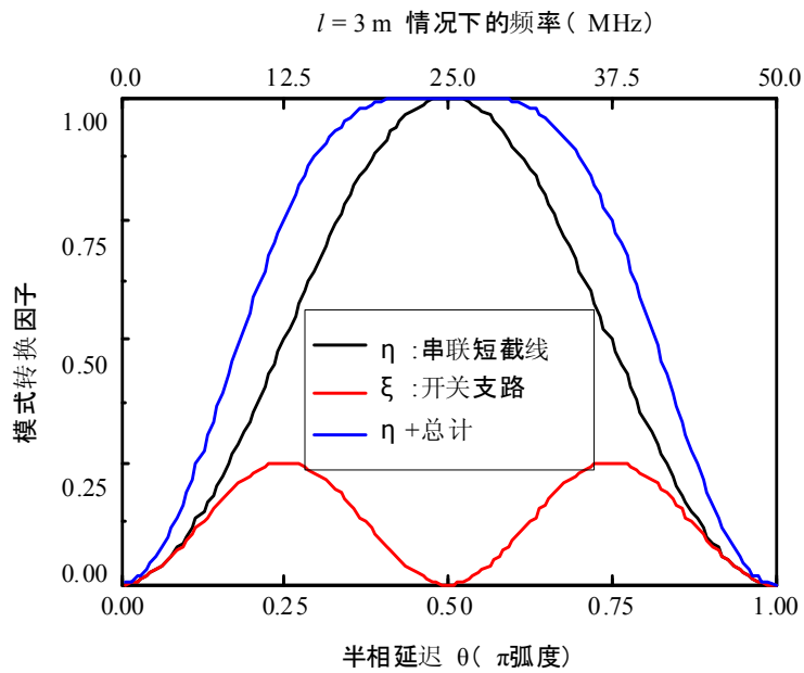
c) 串联短截线和开关支路模式转换因子
