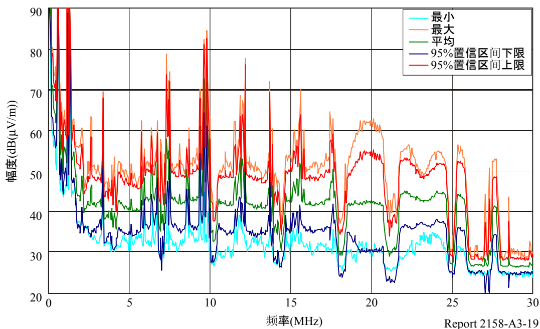
PLT设备6(UPA)在10 m处的射频场强的分布
