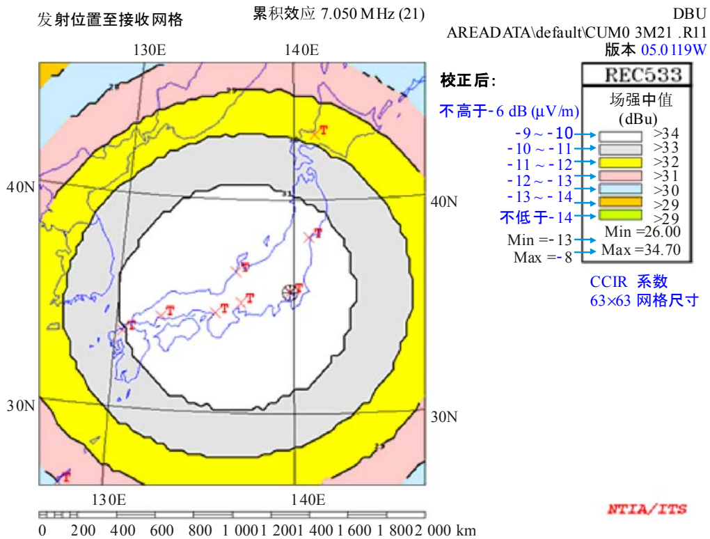
b)天波：7 MHz 频带，带宽：2.4 kHz
