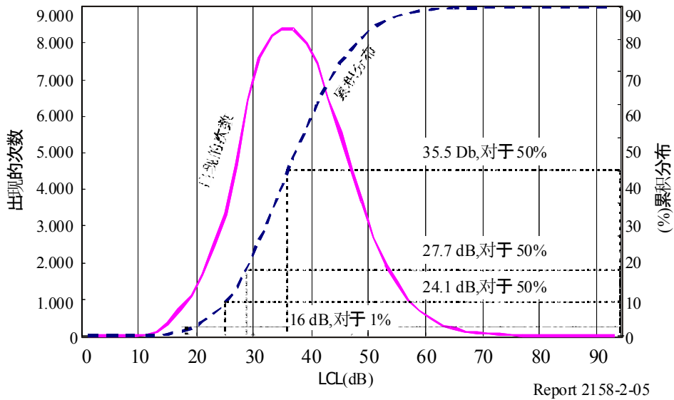
在住房墙面插座测得的LCL值
