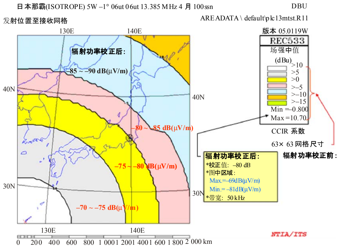
b) 13 MHz 频带, 辐射点: 那霸
