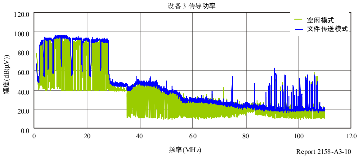
设备3(家用插座AV标准)的传导功率
