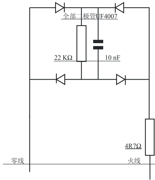
模拟小型供电装置
