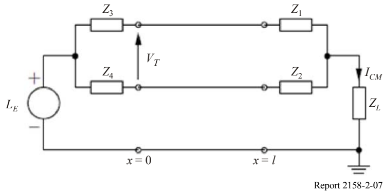
评估远端不平衡负载的LCL值的最简单模型
