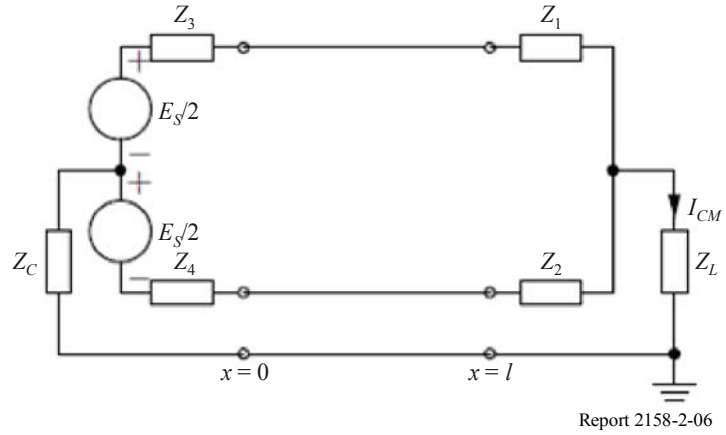
评估转换共模电流的最简单模型
