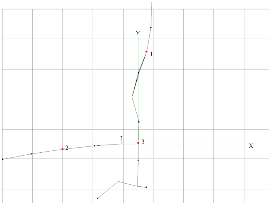
图A2-15 描述PLT输入点的电力线模型架空视图(红点)。 该分析使用输入点3. 输电变压器(阻抗负载为中性)由黑点表示。
