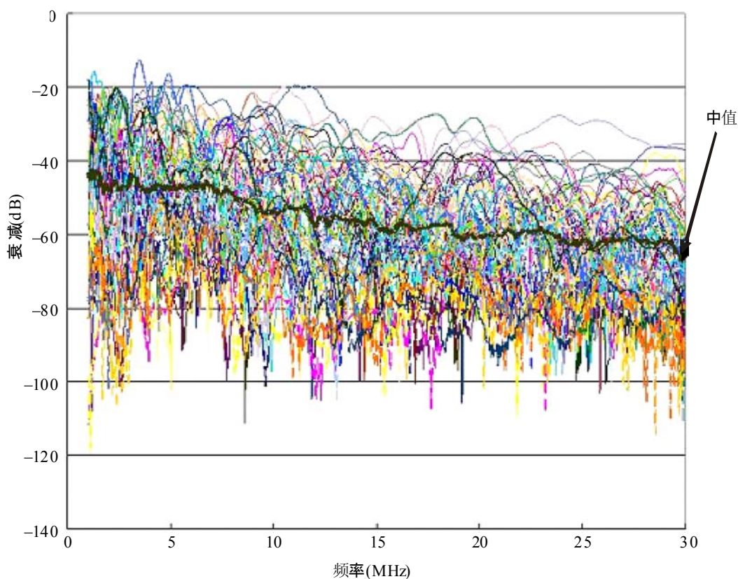
图2-10 因室内电力网设备而产生的差模电流衰减
