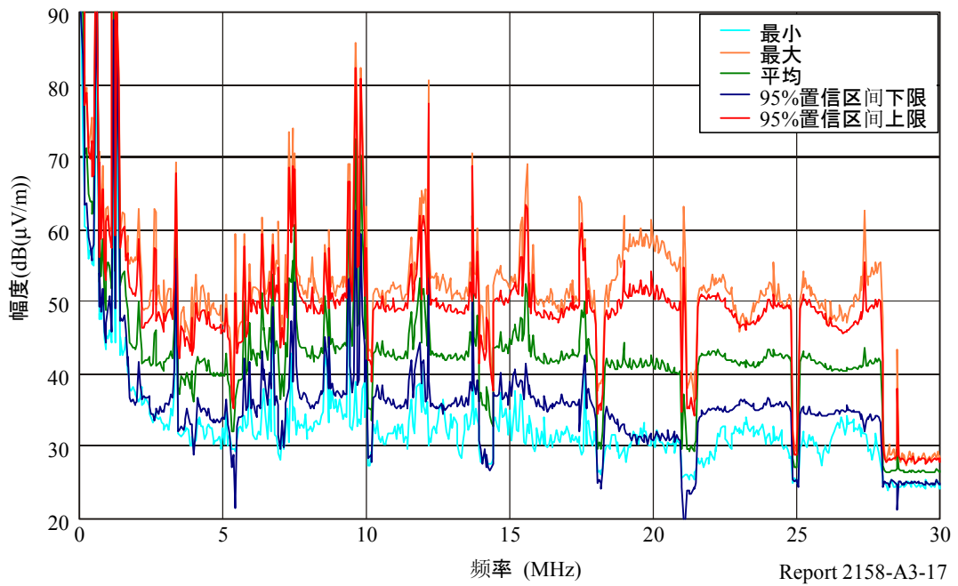
PLT设备3(家用插座AV)在10 m处的射频场强的分布
