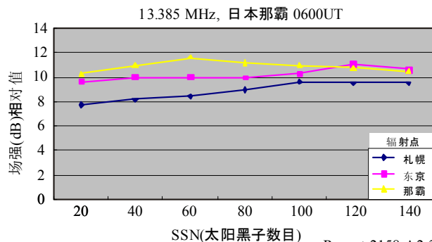
电场强度随SSN变化的实例
