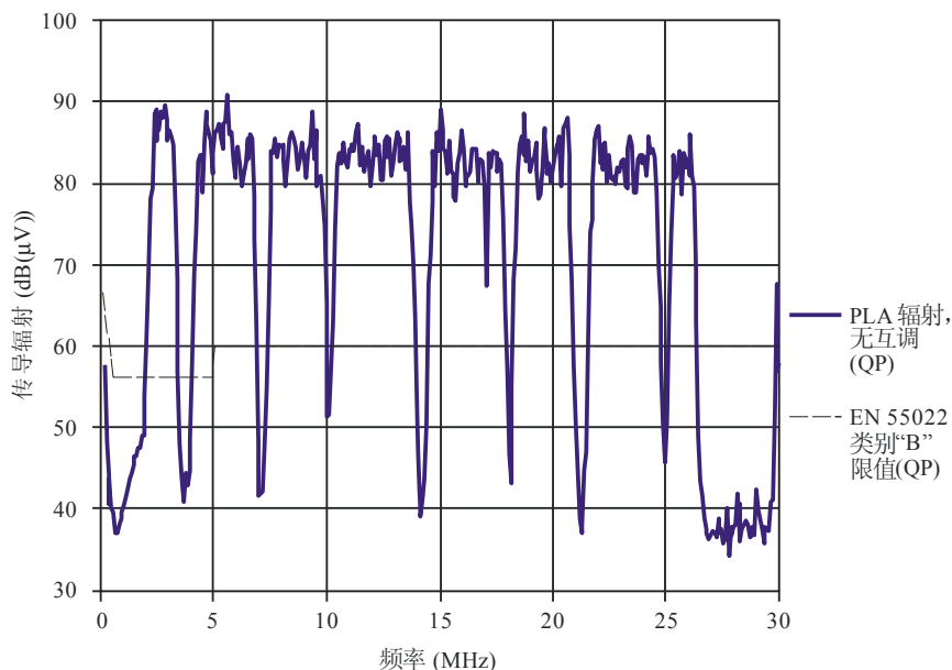
图4-6 存在陷波的频谱
