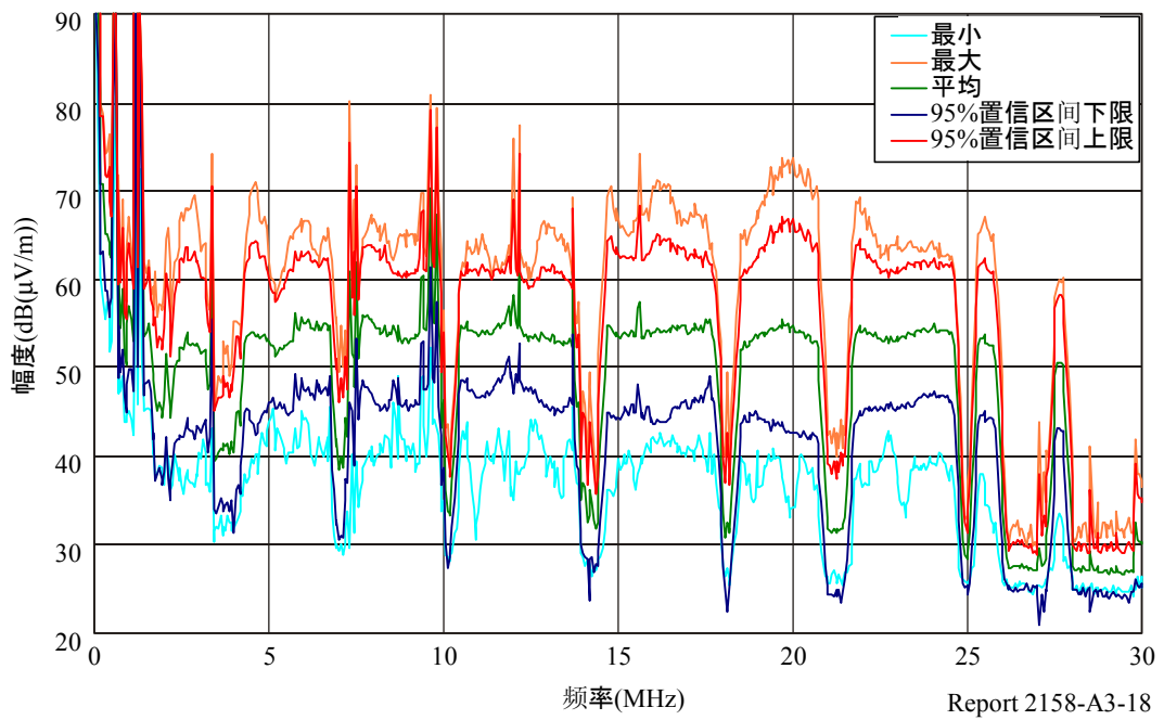
PLT设备6(UPA)在3 m处的射频场强的分布
