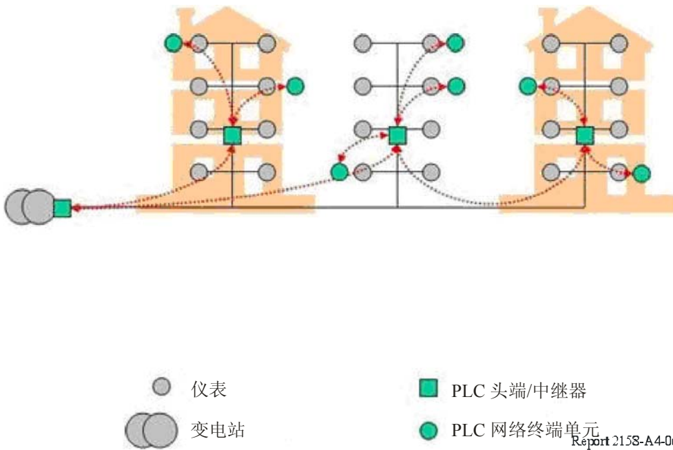
图A4-7 多层PLT网络拓扑示例
