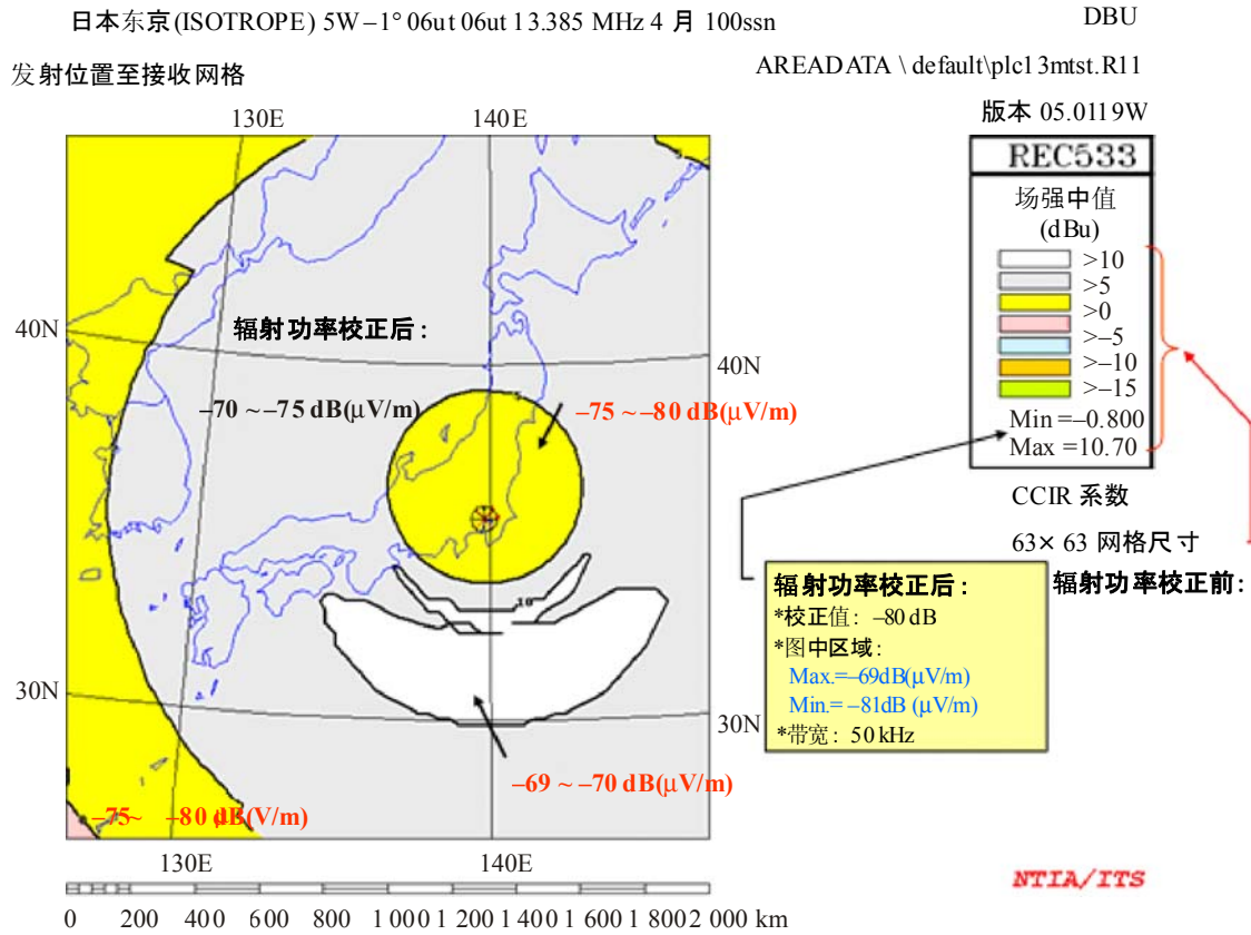
a) 13 MHz 频带, 辐射点: 东京
