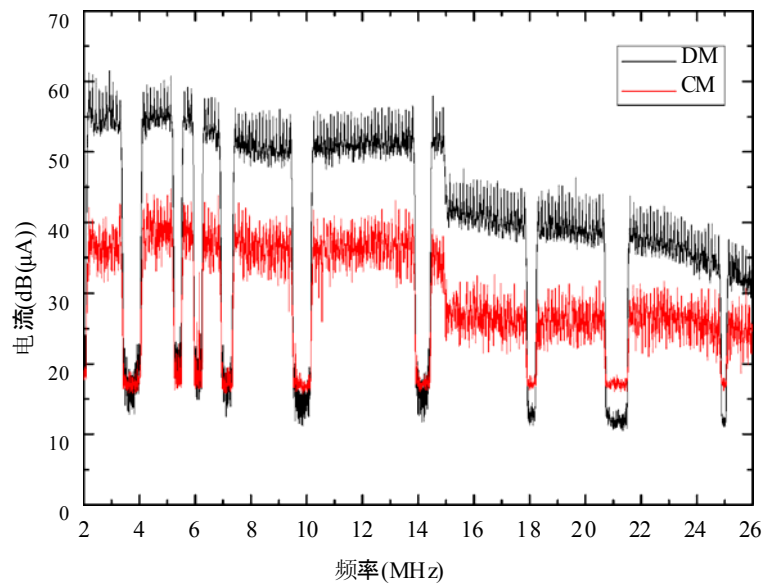
HD-PLC调制解调器(上图)和UPA调制解调器(下图) 差模(DM)电流和共模(CM)电流
