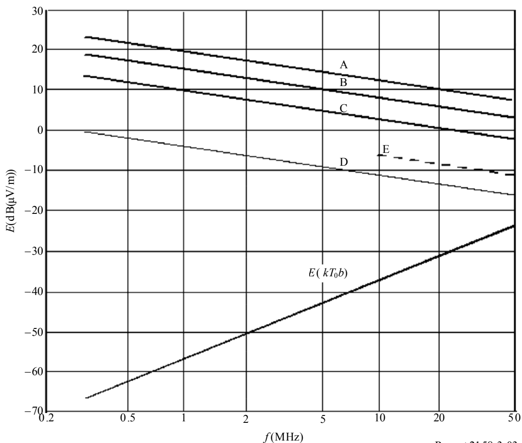
人为噪声的等效场强 (带宽 b = 6 kHz)
