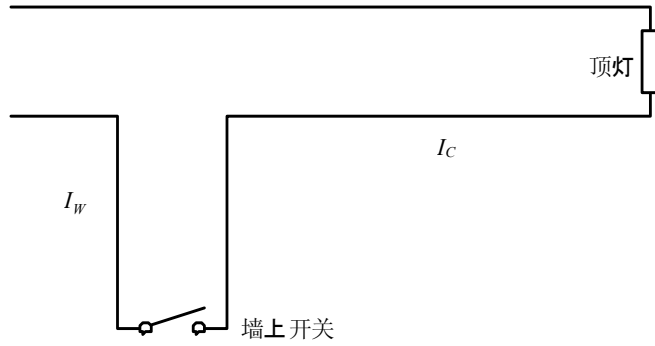
a) 由墙上单极开关和顶灯组成的开关支路
