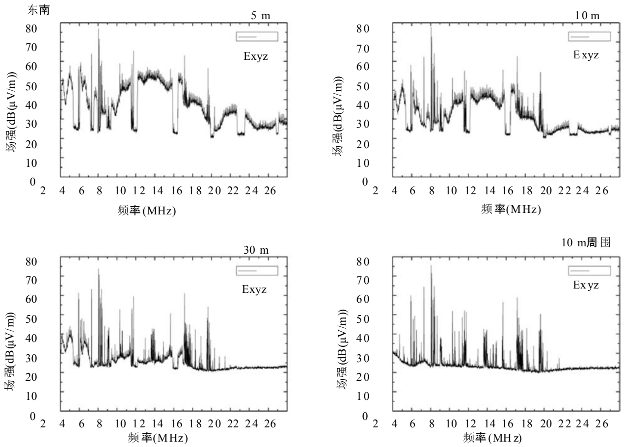
朝向东南面的HD-PLC调制解调器泄漏的场强(dB( \mu V/m))
