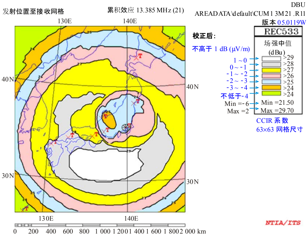
a)天波: 13 MHz 频带, 带宽: 50 kHz
