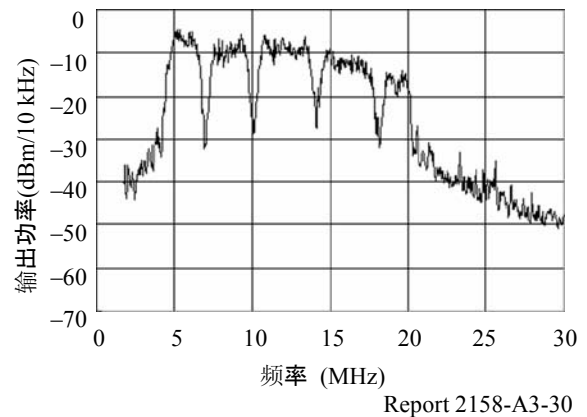
3/4号PLT调制解调器的输出功率
