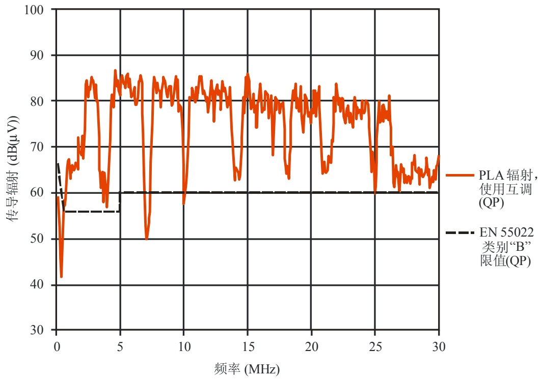
陷波的互调效果
