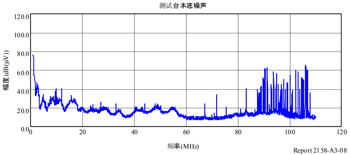
图A3-8 测试台本底噪声的测量
