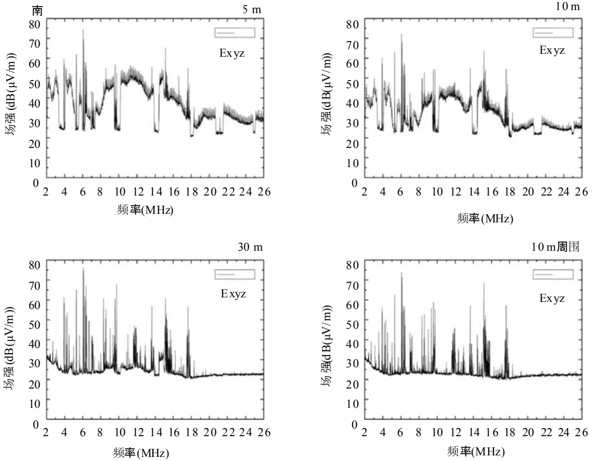
朝向南面的HD-PLC调制解调器泄漏的场强(dB( \mu V/m))
