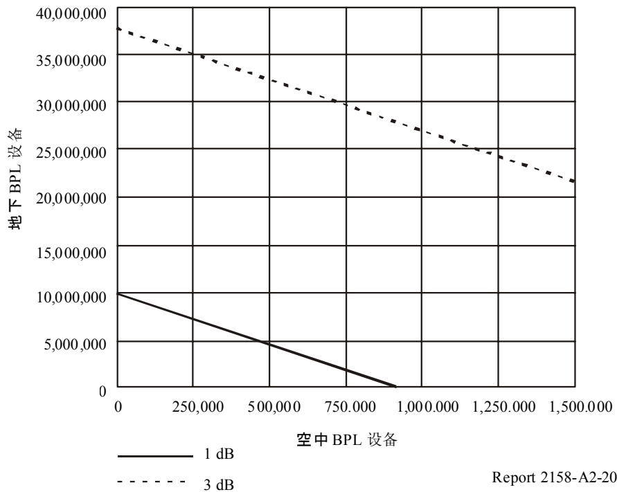
图A2-20 在低SSN条件下，能引起相同本底噪声增加的 地下PLT设备和架空PLT设备数目比较
