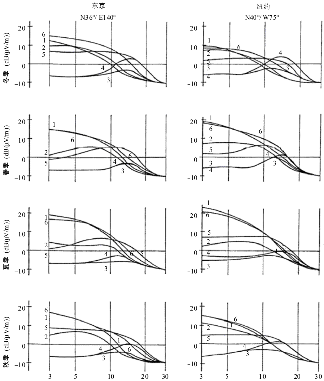
大气噪声场强示例 (东京、纽约)
