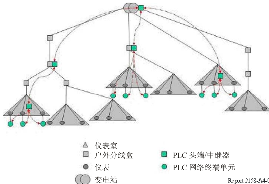
图A4-5 星型PLT网络拓扑示例
