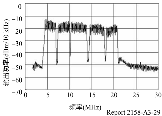
1/2号PLT调制解调器的输出功率
