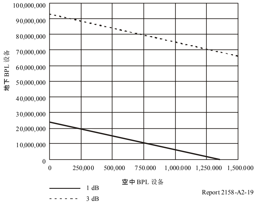
在高SSN条件下，能引起相同本底噪声增加的 地下PLT设备和架空PLT设备数目比较
