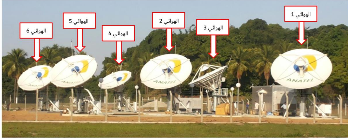
هوائيات في النطاقين C و Ku بالمحطة EMSAT، ريو دي جانيرو
