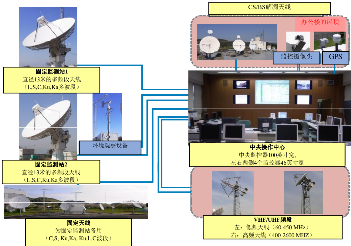
图9 空间无线电监测设备的配置
