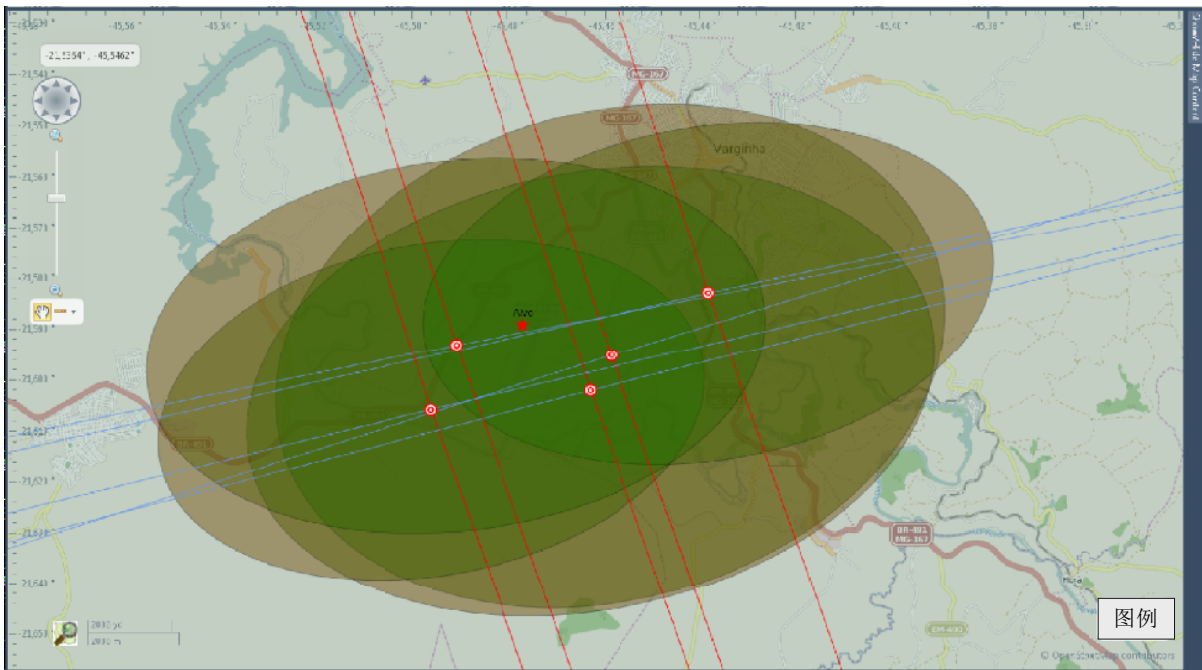
图25 地理定位输出结果（地理定位椭圆重复五次并收敛到同一区域）
