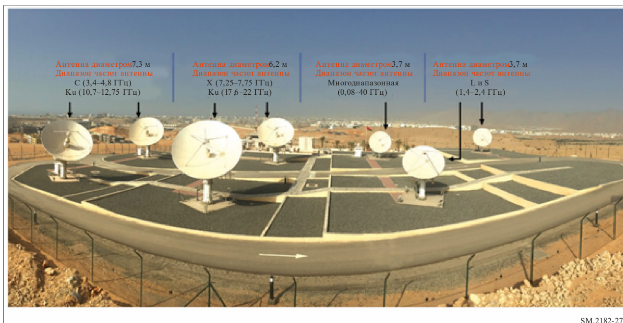
Антенная система SRMS
