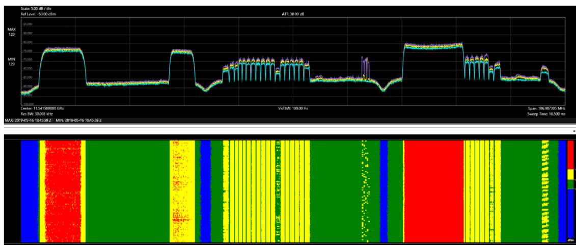
Спектрограмма сигналов, принятых от ретрансляторов
