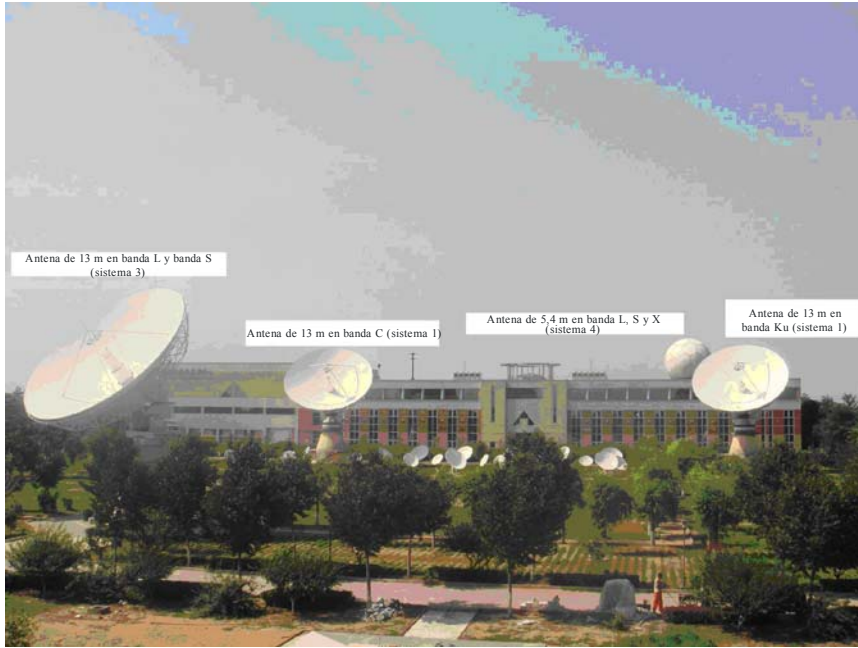
FIGURA 2 Antenas de los sistemas 1, 3 y 4
