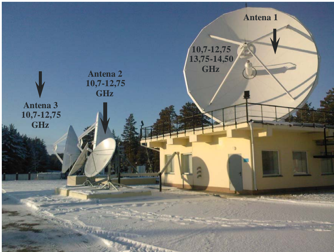
Panorámica general de los sistemas de antena números 1, 2 y 3
