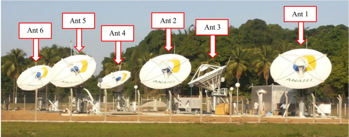
C and Ku antennas at EMSAT, Rio de Janeiro
