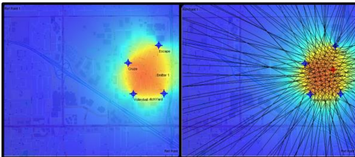
FIGURE 14 GDOP à Santa Clara et affichage des hyperboles TDOA
