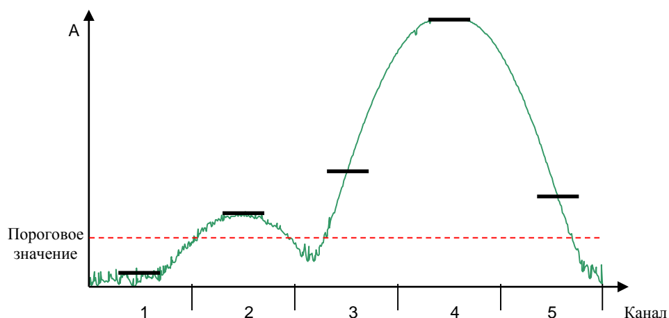
Полоса измерения установлена слишком широкой
