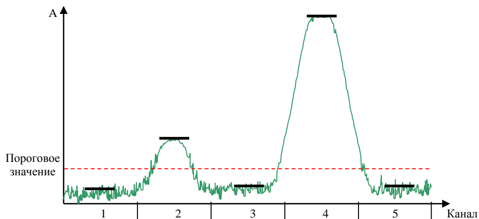
Правильная установка ширины полосы измерений
