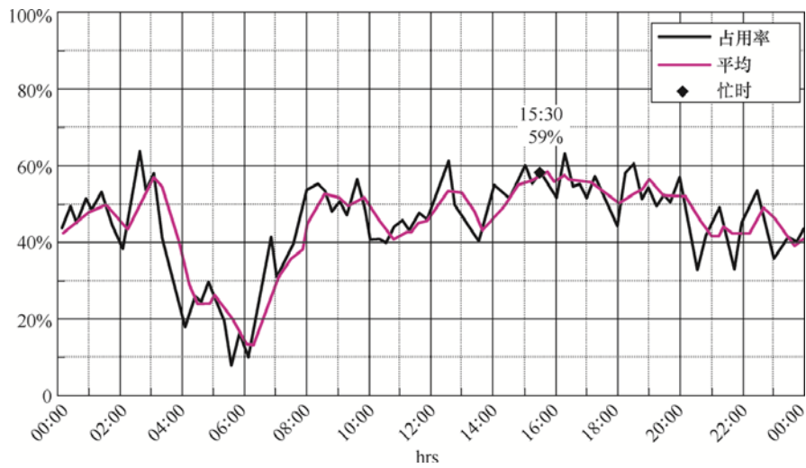
图15 一个频道上的业务量图
