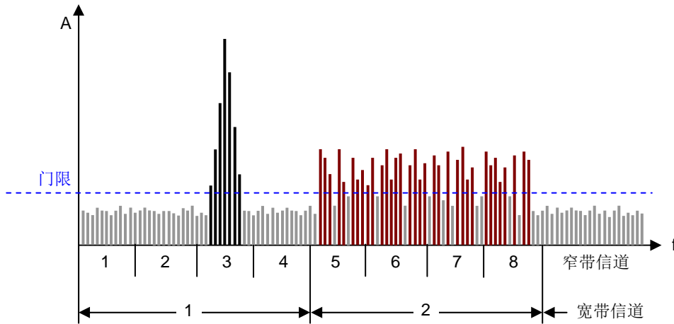
图14 评估具有不同信道宽度的频段内的测量样本
