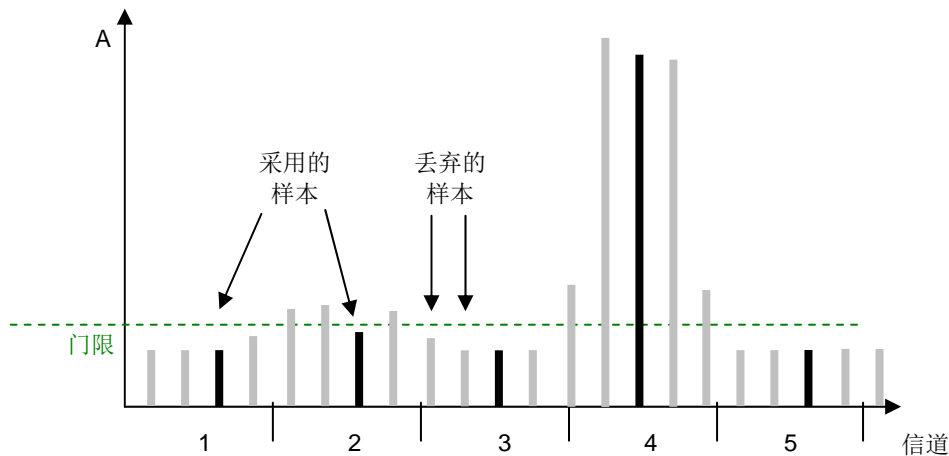
图12 合并测量样本的简单方法
