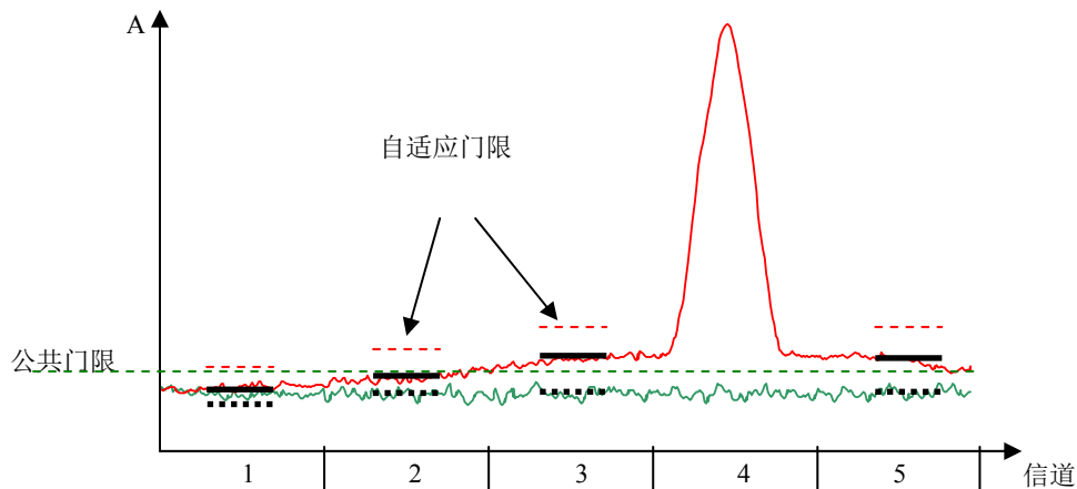
图 5 噪声电平和自适应门限
