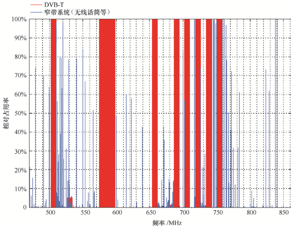
图 16 具有不同宽度的多个信道的占用率举例
