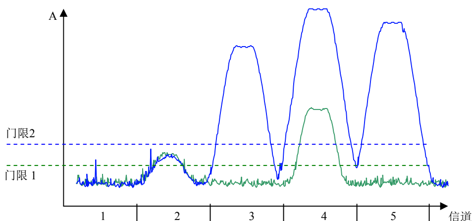
图6 门限和占用率的相关性
