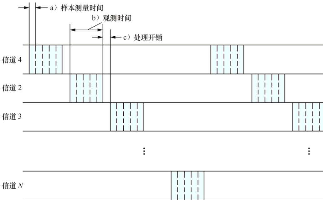
图 8 针对短持续时间信号的时间安排优化
