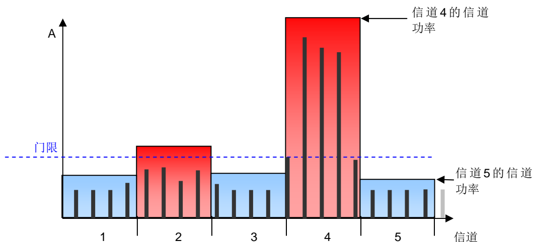
图13 通过信道功率计算的测量样本合并
