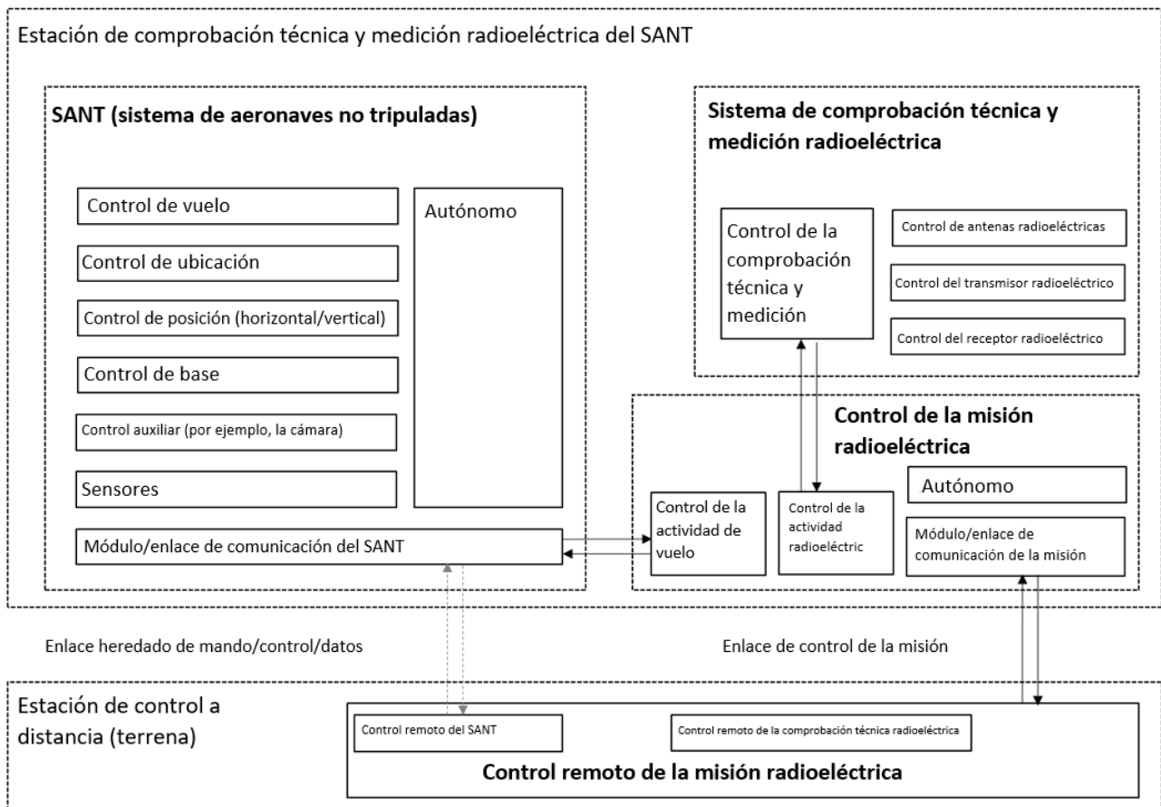
FIGURA 1 Arquitectura funcional de una estación de comprobación técnica y medición radioeléctrica basada en drones
