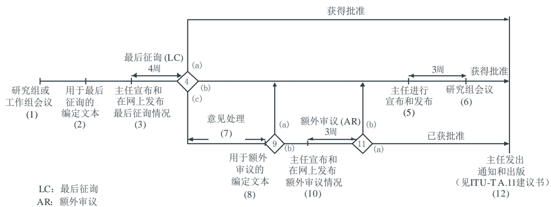
图1 – 流程
