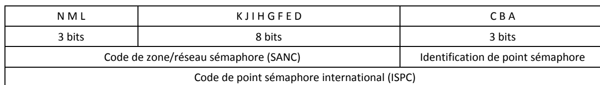
Figure 7 – Structure du code de point sémaphore international
