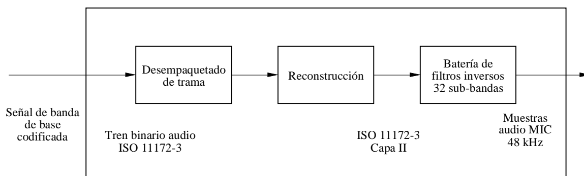
FIGURA 3 Diagrama de bloques del decodificador audio básico del Sistema
