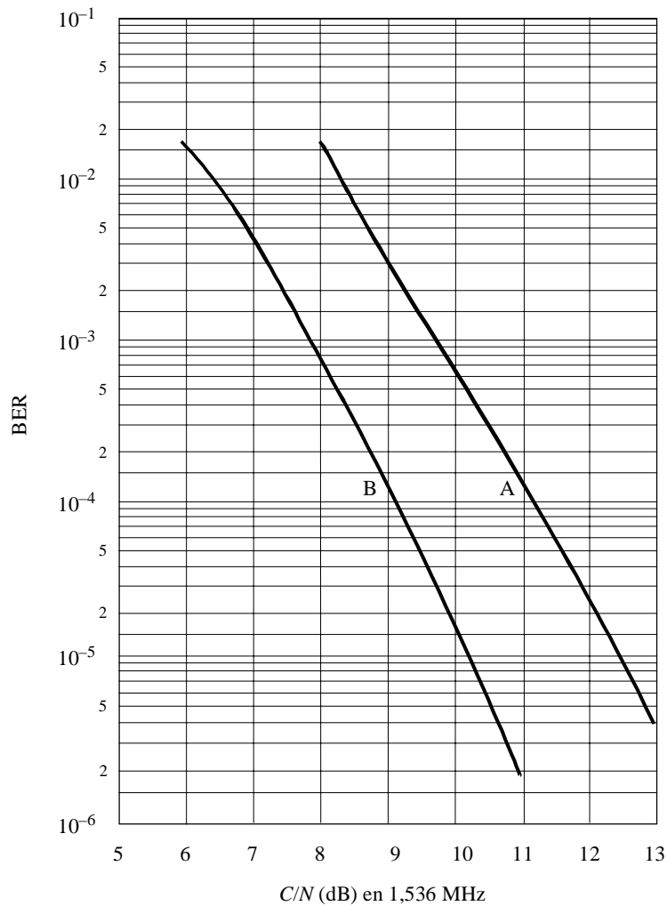
FIGURA 9 BER en función de C/N (en 1,5 MHz) en un canal Rayleigh, 1 500 MHz, Modo II
