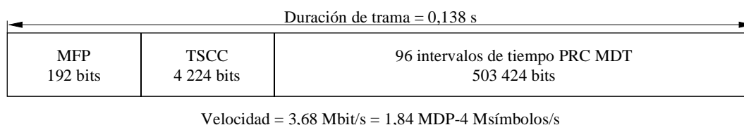
FIGURA 23 Trama MDT de enlace descendente
