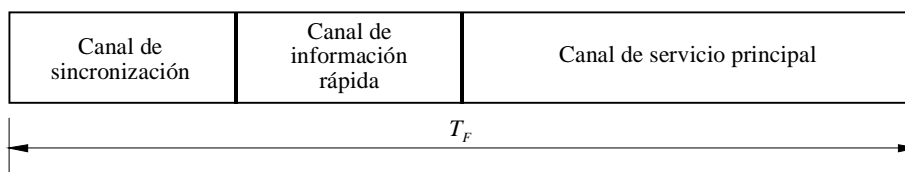
FIGURA 4 Estructura de la trama múltiplex
