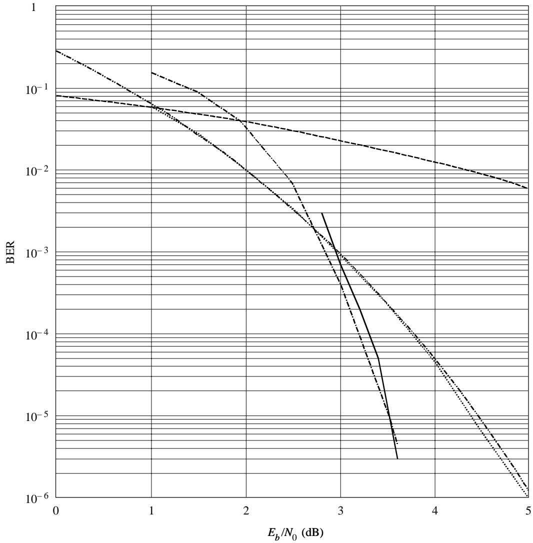
FIGURA 12 Calidad de funcionamiento del Sistema B en un canal AWGN
