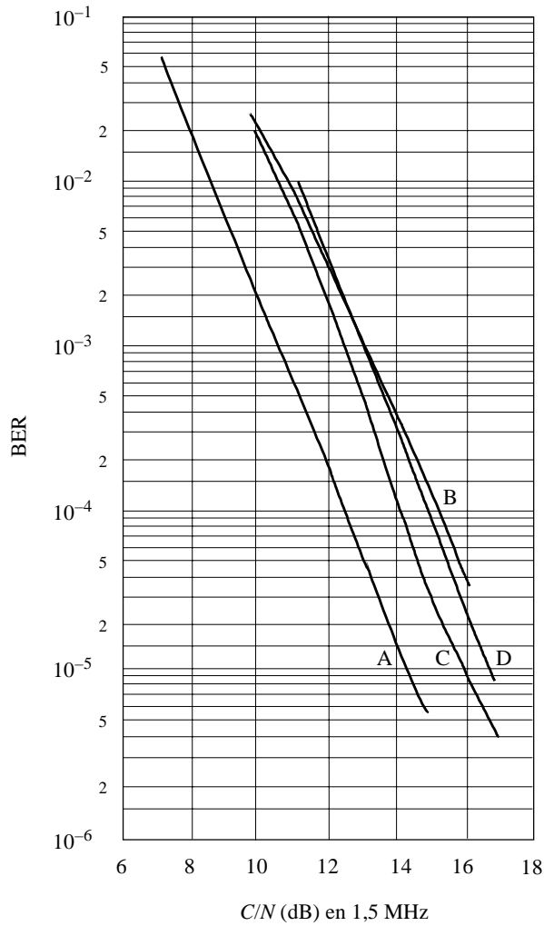
FIGURA 8 BER en función de C/N (en 1,5 MHz) en un canal de Rayleigh 226 MHz, Modo I
