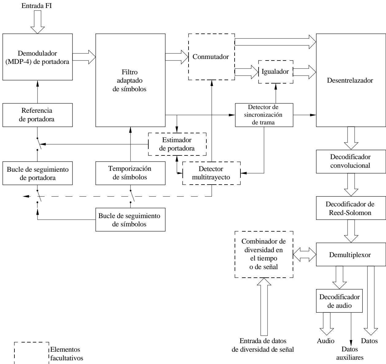
Diagrama de bloques funcionales del receptor
