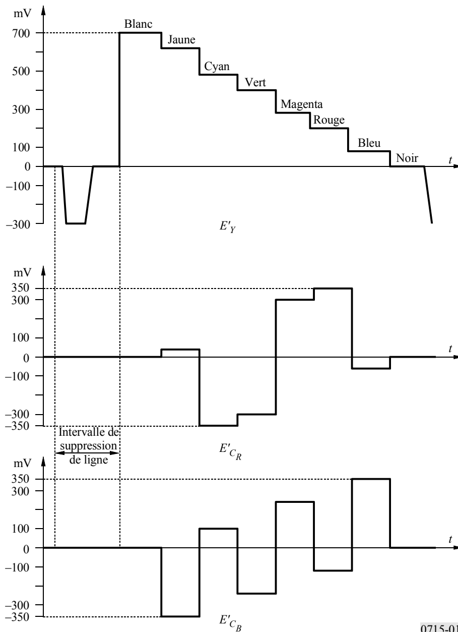
Forme d'onde des signaux vidéo pour les barres de couleur 100/0/100/0
