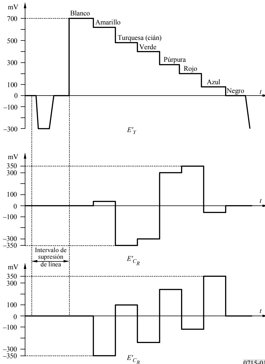
Forma de onda de las señales vídeo para las barras de color 100/0/100/0
