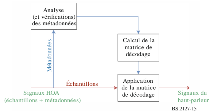
Diagramme du flux de restitution HOA
