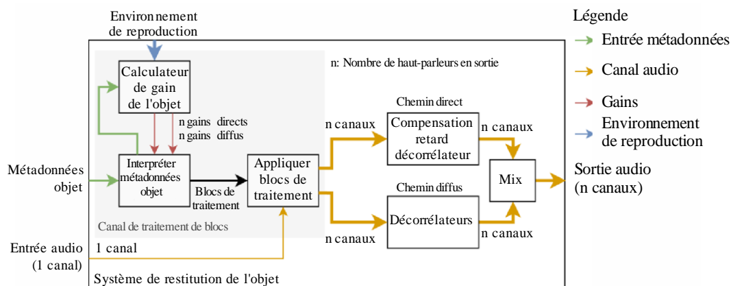
Structure du système de restitution des objets
