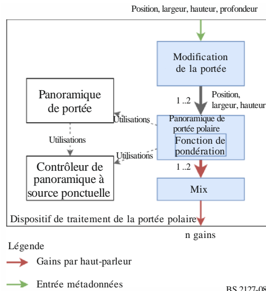
FIGURE 8 Structure du gestionnaire de portée
