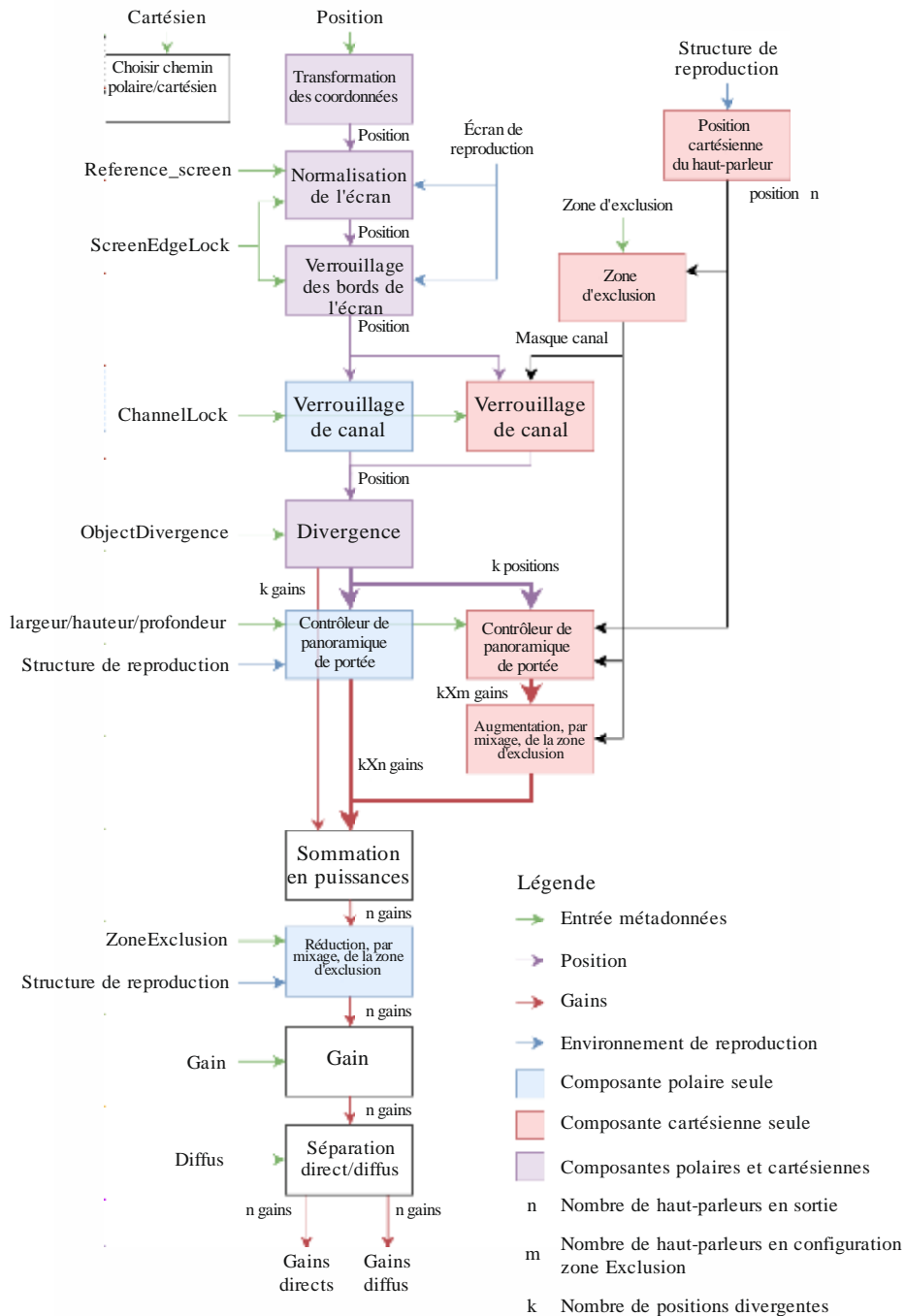
FIGURE 7 Structure du calculateur de gain pour le composant typeDefinition==Objects
