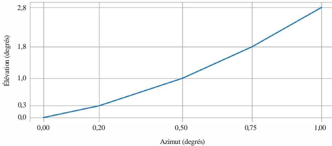
FIGURE 14 Mise en correspondance linéaire par morceaux entre les paramètres de la portée de l'ADM et les valeurs de l'algorithme de la portée interne.
