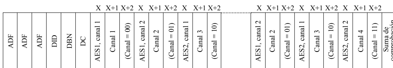
FIGURA 2 Estructura del paquete de datos de audio (Ejemplo de 4 canales de audio, 1 grupo de audio)
