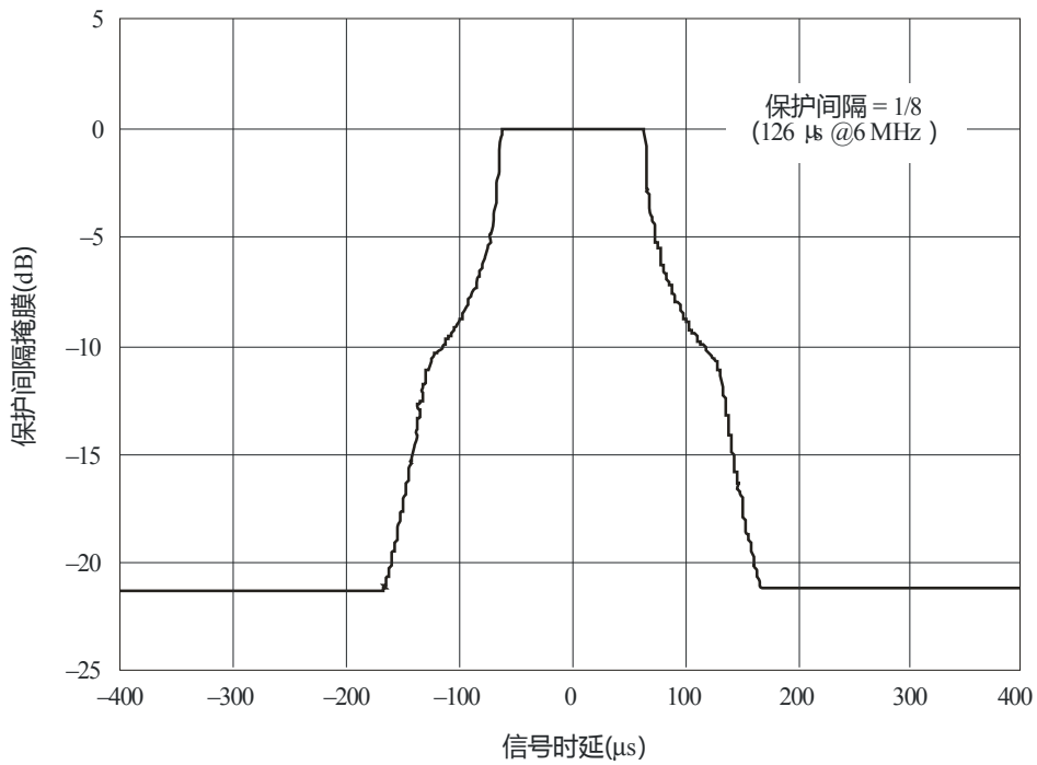
6 MHz的保护间隔掩膜特性 (@GI = 1/8, 64-QAM-FEC 3/4) 12
