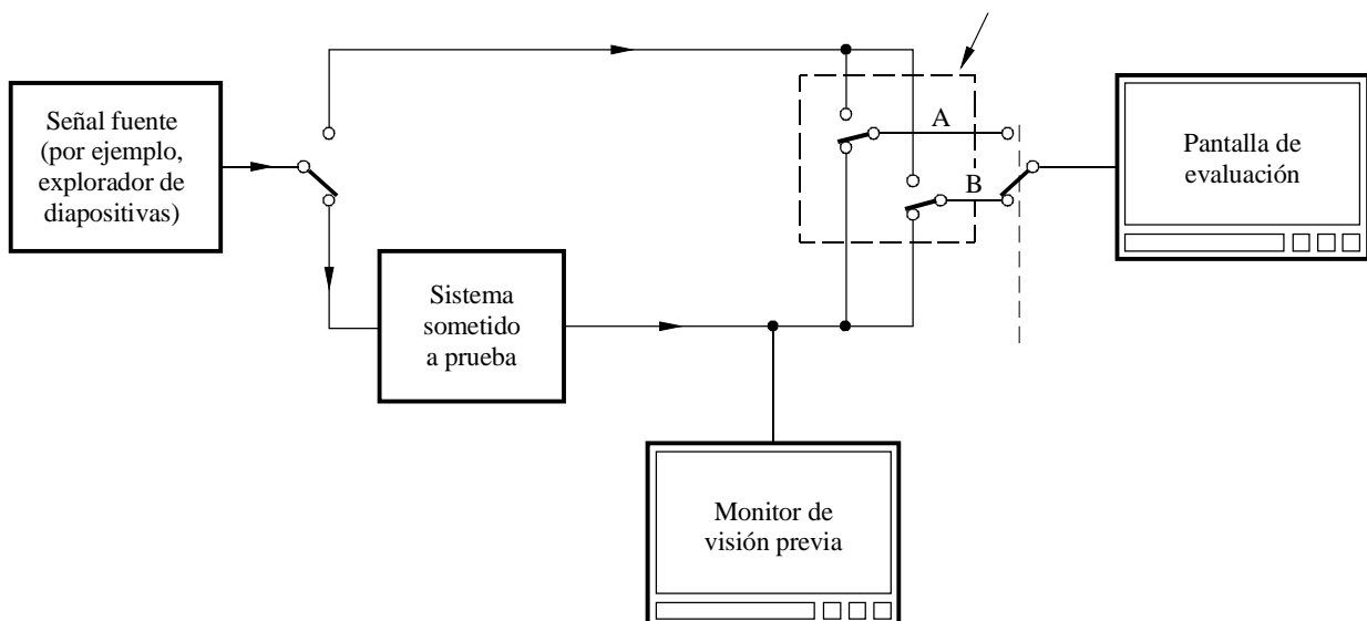
Disposición general del sistema de prueba para el método de doble estímulo con escala de calidad continua
