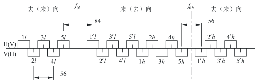
图 4 7 GHz 频段射频信道安排 （所有频率单位为 MHz）
