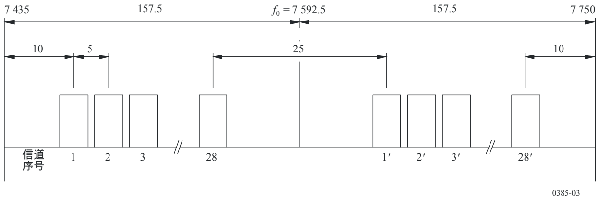
图 3 工作于 7 GHz 频段的数字系统的射频信道安排 (所有频率单位为 MHz)
