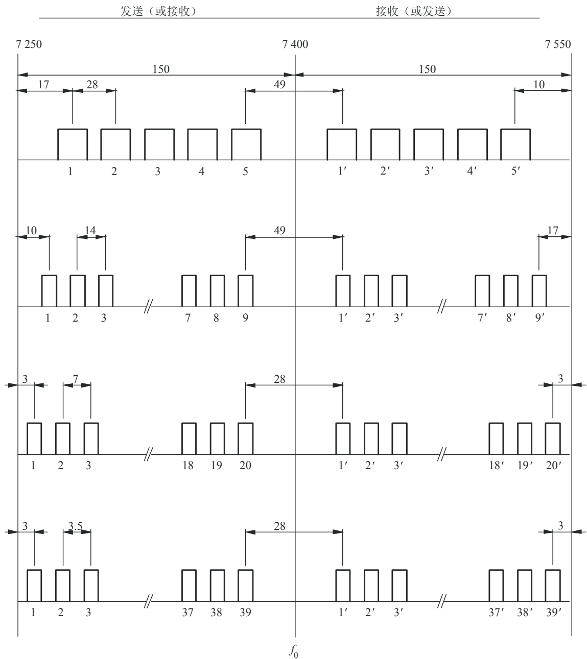
图6 工作于 7 GHz 频段的且信道间隔为 28、14、7 和 3.5 MHz 的数字无线系统的射频信道安排 (所有频率单位为 MHz)
