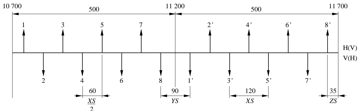
FIGURE 6 Disposition des canaux radioélectriques pour un faisceau hertzien à 140 Mbit/s fonctionnant dans la bande 10,7-11,7 GHz (Fréquences en MHz)
