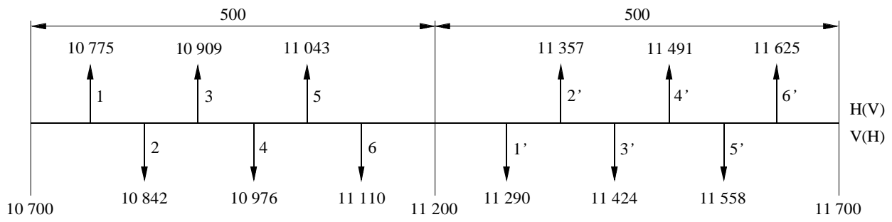
FIGURE 5 Disposition des canaux radioélectriques pour des faisceaux hertziens numériques MDP-4 (Fréquences en MHz)
