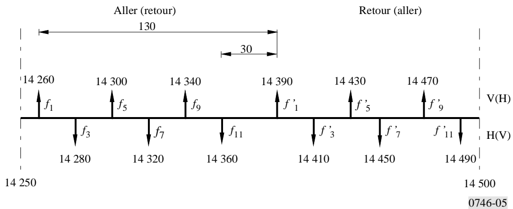
Disposition des canaux radioélectriques pour des faisceaux hertziens fonctionnant dans la bande des 14 GHz avec un espacement de 20 MHz (Fréquences en MHz)
