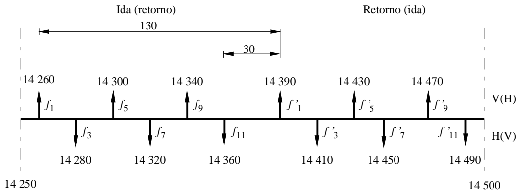
FIGURA 5 Disposición de radiocanales para los sistemas de radioenlaces que funcionan en la banda de 14 GHz con una separación de 20 MHz (Todas las frecuencias en MHz)
