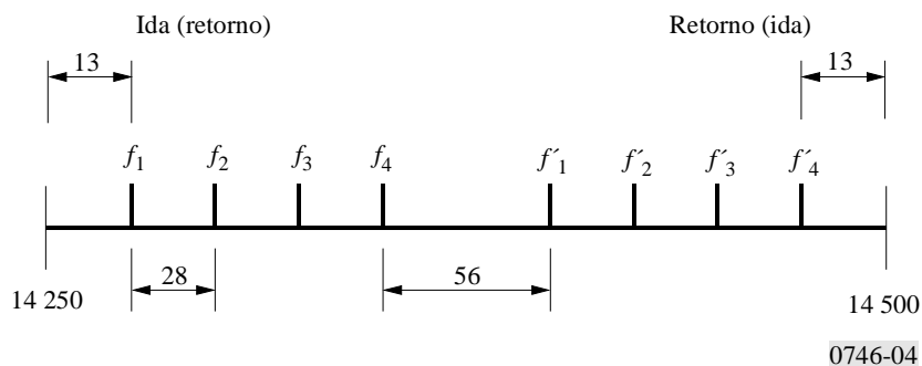
FIGURA 4 Disposición de radiocanales en la banda de frecuencias 14,25-14,5 GHz (Todas las frecuencias en MHz)
