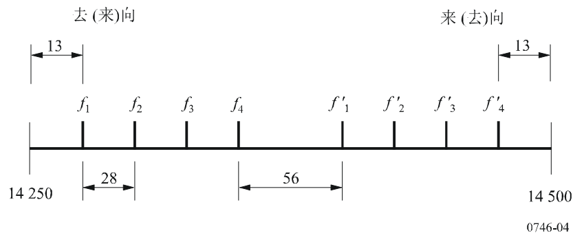
图 4 14.25-14.5 GHz频段的射频信道配置 (所有频率单位为MHz)
