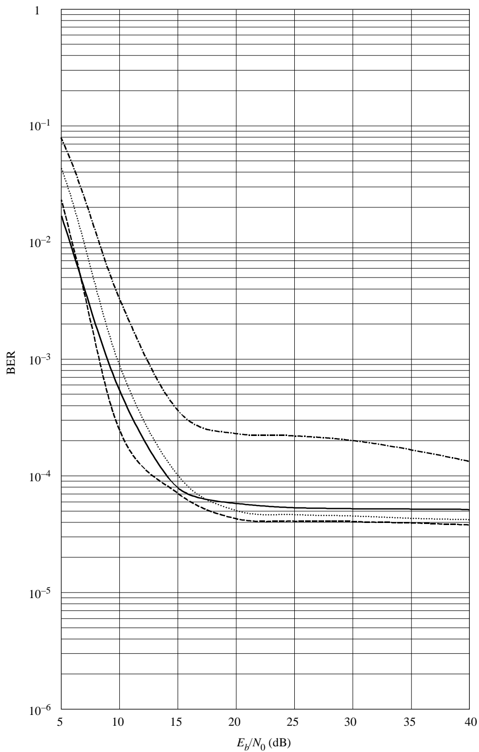
FIGURA 18 BER de MDP-4 en función de la densidad espectral de ruido para un canal con desvanecimiento
