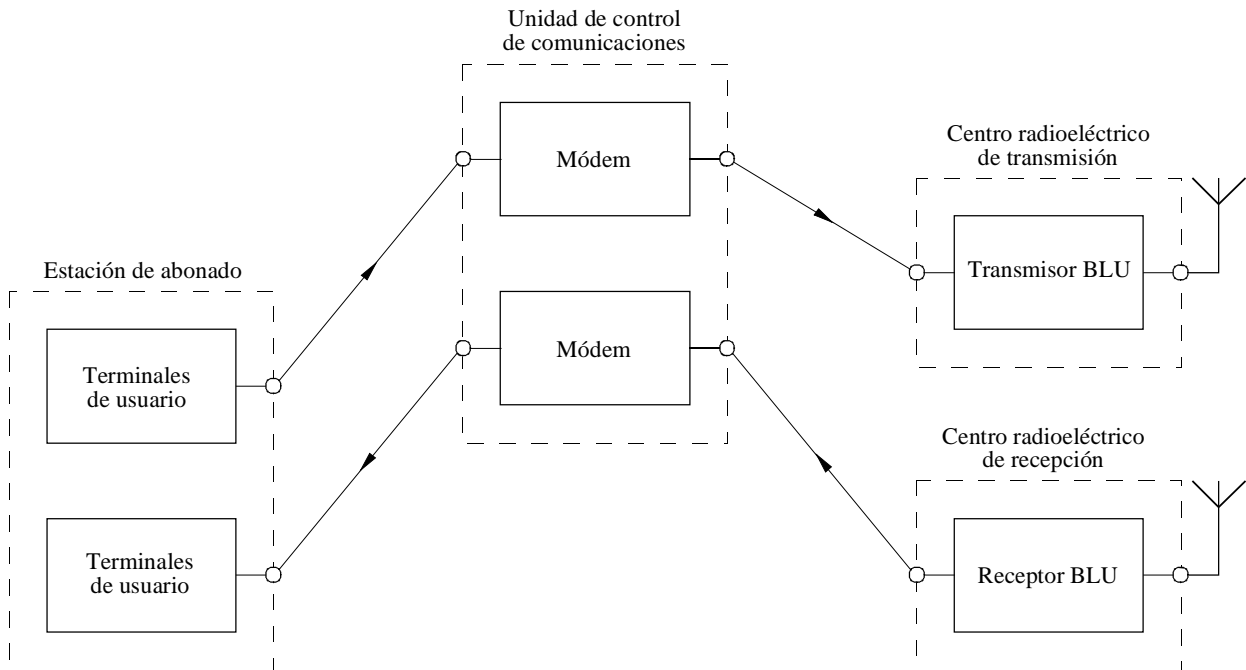
FIGURA 9 Diagrama de bloques del sistema
