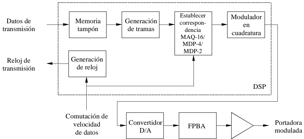
FIGURA 13a Diagrama de bloques del modulador
