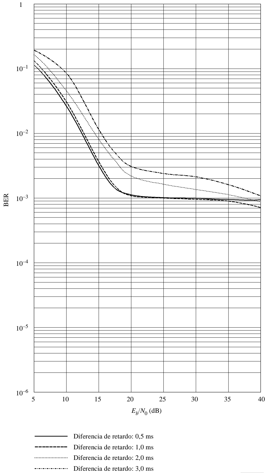
FIGURA 17 BER de MAQ-16 en función de la densidad espectral de ruido para un canal con desvanecimiento
