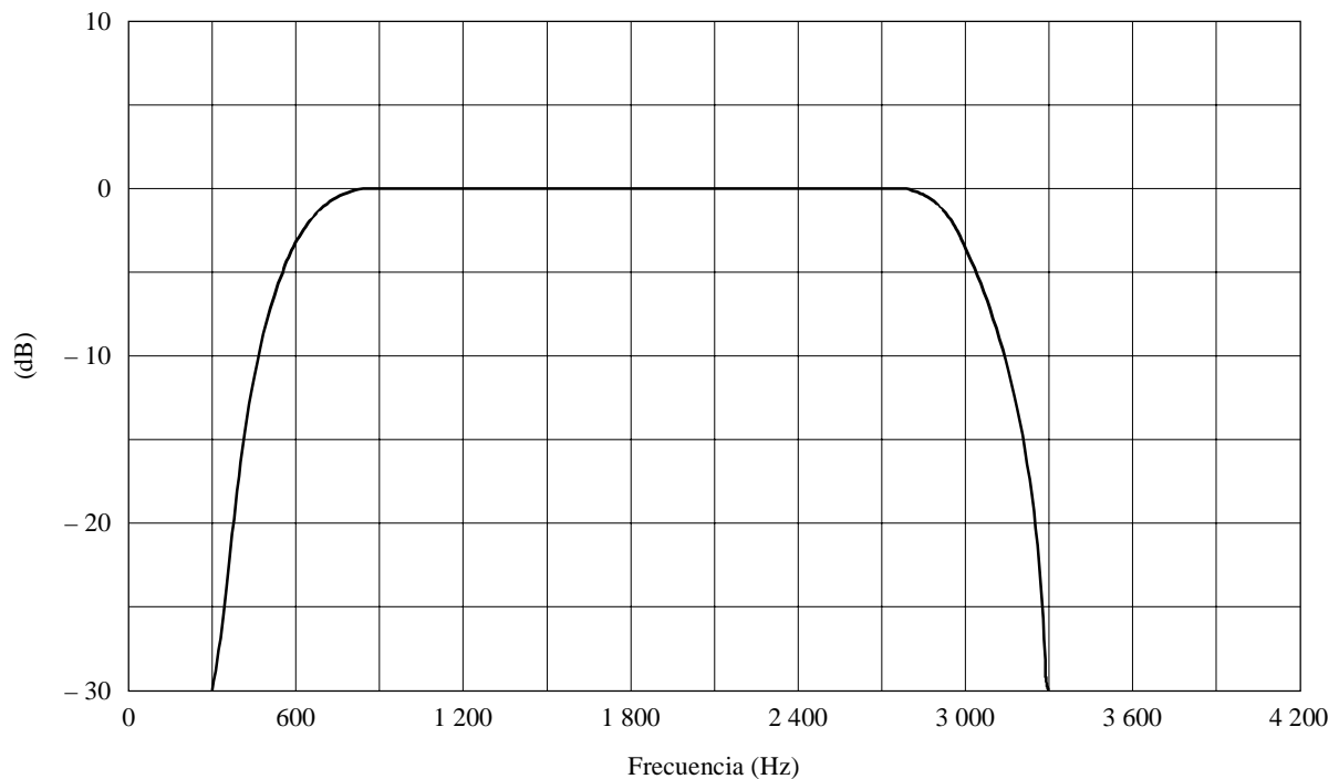
FIGURA 7 Espectro de la señal modulada
