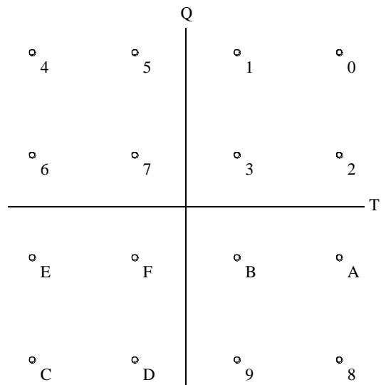
FIGURA 15 Diagrama de constelación de MAQ-16
