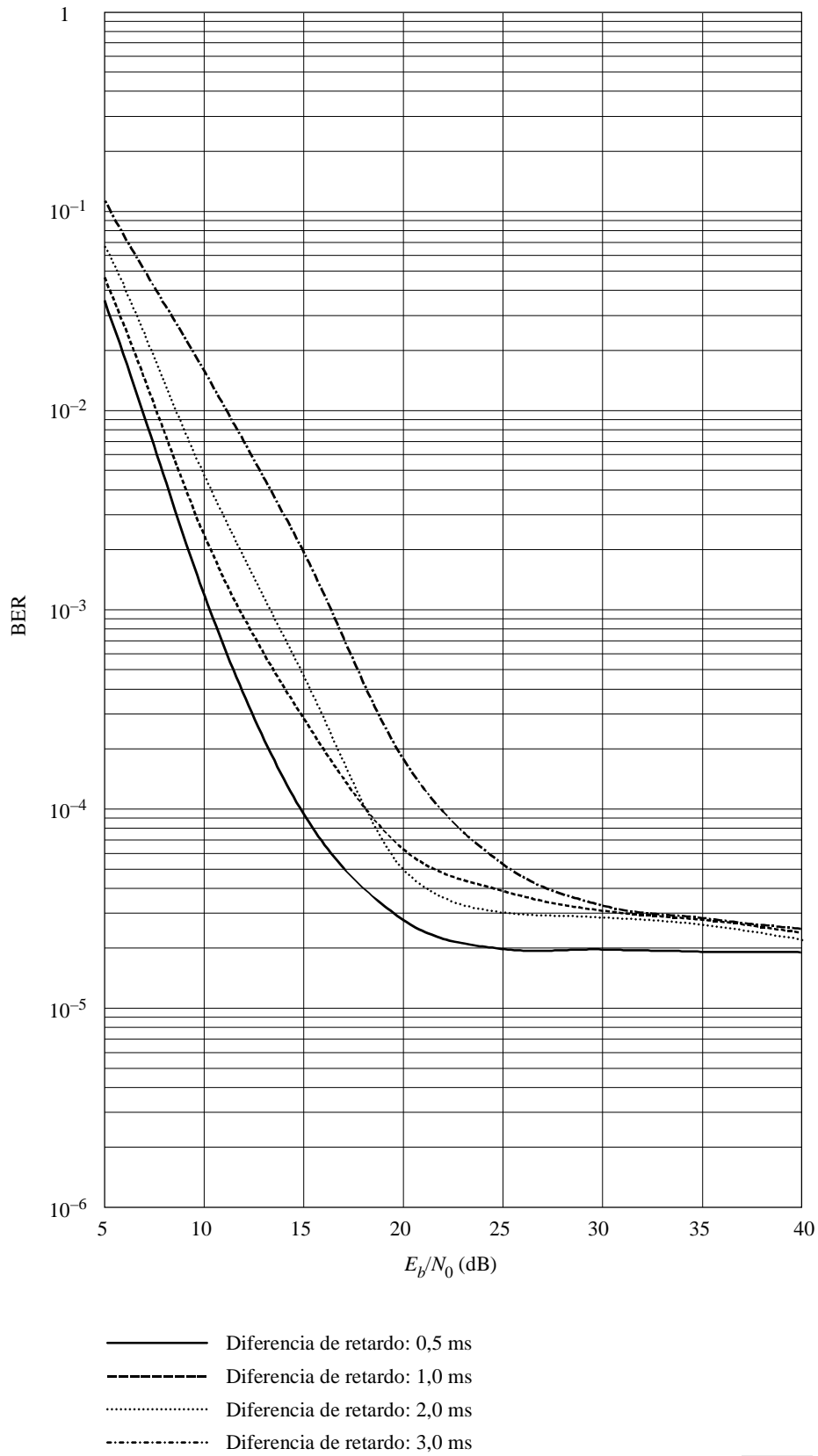
FIGURA 19 BER de MDP-2 en función de la densidad espectral de ruido para un canal con desvanecimiento
