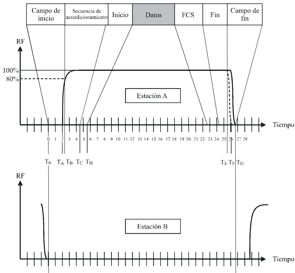
Temporización de la transmisión
