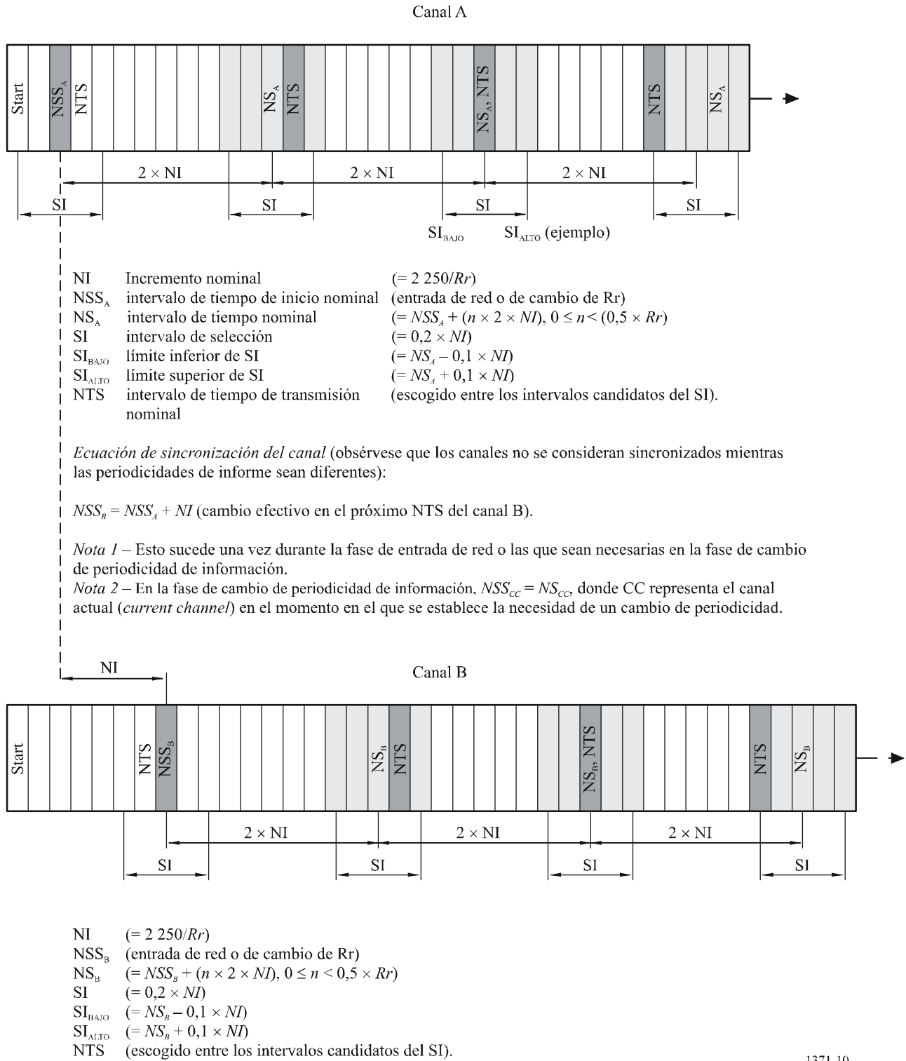
FIGURA 10 Periodicidad de información uniforme utilizando dos canales
