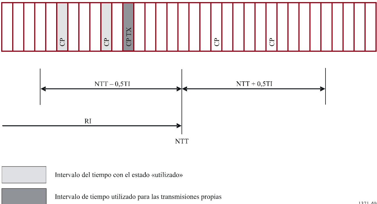
FIGURA 40 Ejemplo de acceso AMDT-CS
