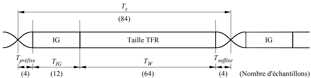
Format des symboles MROF
