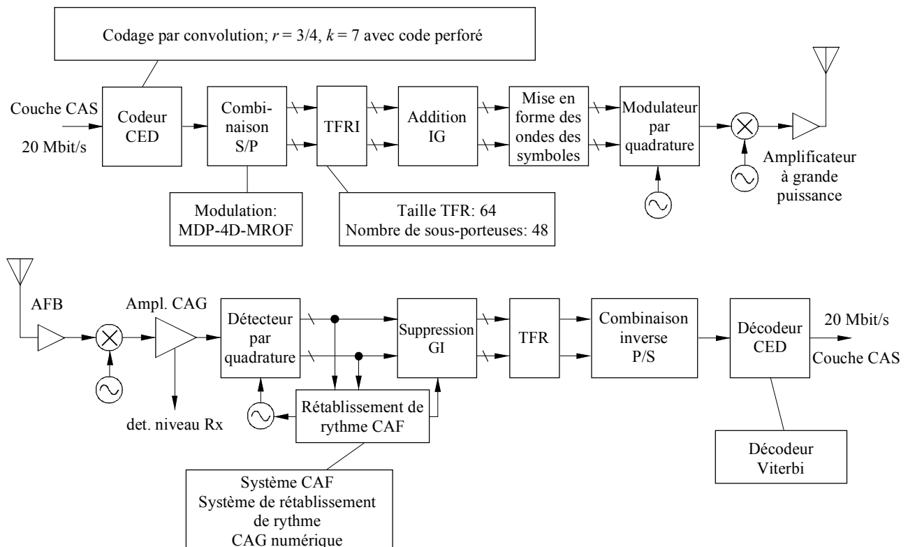
Configuration du système MDP-4D-MROF avec codage par convolution
