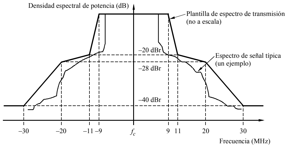
FIGURA 1 Plantilla de espectro de transmisión
