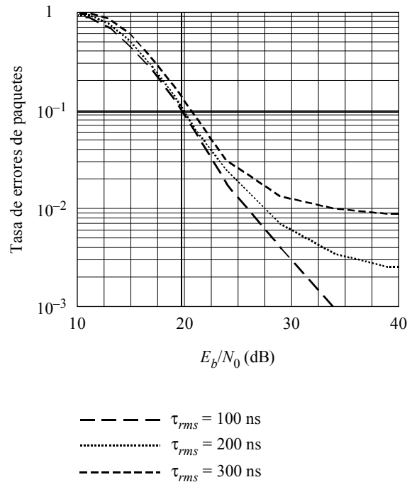
FIGURA 5 Tasa de errores de paquetes en función de E_b/N_0
