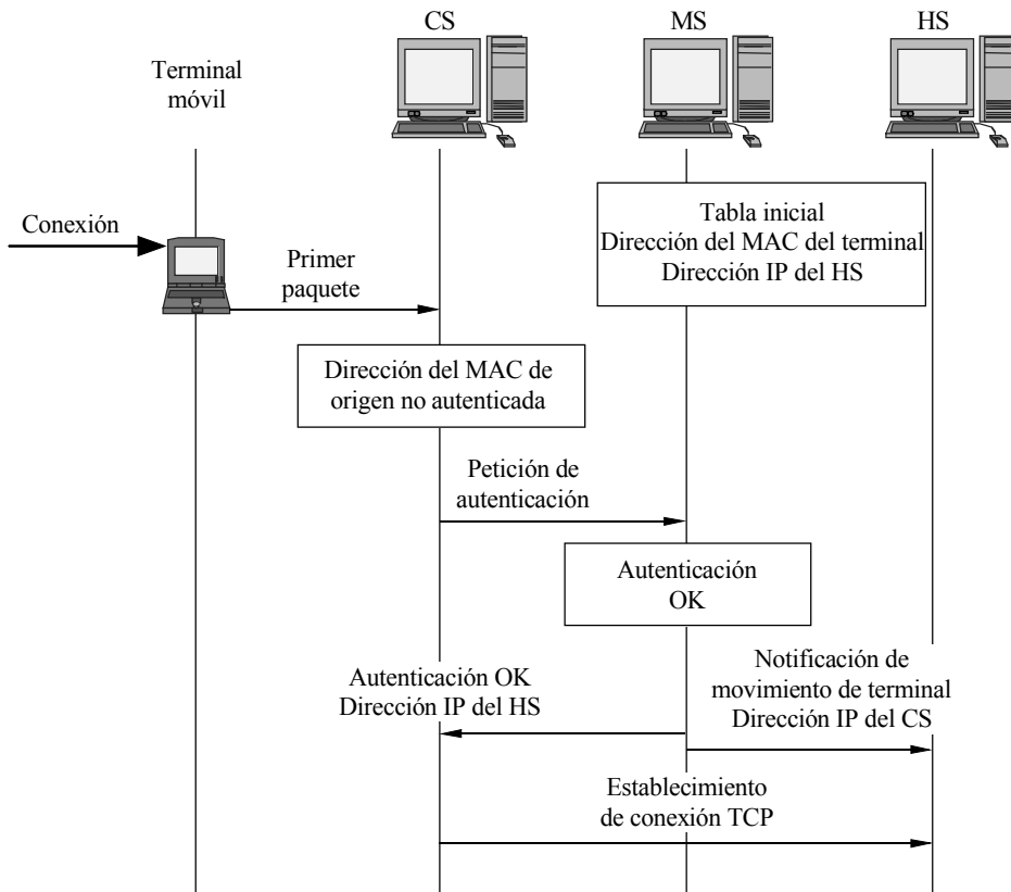
FIGURA 7 Diagrama secuencial de la autenticación de terminal, registro de emplazamiento y conexión
