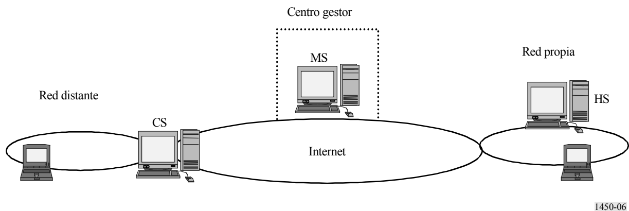
FIGURA 6 Composición de un sistema VLAN móvil
