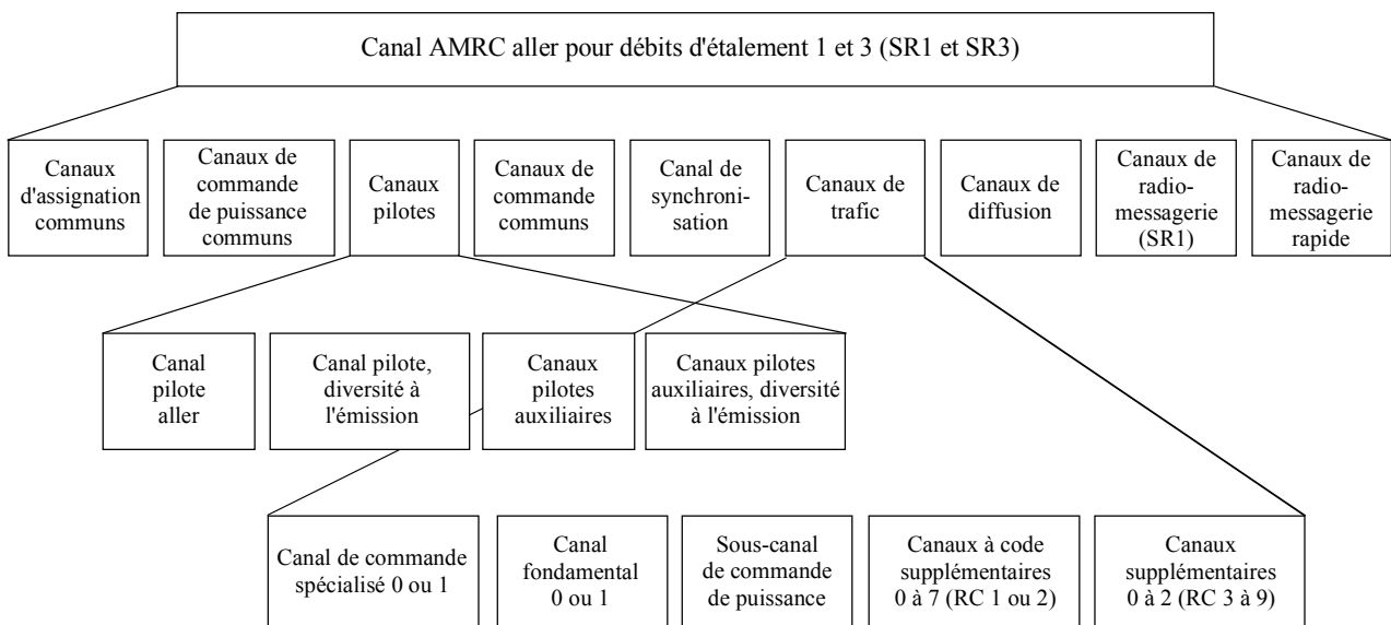
FIGURE 18 Canaux AMRC aller reçus à la station mobile
