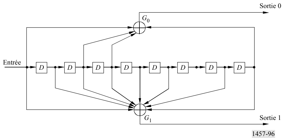
Générateur de code convolutif, taux = 1/2, longueur de contrainte = 9
