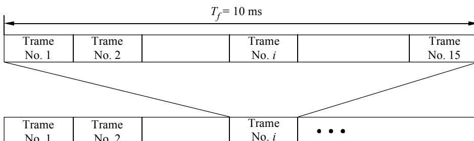
FIGURE 8 Structure de base des trames
