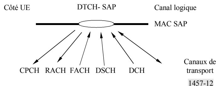
FIGURE 12 Possibilités de mappage du canal DTCH sur des canaux de transport (Les flèches indiquent le sens du canal (côté UE). Les directions sont opposées vues depuis le réseau)
