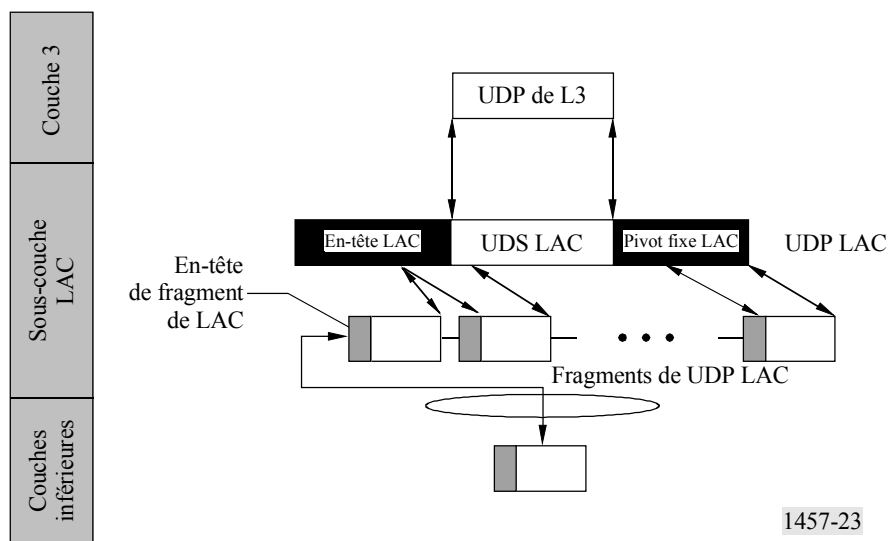
Traitement des unités de données LAC
