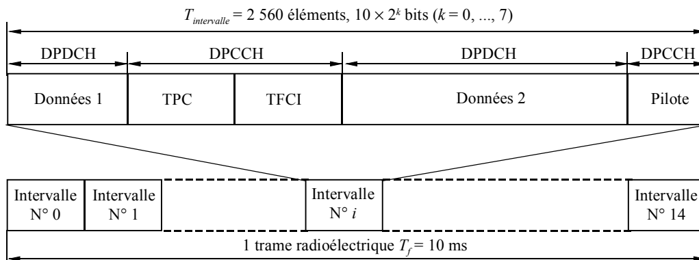
FIGURE 84 Format de trame pour le canal DPCH de liaison descendante
