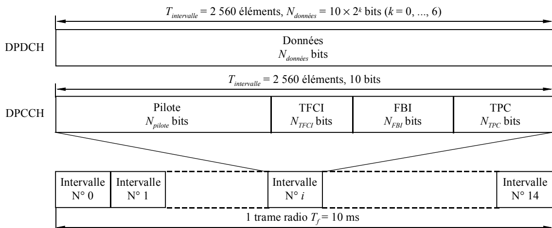
Structure de trame pour le canal DPCH de la liaison montante
