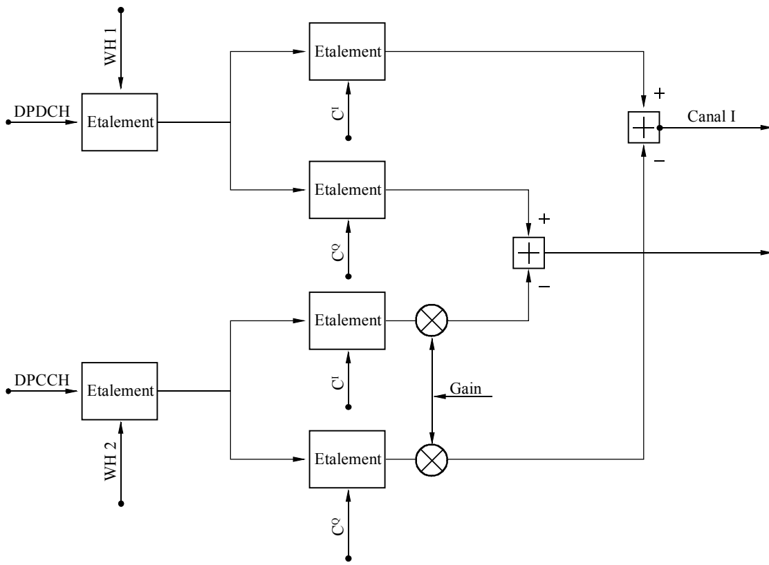
Système de modulation par étalement sur la liaison retour pour des canaux physiques spécialisés a) et sa représentation complexe b)
