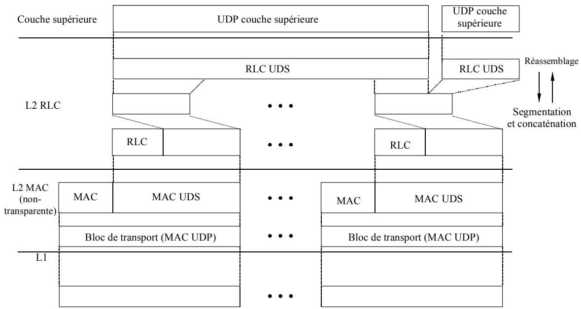
FIGURE 28 Flux de données associés à un service utilisant une sous-couche RLC et une couche MAC non transparentes (voir les § 5.3.1.4.1 et 5.3.1.4.2 pour la définition plus précise des services et fonctionnalités RLC et MAC)
