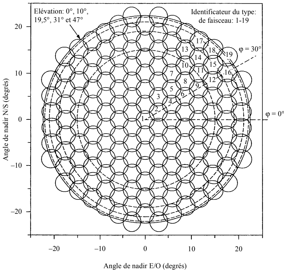
Grille hexagonale représentant les 19 types de faisceau
