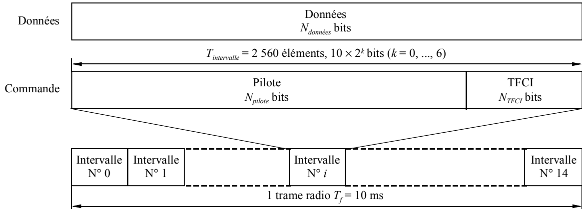
Structure de trame pour les parties données et commande de liaison montante associées à un canal PCPCH
