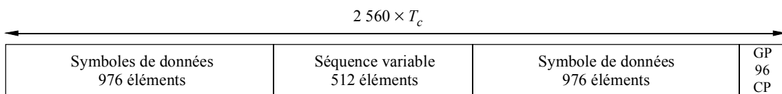
FIGURE 32 Structure des salves pour le type de salve 1 (GP correspond à la période de garde et CP aux périodes des éléments)
