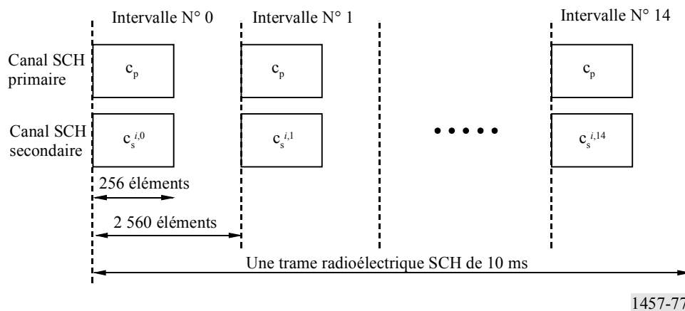
Structure du canal de synchronisation (SCH)
