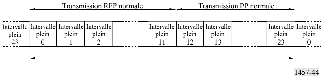
FIGURE 44 Structure des trames utilisant le format d'intervalle plein
