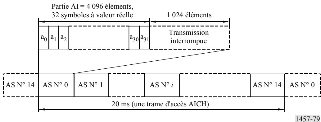
Structure du canal indicateur d'acquisition (AICH)
