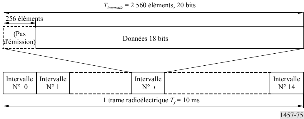
FIGURE 75 Format des trames du canal physique de commande commun primaire (P-CCPCH)
