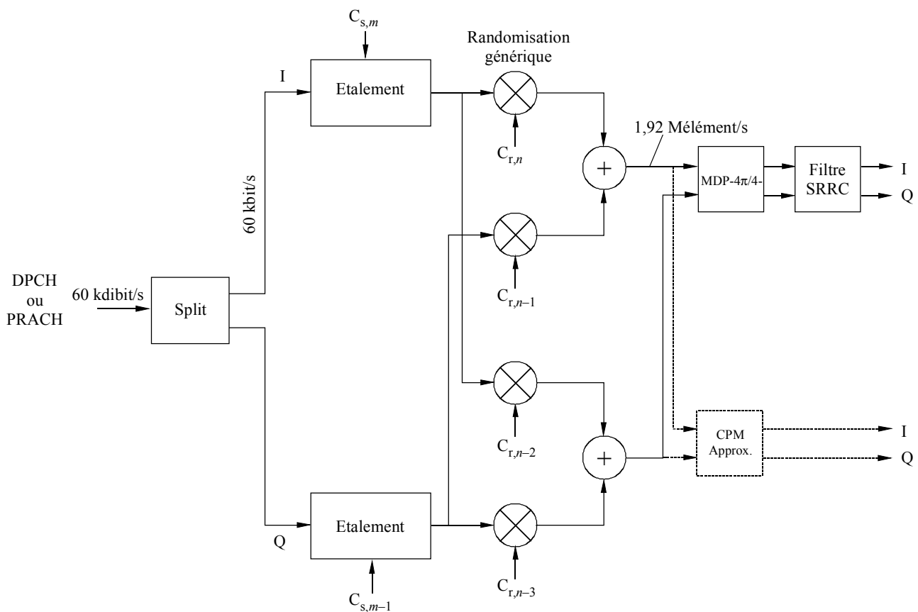
Etaleur et modulateur génériques de la liaison retour (Les débits indiqués correspondent à l'option à 1,92 Mélément/s et à un facteur d'étalement de 32)
