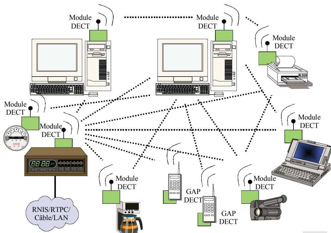
Réseau LAN hertzien ethernet DECT avec communication décentralisée et capacité vocale additionnelle
