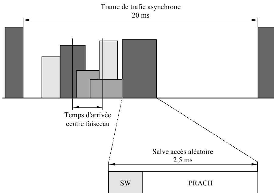
FIGURE 59 Trafic asynchrone dans la liaison retour, trame 0
