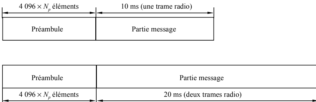
FIGURE 86 Structure de la transmission à accès aléatoire
