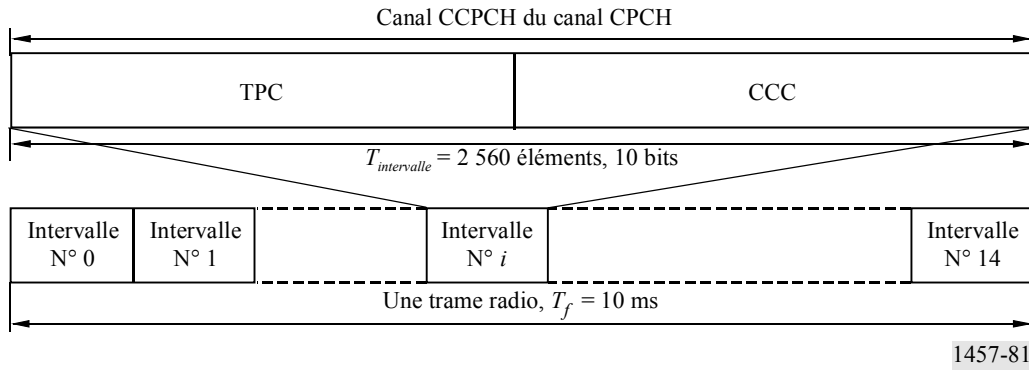
FIGURE 81 Structure de trame du canal CPCH-CCPCH de liaison descendante
