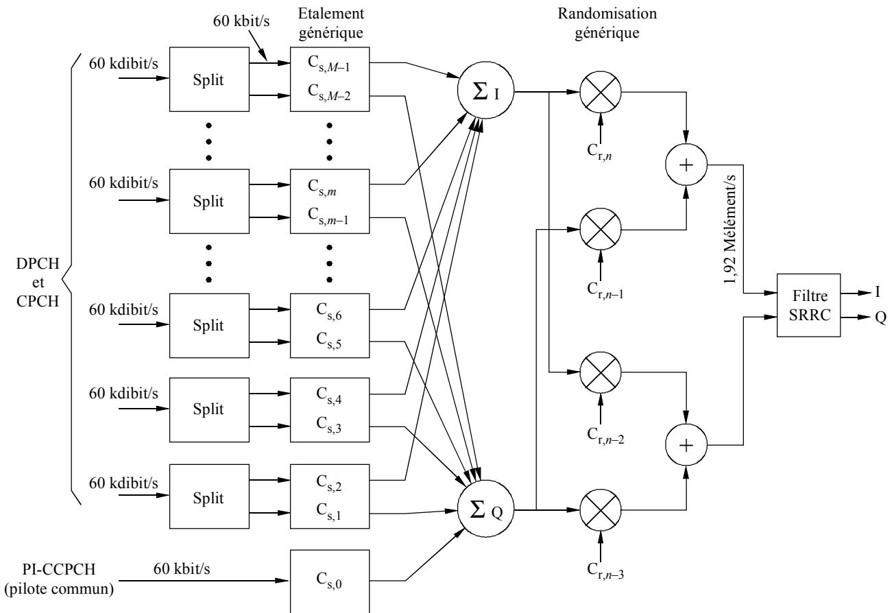
Etaleur et modulateur générique de la liaison aller (Les débits indiqués correspondent à l'option à 1,920 Mélément/s et à un facteur d'étalement de 32)
