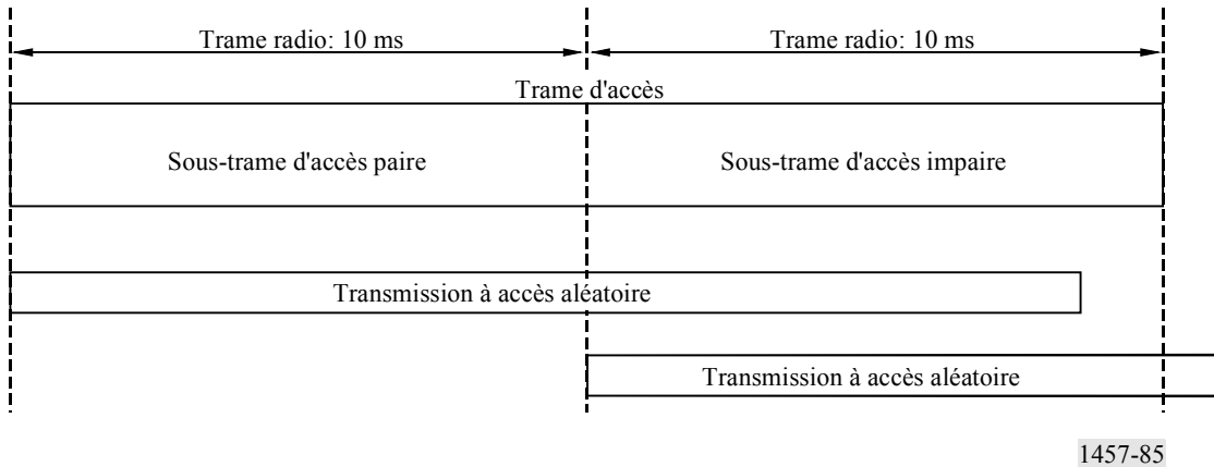
FIGURE 85 Trame d'accès aléatoire
