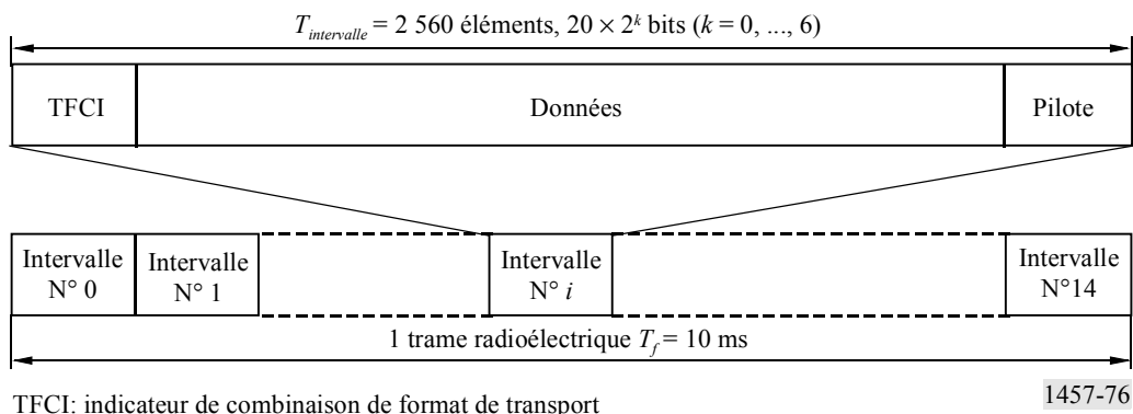
FIGURE 76 Format des trames pour le canal physique de commande commun secondaire (S-CCPCH)
