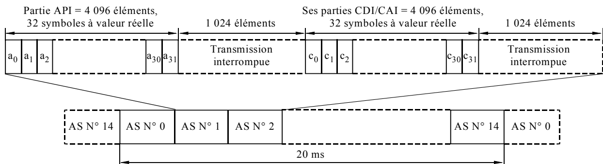
Structure du canal d'indicateur APA/CD/CA (APA/CD/CA-AICH)
