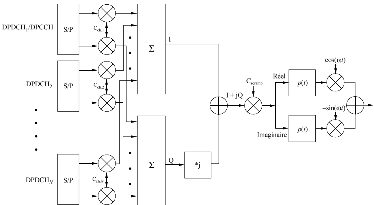
Etalement/modulation pour le canal DPCH sur liaison descendante
