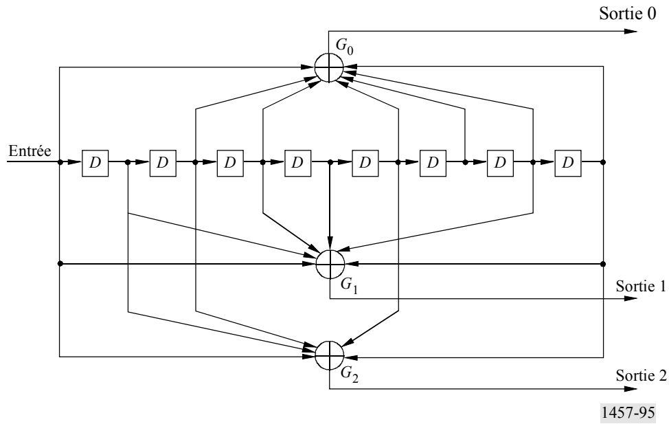
Générateur de code convolutif, taux = 1/3, longueur de contrainte = 9
