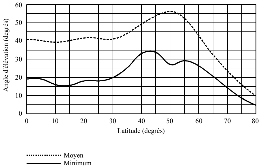
FIGURE 69 Distribution en fonction de la latitude des angles d'élévation minimum et moyen
