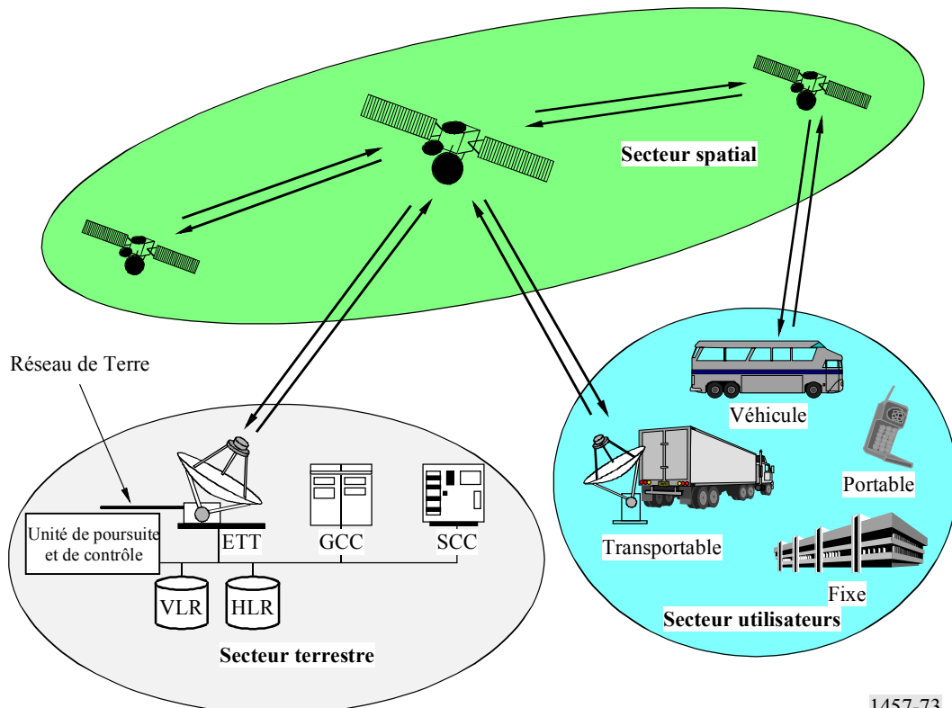
FIGURE 73 Architecture du système
