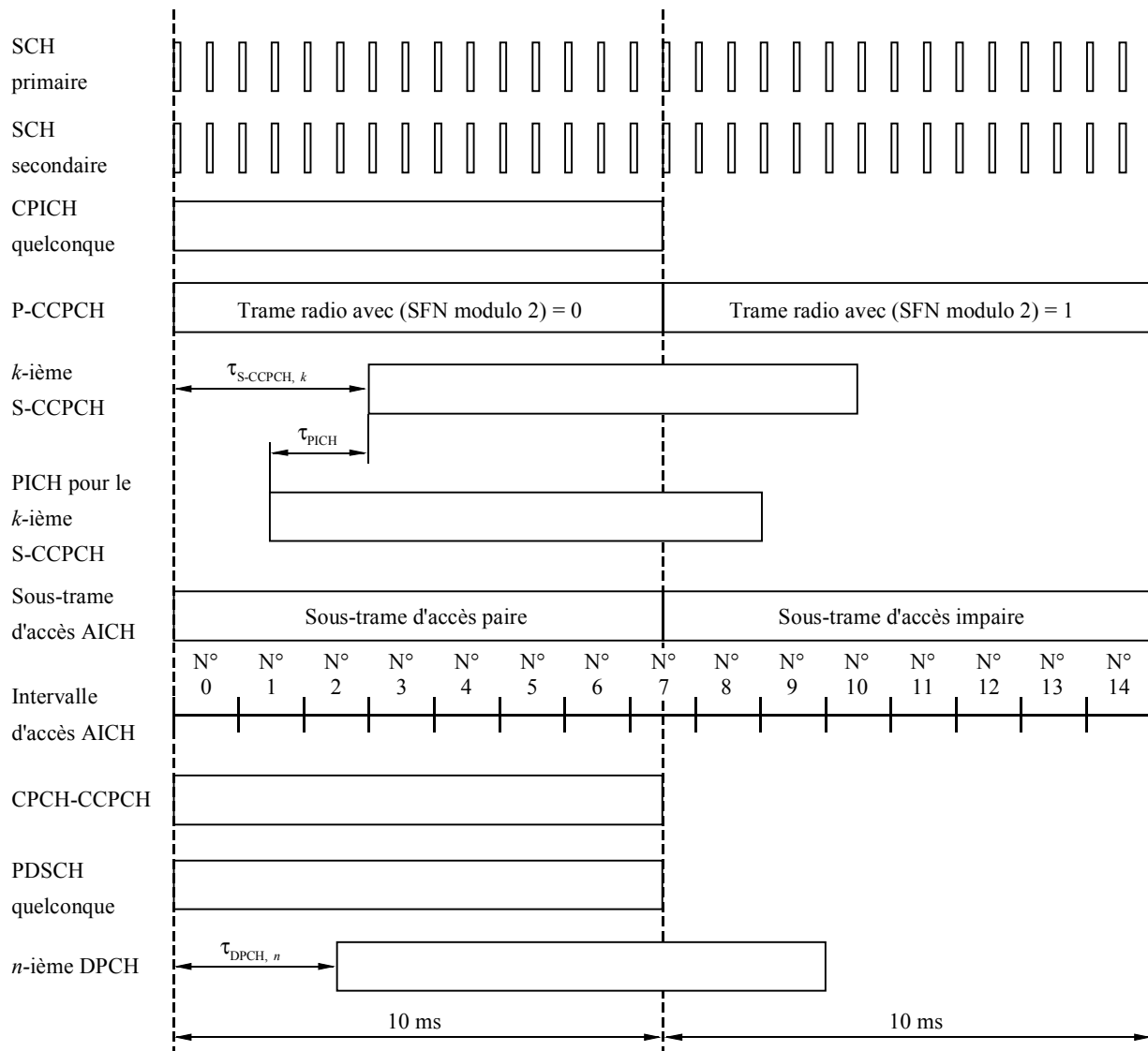
FIGURE 91 Structure temporelle de la trame et structure temporelle des intervalles d'accès des canaux physiques de liaison descendante
