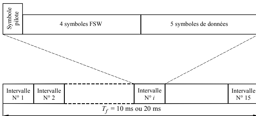
FIGURE 52 Structure des trames pour les canaux physiques de commande communs (CCPCH)
