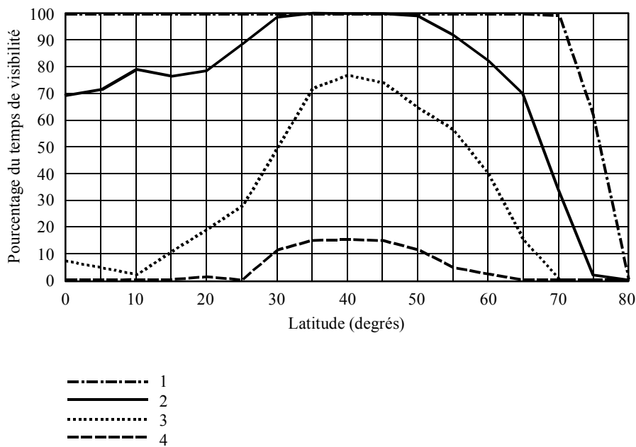
FIGURE 70 Pourcentage du temps de visibilité des satellites avec un angle d'élévation minimum supérieur à 15°
