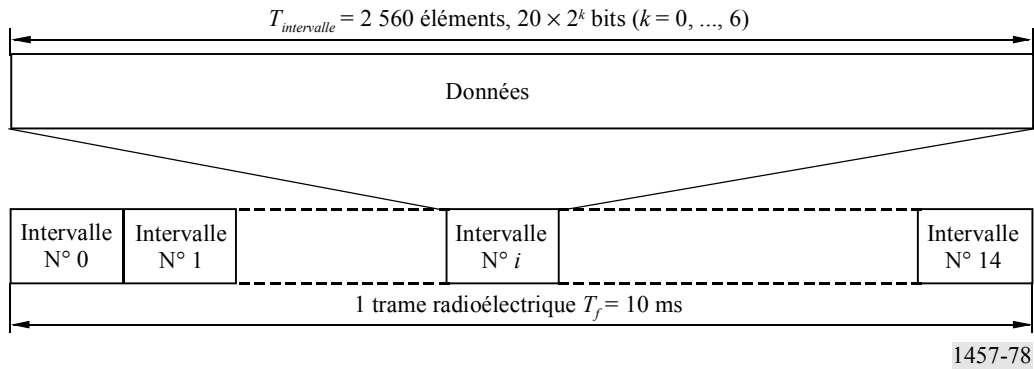
Format de trame pour le canal partagé physique de liaison descendante (PDSCH)
