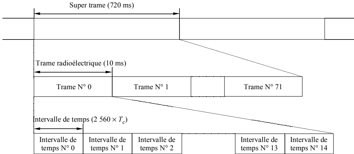
FIGURE 31 Structure de base des trames
