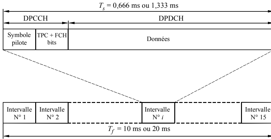
FIGURE 51 Structure des trames des canaux physiques spécialisés de la liaison aller (DPDCH/DPCCH)
