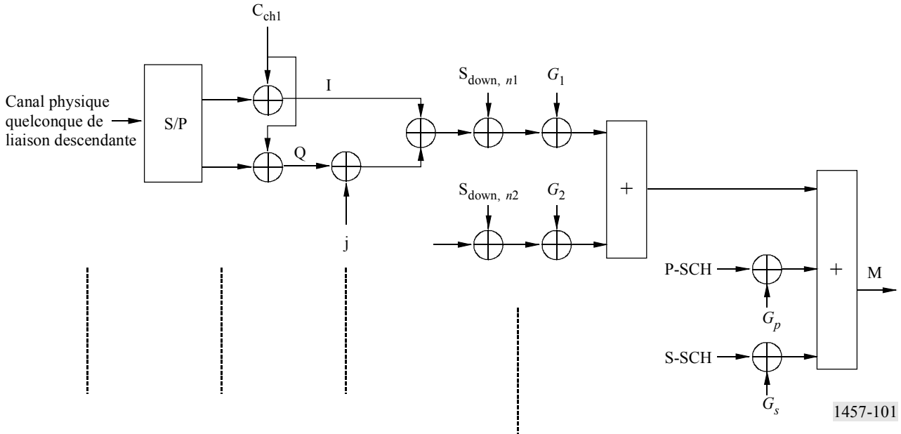
Etalement: canaux physiques de liaison descendante
