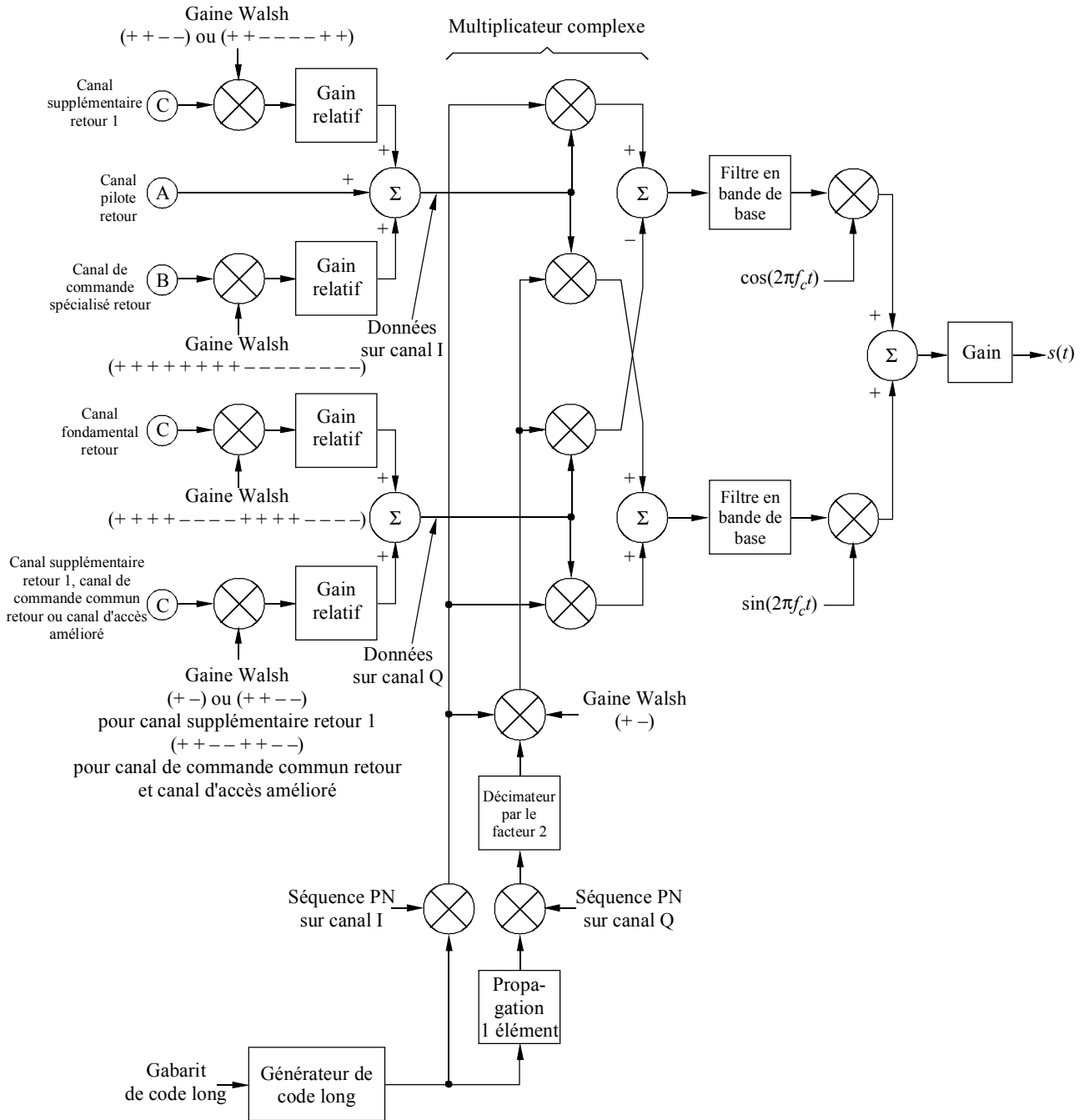
FIGURE 16 Etalement et modulation de la liaison montante pour les configurations radioélectriques 3 à 6
