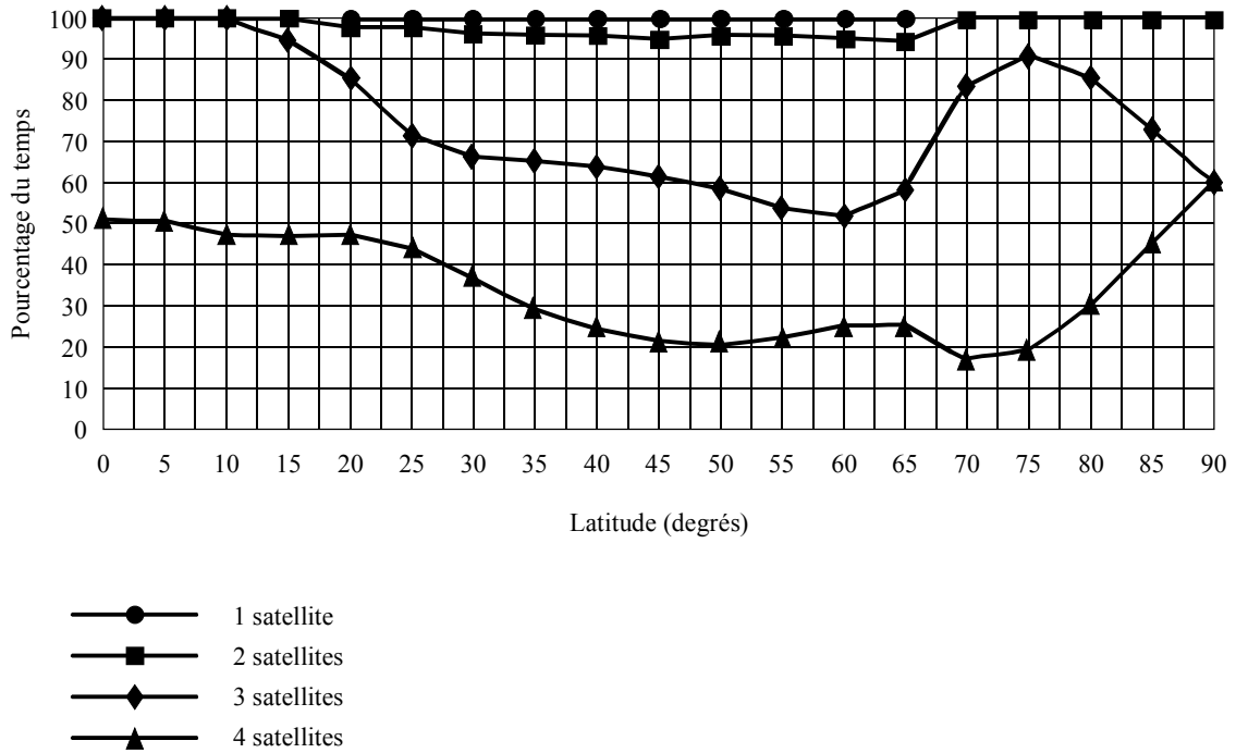
Statistiques courantes de visibilité pour une constellation de satellites (10 satellites)
