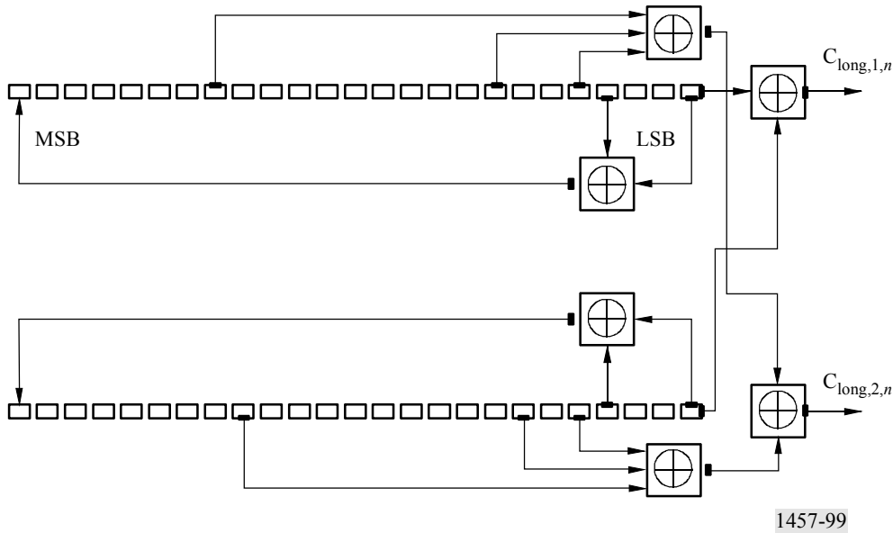
FIGURE 99 Générateur à codes longs de la liaison montante
