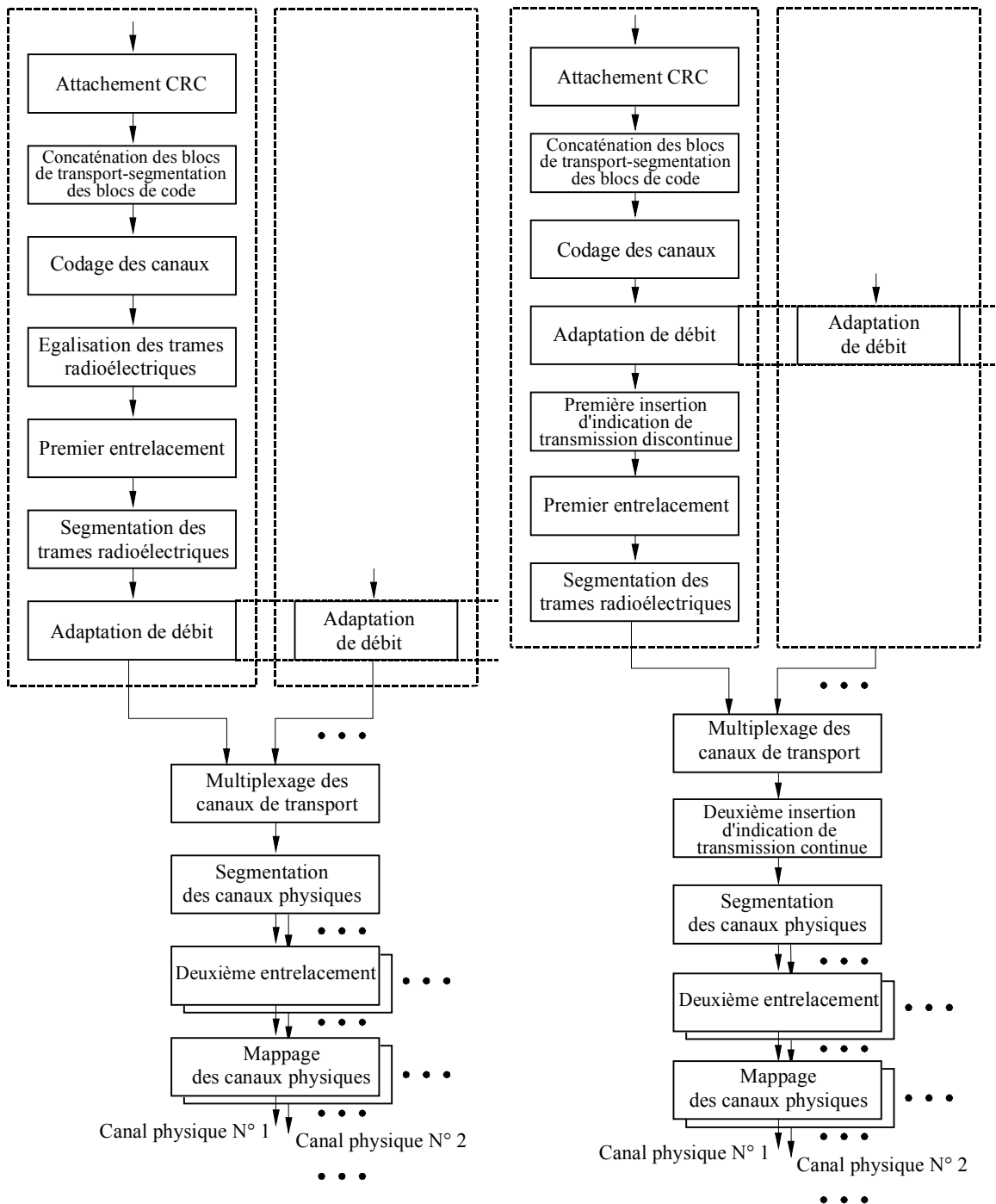
FIGURE 94 Schéma de passage d'un canal de transport à un canal physique (gauche: liaison montante, droite: liaison descendante)
