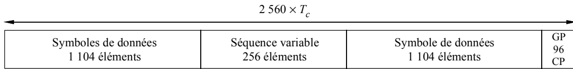
FIGURE 33 Structure des salves pour le type de salve 2 (GP correspond à la période de garde et CP aux périodes des éléments)
