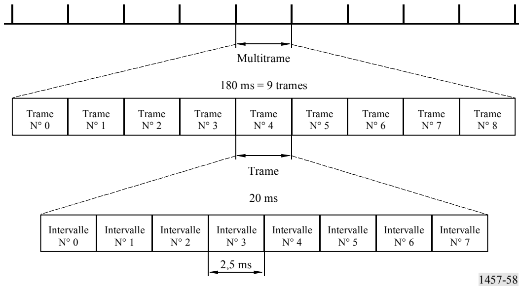
FIGURE 58 Structure des trames sur les liaisons aller et retour
