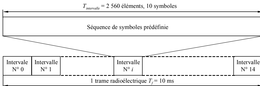
Format des trames sur le canal pilote commun (CPICH)
