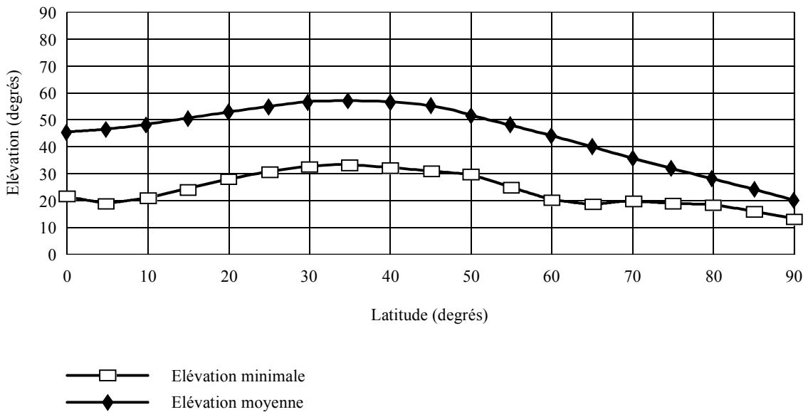
Angles d'élévation typiques minimal et moyen du satellite le plus proche (10 satellites)
