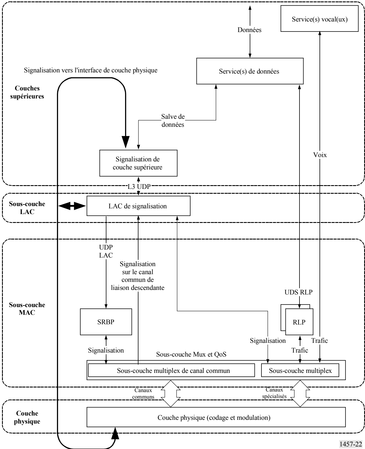
FIGURE 22 Structure en couches et interfaces de services (station mobile)
