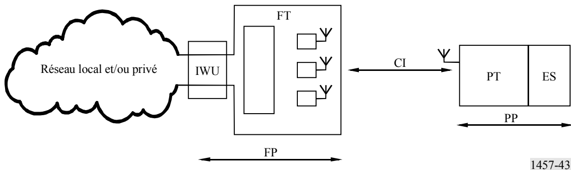
FIGURE 43 Structure de l'interface commune (CI)
