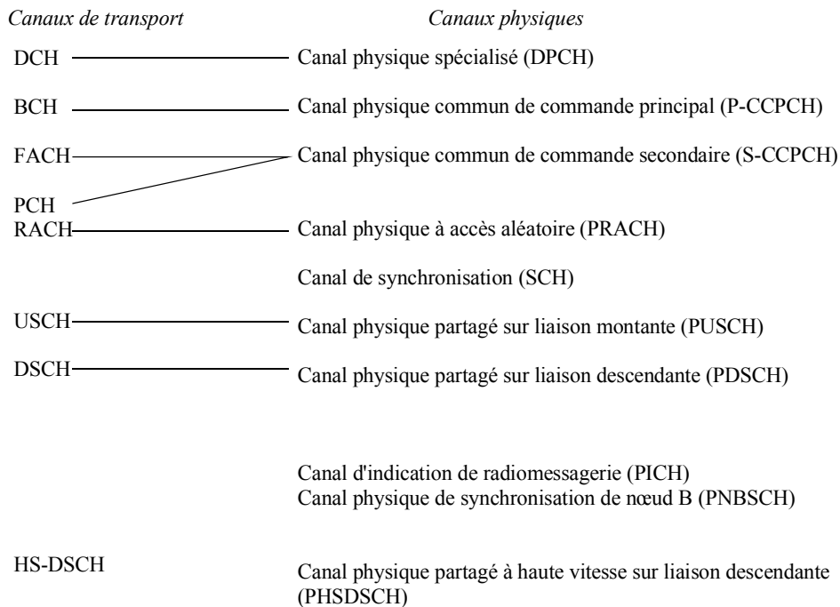
FIGURE 30 Canaux de transport, canaux physiques et leur mappage
