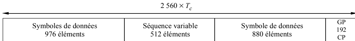
FIGURE 34 Structure des salves pour le type de salve 3 (GP correspond à la période de garde et CP aux périodes des éléments)
