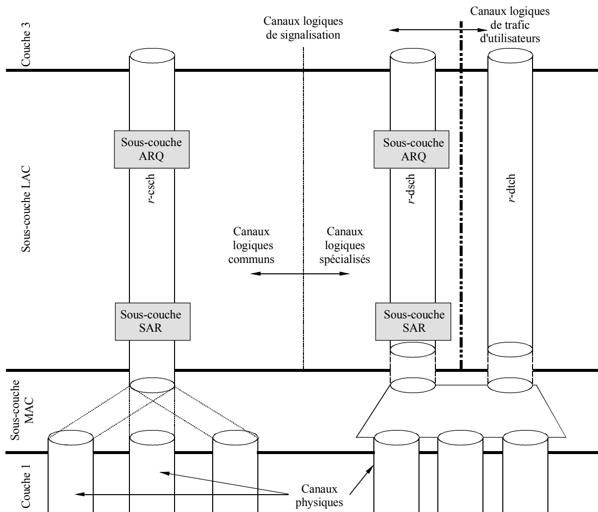
FIGURE 25 Architecture d'un canal logique sur la liaison montante
