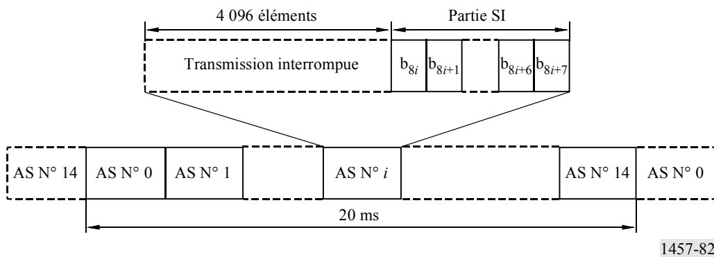
FIGURE 82 Structure du canal indicateur d'état du canal CPCH (CSICH)
