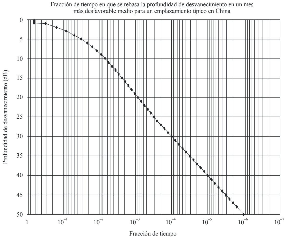
FIGURA 4 Profundidad de desvanecimiento en función del tiempo
