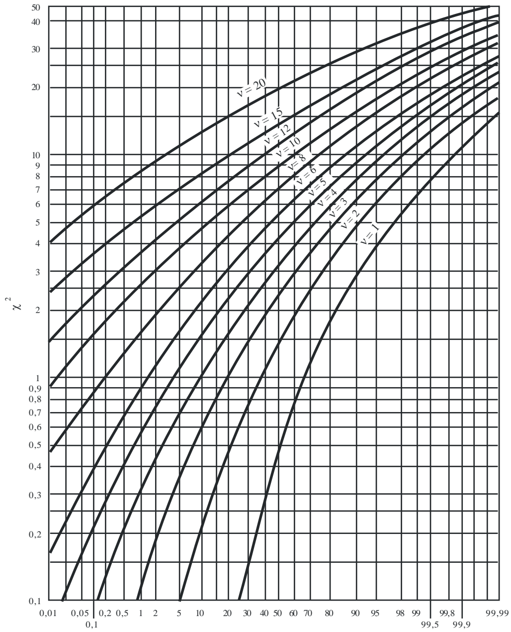
FIGURA 7 Distribución de probabilidad \chi^2
