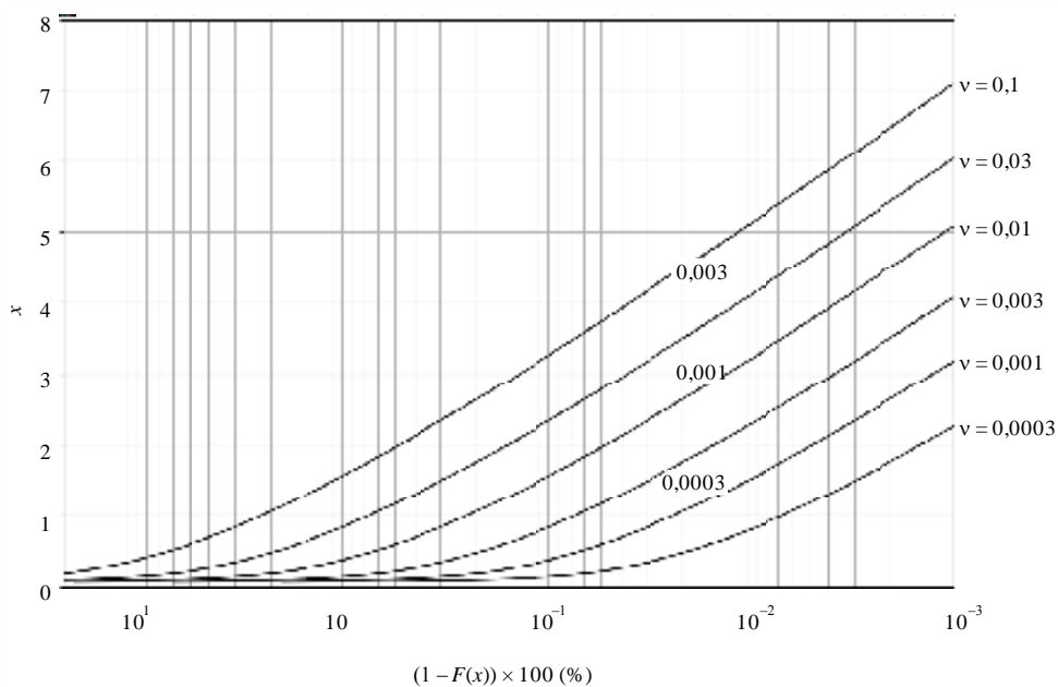
FIGURA 5 Distribución de probabilidad gamma \alpha = 1, \nu \leq 0,1
