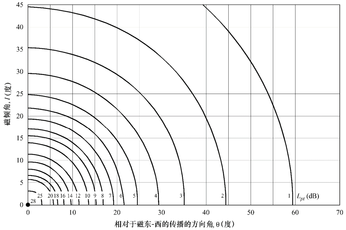
图 7 过极化耦合损耗 L_p (单个终端)
