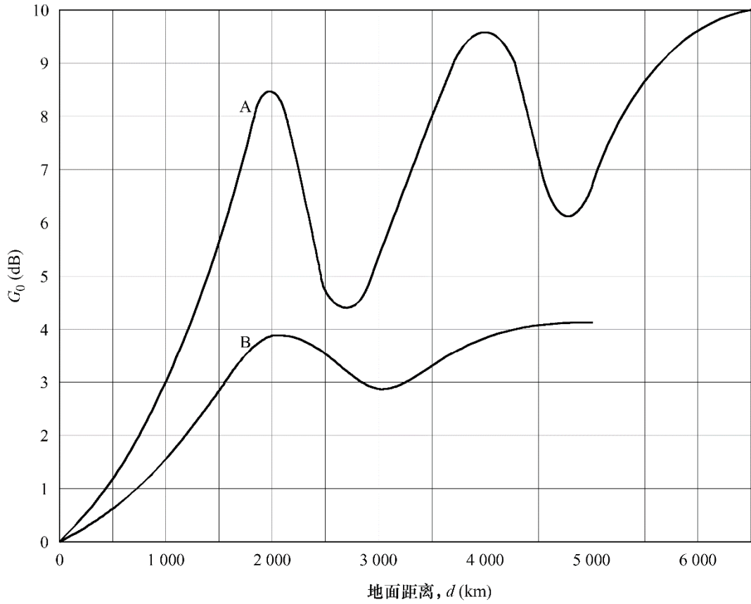
图 2 位于海岸的单个终端的海洋增益 ( G_0 )
