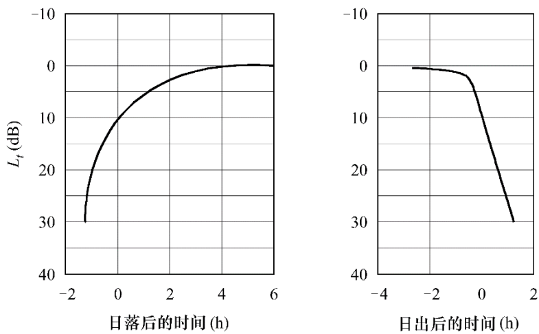
图 3 以小时计的损耗因子 ( L_t )
