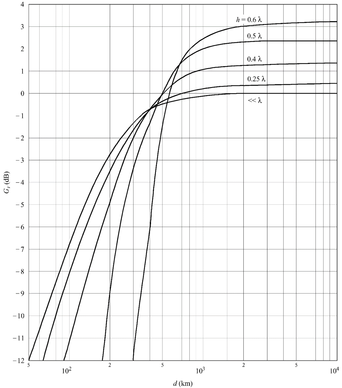
图 1 位于良好大地上的单极天线的发射天线增益因子 ( G_V )
