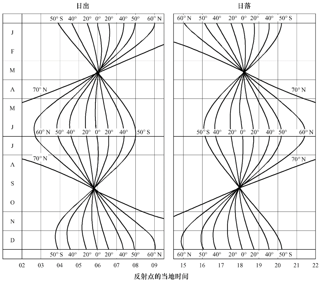
图 11 不同月份和地理纬度的日出和日落的时间
