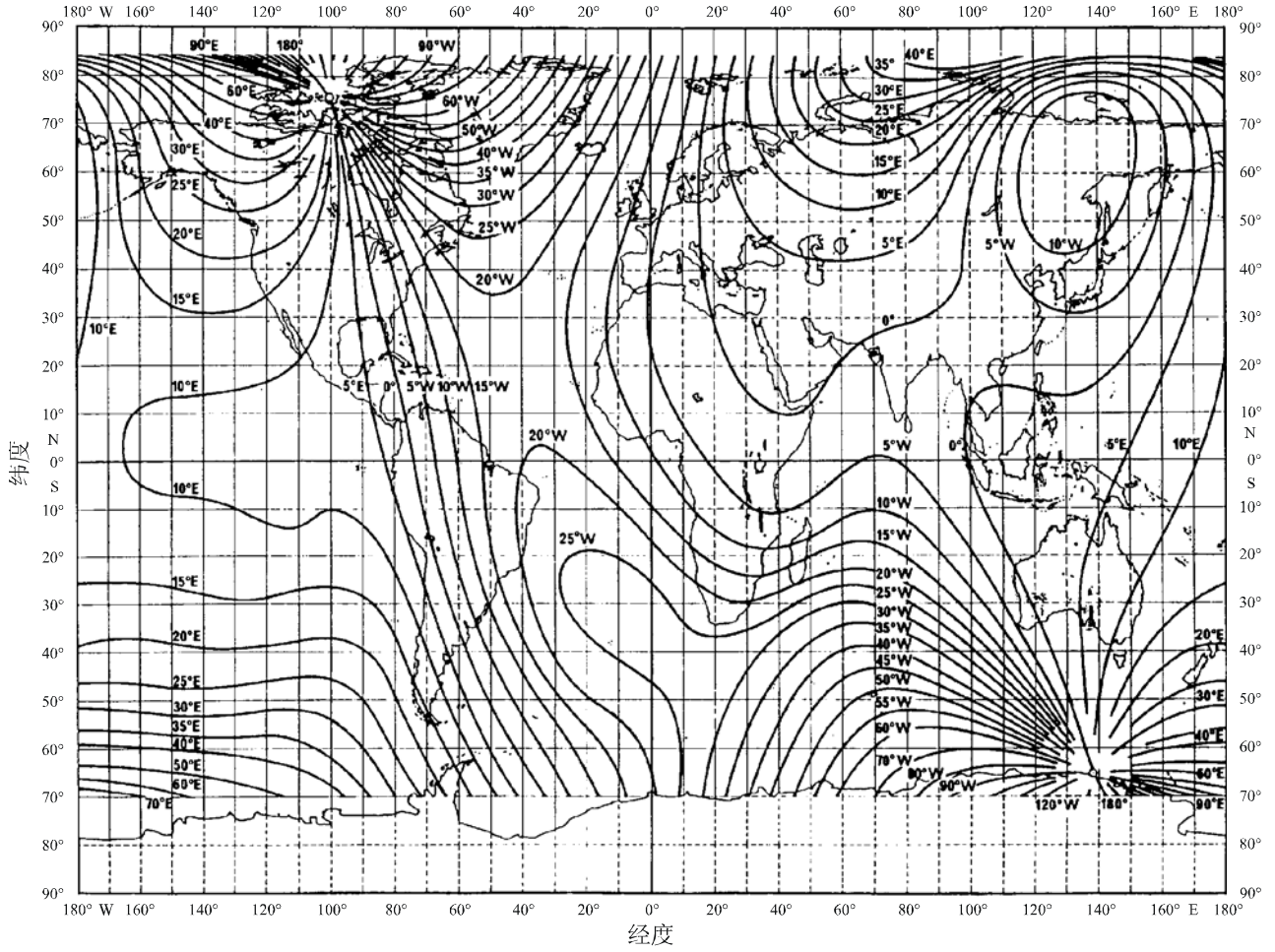
图 6 磁偏角图 (绘制时间1975.0)
