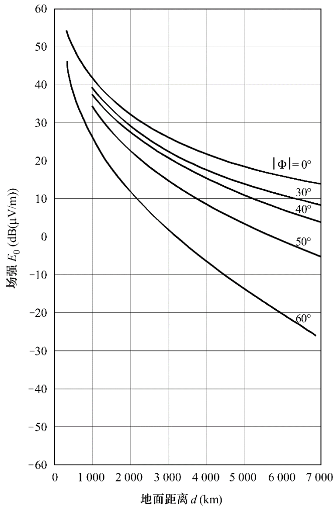
图 4b 当 G_s, L_p 和 R 都为零，地磁纬度不变时， 在 MF 的表示 E_0 的曲线
