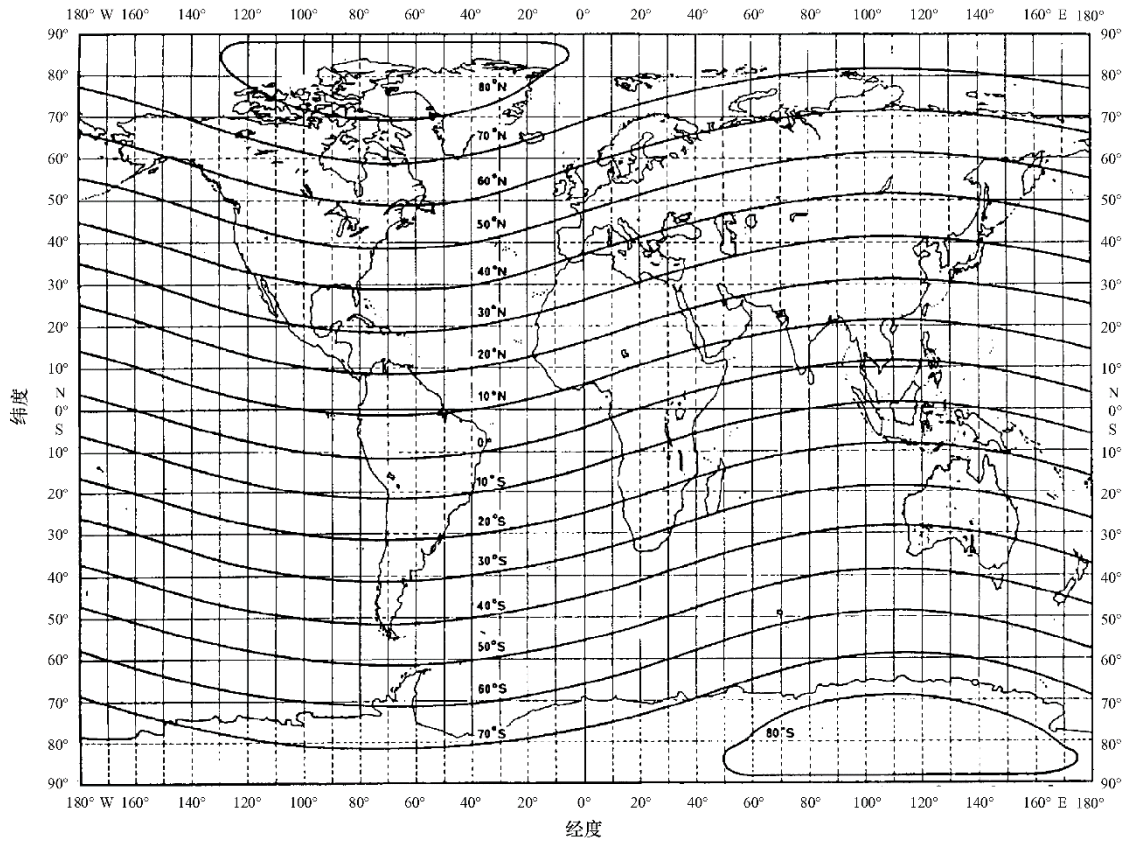
图 10 地磁纬度
