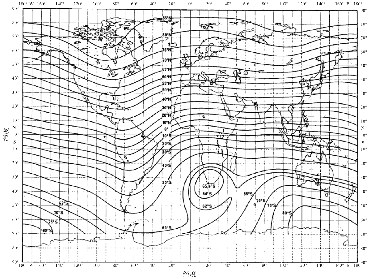
图 5 磁倾角图 (绘制时间 1975.0)
