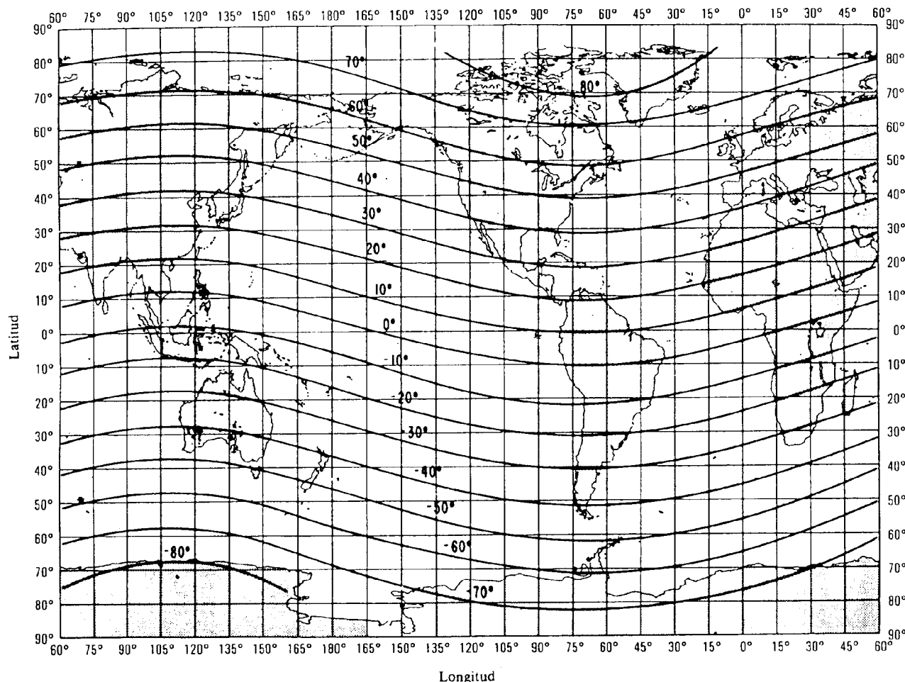
FIGURA 2 Latitudes geomagnéticas
