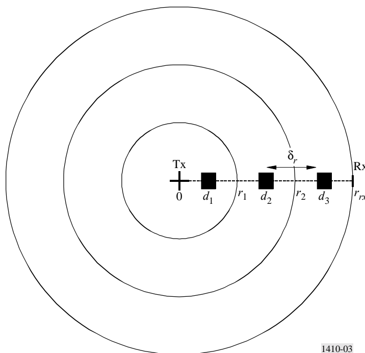
FIGURE 3 Emplacements des bâtiments par rapport au récepteur (Rx) situé à une distance r_{rx} de l'émetteur (Tx)
