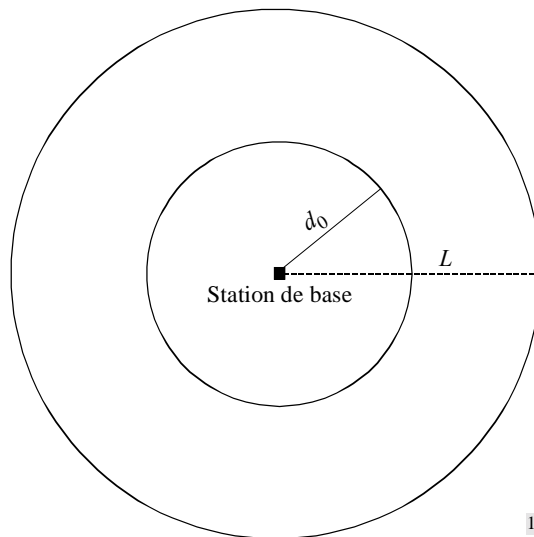
FIGURE 6 Schéma de la cellule à station centrale représentant le rayon de la zone de couverture équivalente durant les précipitations
