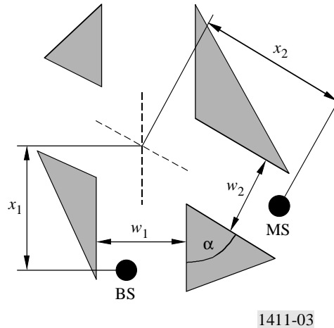
FIGURE 3 Définition des paramètres correspondant au cas NLOS2
