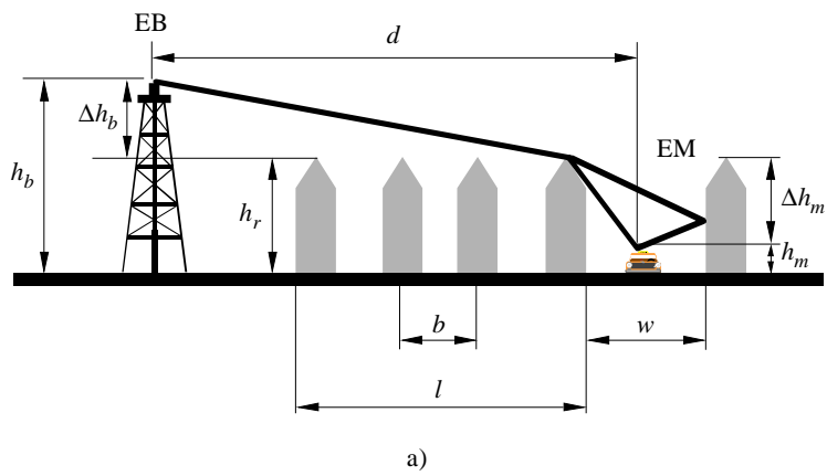
FIGURA 2 Definición de los parámetros del caso NLoS1
