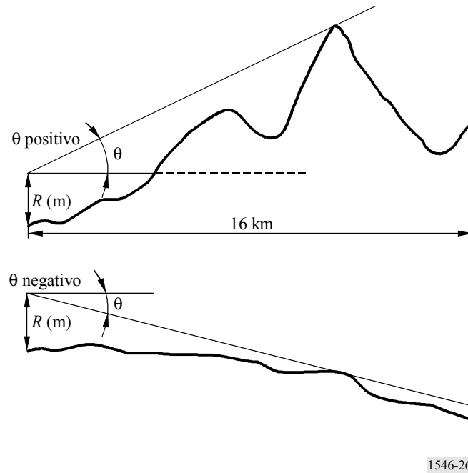
FIGURA 26 Ángulo de despejamiento del terreno
