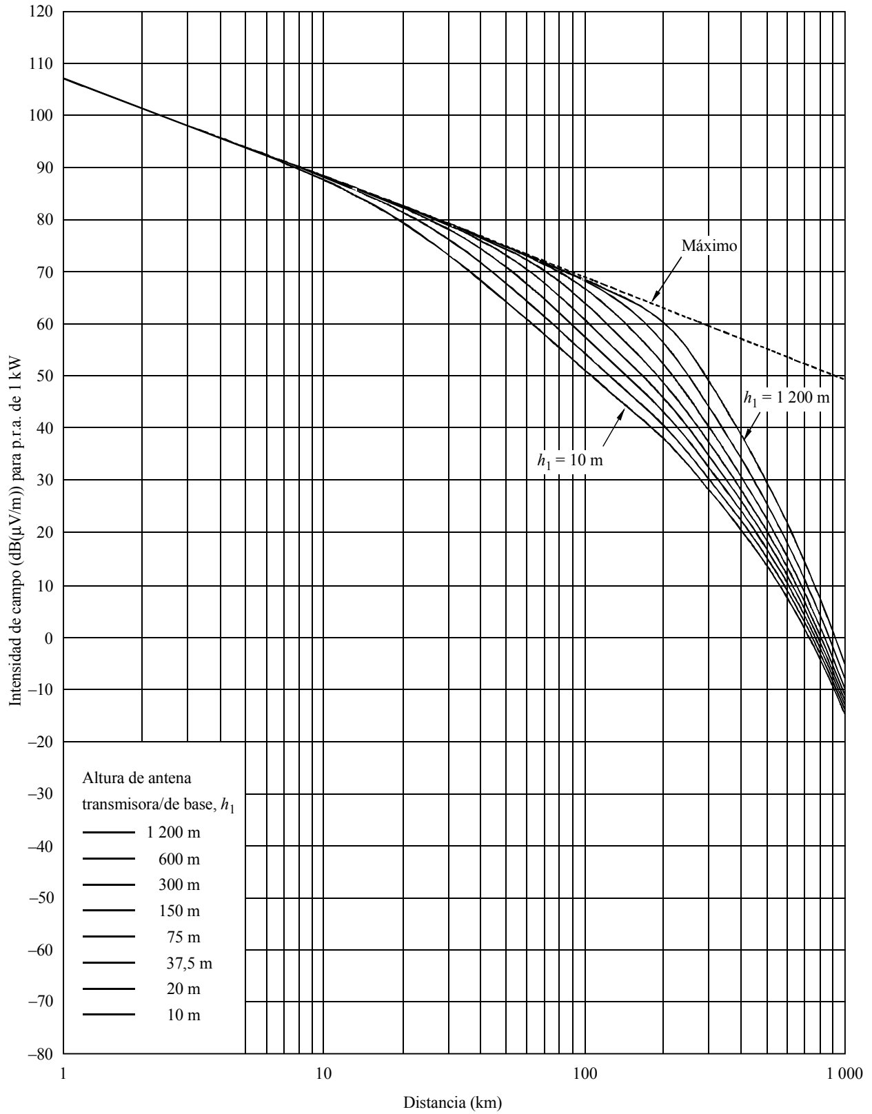
FIGURA 23 2 000 MHz, trayecto sobre mares cálidos, 10% del tiempo
