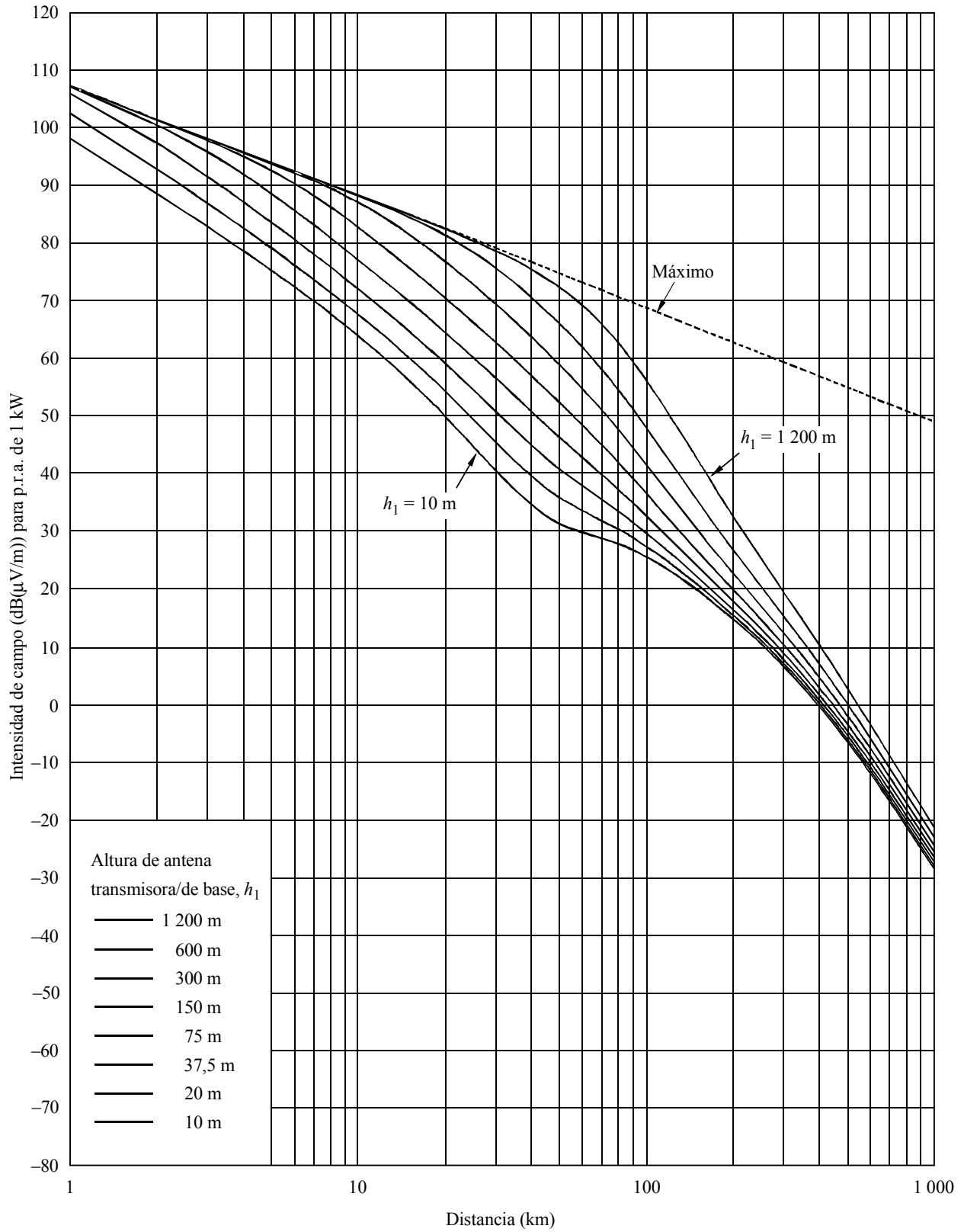
FIGURA 7 100 MHz, trayecto sobre mares cálidos, 10% del tiempo
