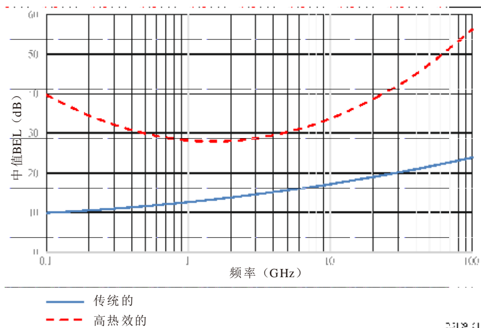
图1 以水平发生率预测的建筑物入口损耗中值
