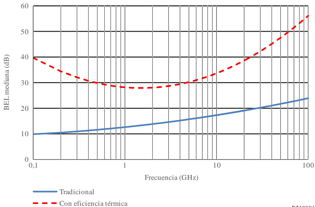
FIGURA 1 Pérdidas medias por penetración en edificios con una incidencia horizontal
