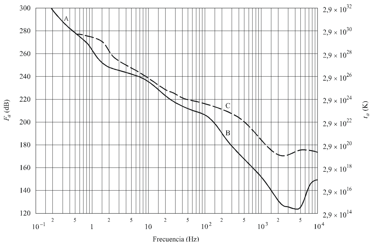
FIGURA 1 F_a máximo y mínimo en función de la frecuencia (0,1 a 10^4 Hz)
