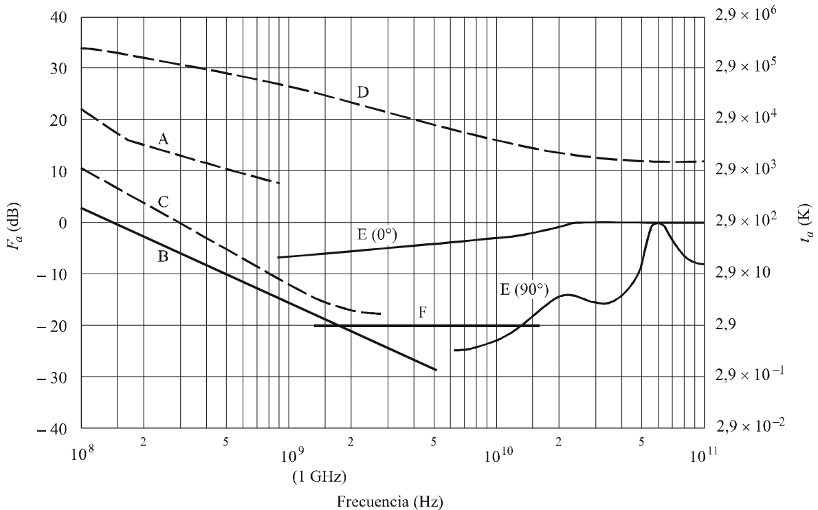
FIGURA 3 F_a en función de la frecuencia ( 10^8 a 10^{11} Hz)
