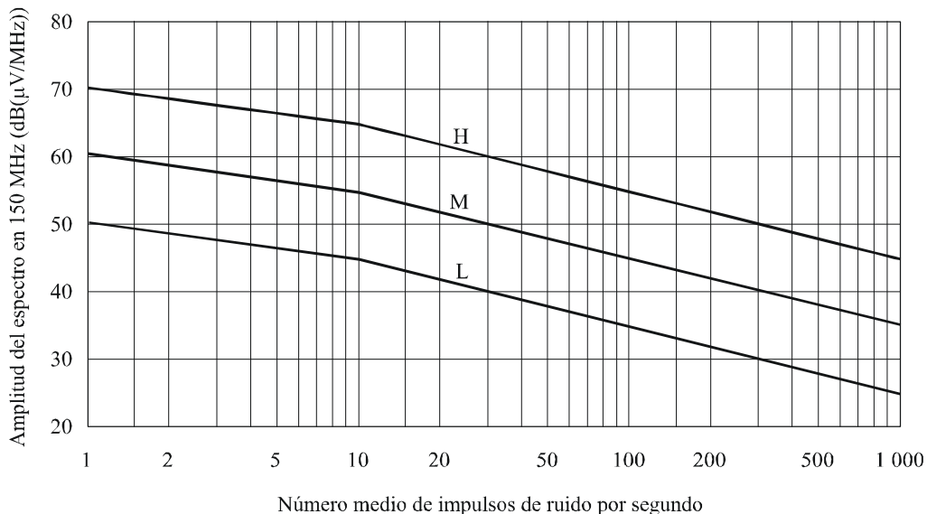
FIGURA 11 Distribución de amplitud del ruido en una estación de base (150 MHz)
