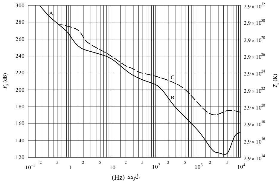
F_a ، الدنيا والقصوى بدلالة التردد (0,1 إلى 10 4 Hz)
