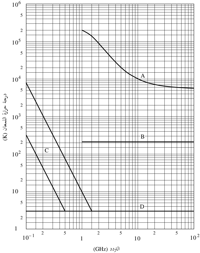
الشكل 12 مصادر الضوضاء من خارج الأرض
