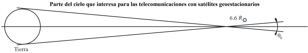
a) La órbita de los satélites geoestacionarios vista desde la Tierra mostrando \theta_0 ( R_0 : radio medio de la Tierra)
