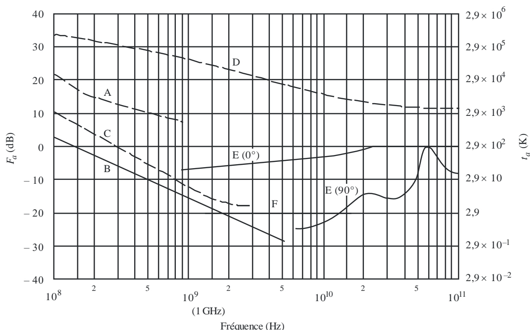
FIGURE 3 F_a en fonction de la fréquence ( 10^8 à 10^{11} Hz)
