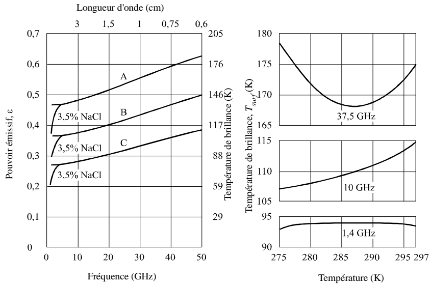
a) Pouvoir émissif d'une surface d'eau lisse
