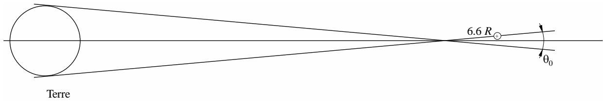
a) Orbite géostationnaire vue de la Terre montrant \theta_0 ( R_{\oplus} : rayon moyen de la Terre)
