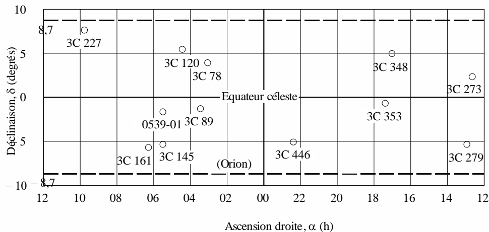
b) Emplacements des sources radioélectriques les plus puissantes (O) pour une bande de \pm 8,7^\circ de part d'autre de l'équateur céleste. Les numéros se rapportent aux désignations des catalogues, par exemple. 3C indique "third Cambridge"
