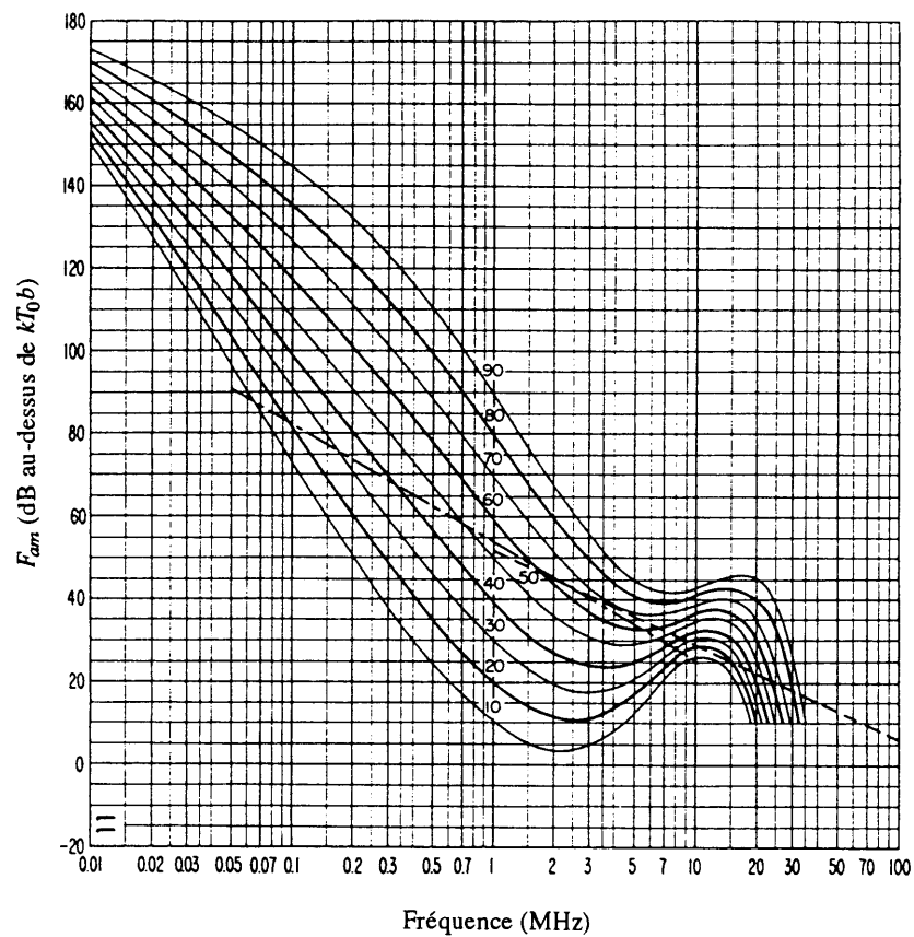
FIGURE 24b – Variation du bruit radioélectrique en fonction de la fréquence (Printemps; 1200-1600 heure locale)
