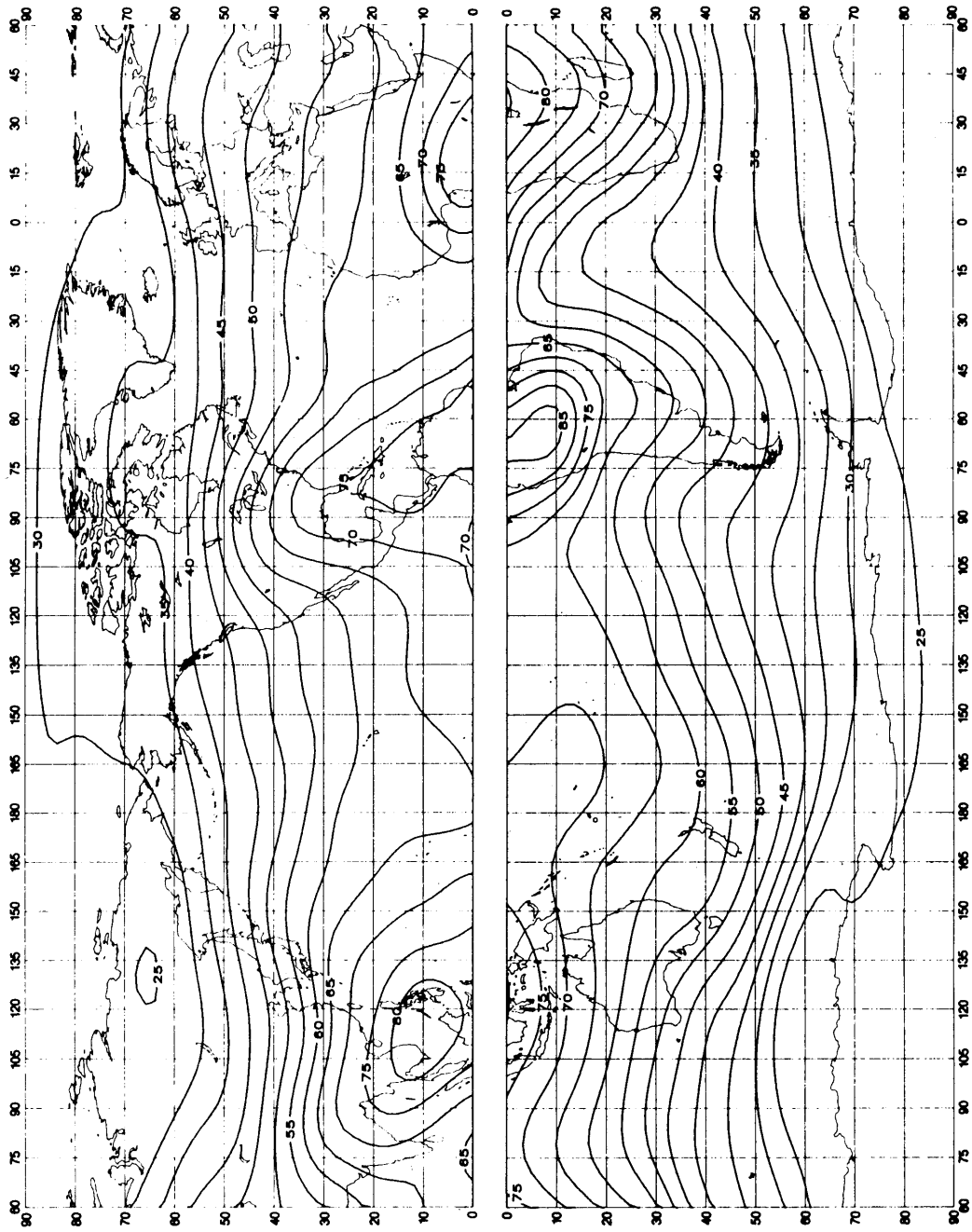
FIGURE 22a – Valeurs attendues du bruit atmosphérique radioélectrique, F_{0m} , en dB au-dessus de kT_0b à 1 MHz (Printemps; 0400-0800 heure locale)
