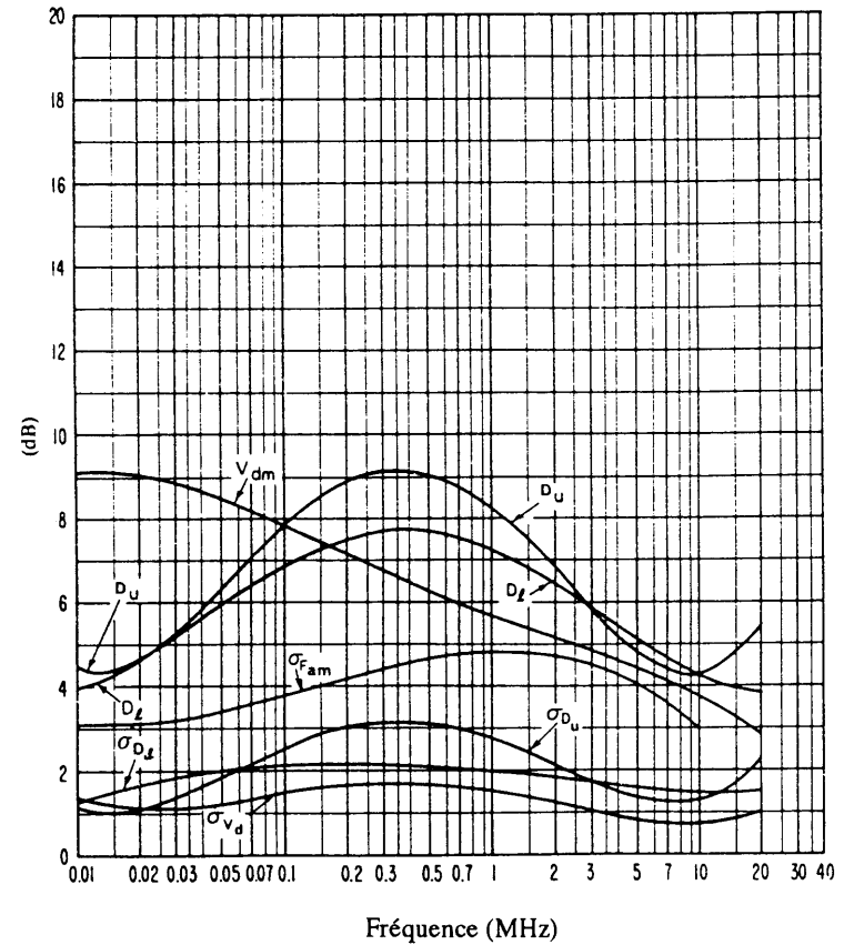
FIGURE 32c – Données sur la variabilité et le caractère du bruit (Eté; 2000-2400 heure locale)
