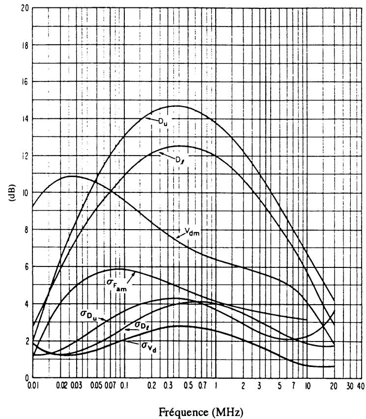
FIGURE 16c – Données sur la variabilité et le caractère du bruit (Hiver; 0400-0800 heure locale)
