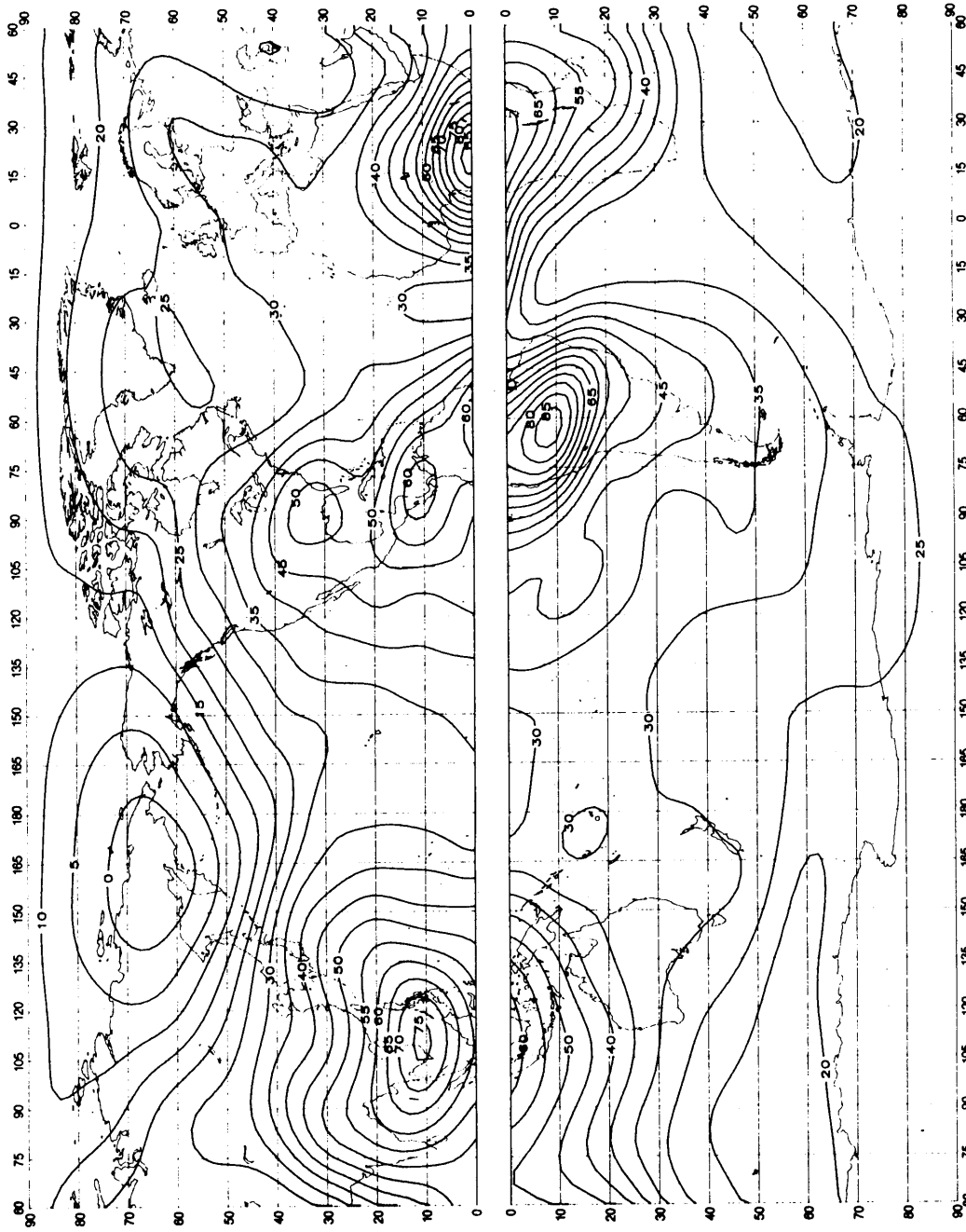
FIGURE 23a – Valeurs attendues du bruit atmosphérique radioélectrique, F_{fm} , en dB au-dessus de kT_0 à 1 MHz (Printemps; 0800-1200 heure locale)
