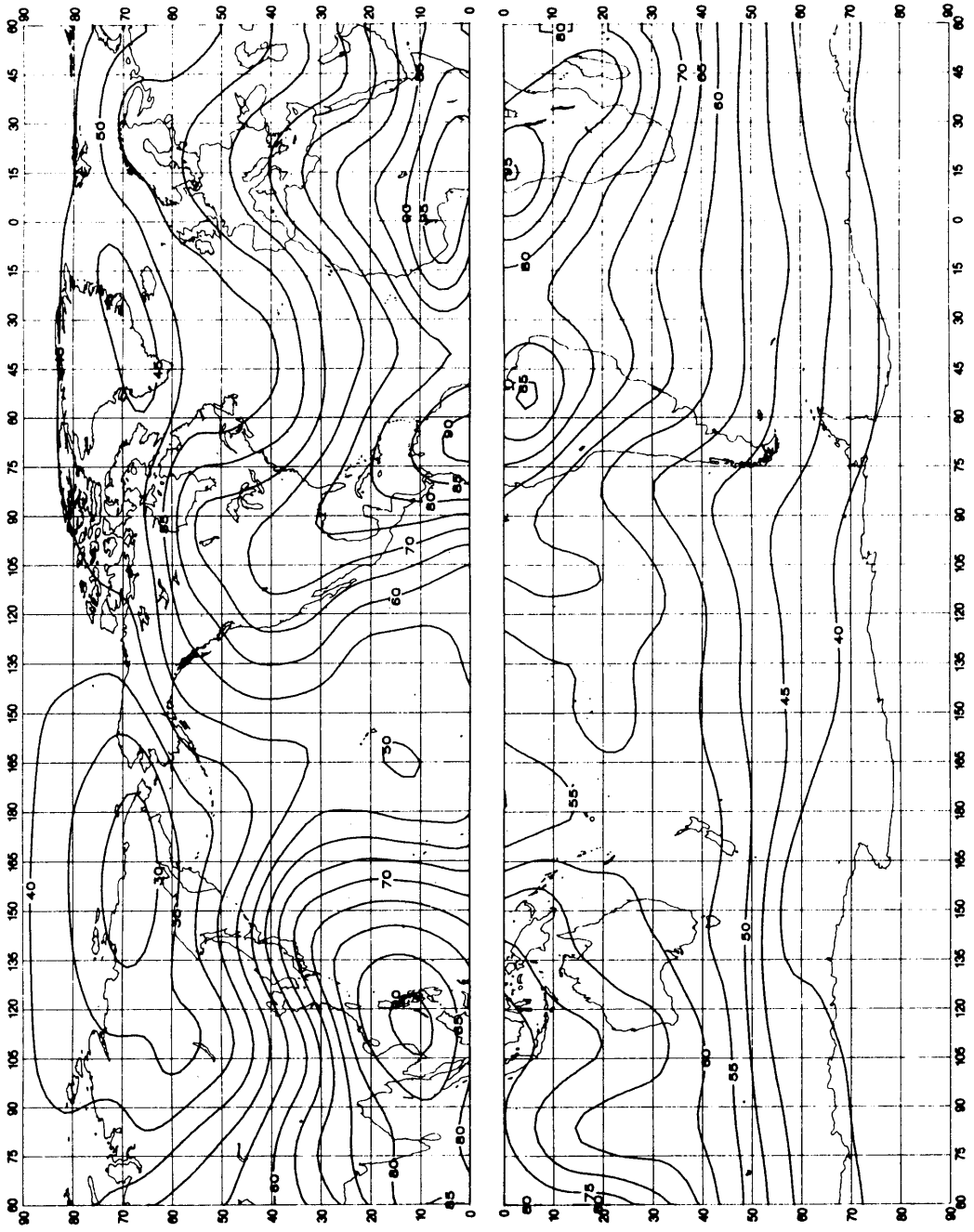
FIGURE 37a - Valeurs attendues du bruit atmosphérique radioélectrique, F_{fm} , en dB au-dessus de kT_0b à 1 MHz (Automne; 1600-2000 heure locale)
