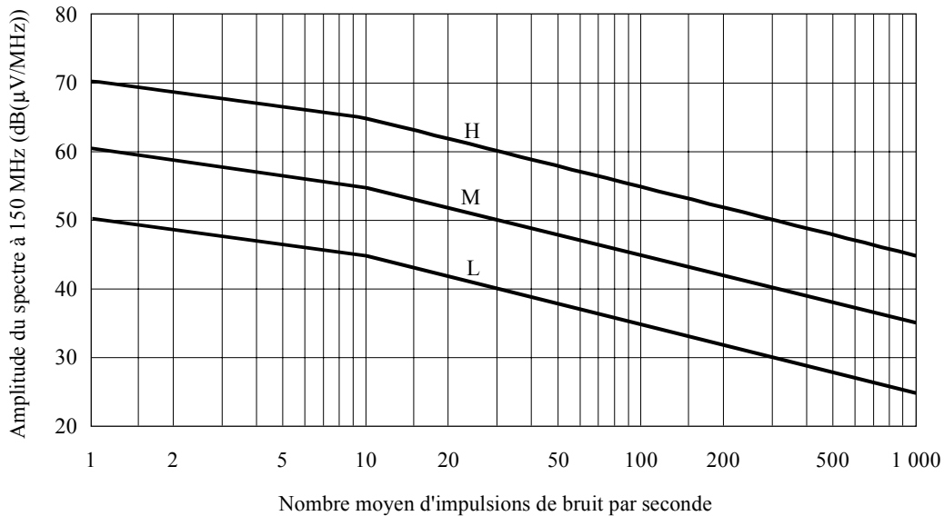
Répartition de l'amplitude du bruit dans une station de base (150 MHz)
