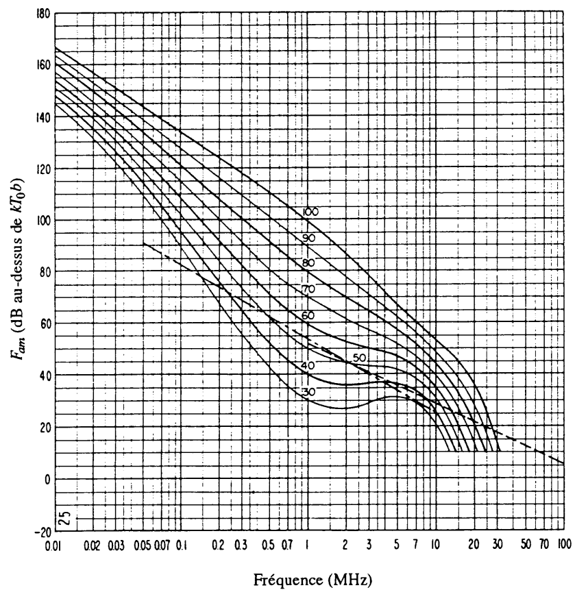
FIGURE 38b – Variation du bruit radioélectrique en fonction de la fréquence (Automne; 2000-2400 heure locale)
