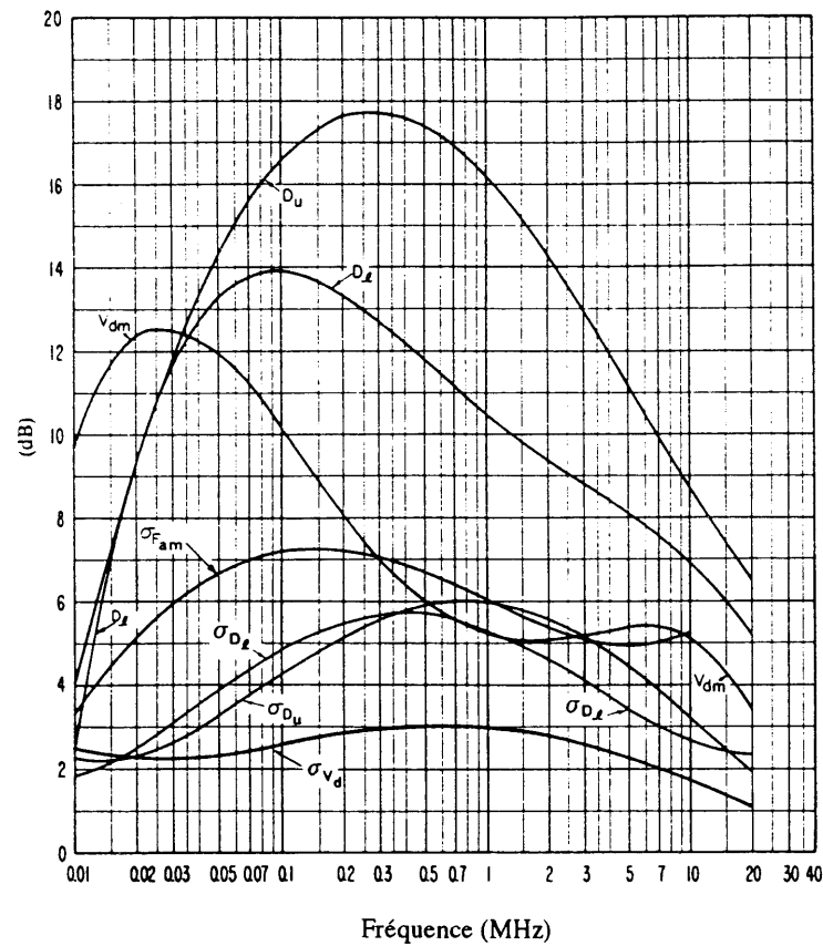
FIGURE 36c – Données sur la variabilité et le caractère du bruit (Automne; 1200-1600 heure locale)
