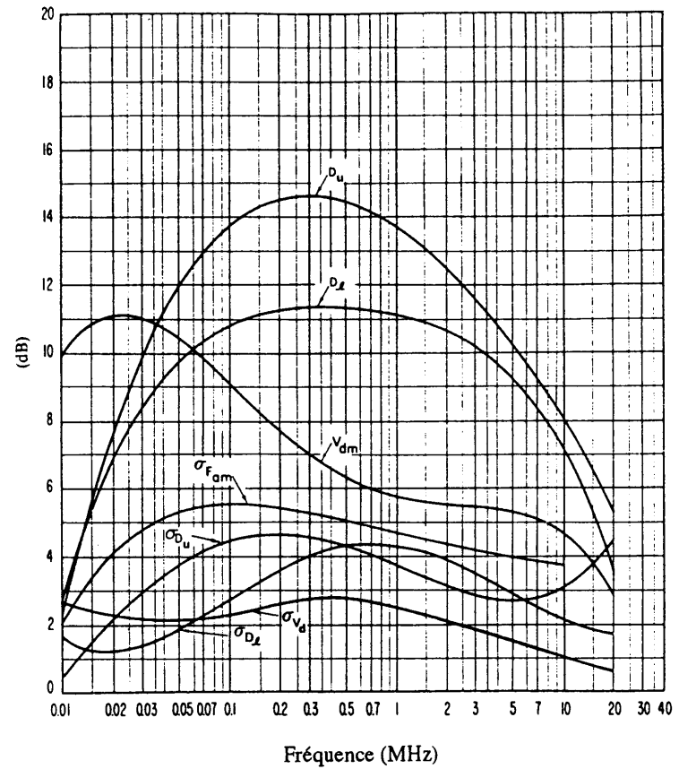
FIGURE 19c – Données sur la variabilité et le caractère du bruit (Hiver; 1600-2000 heure locale)
