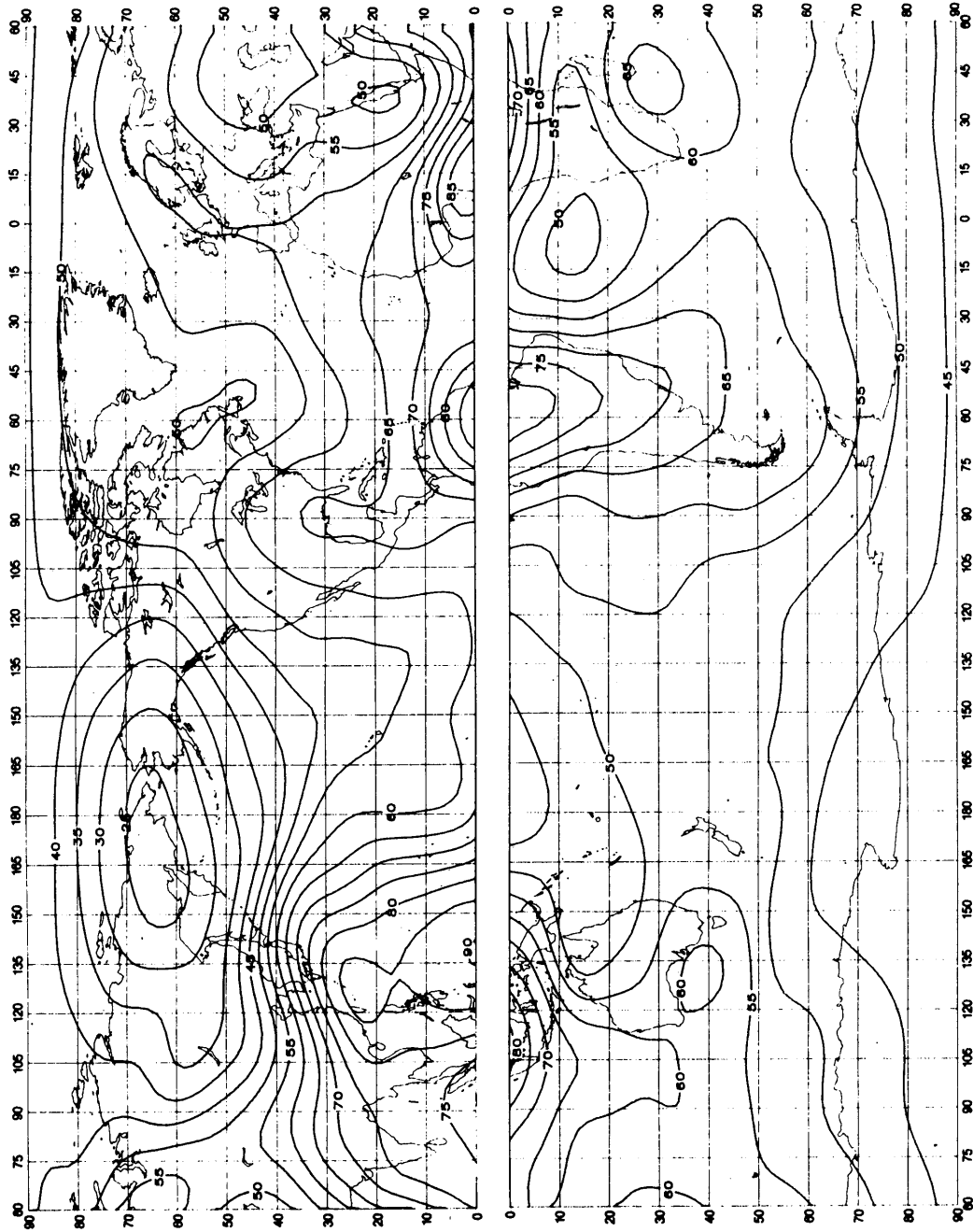
FIGURE 19a - Valeurs attendues du bruit atmosphérique radioélectrique, F_{fm} , en dB au-dessus de kT_0b à 1 MHz (Hiver; 1600-2000 heure locale)
