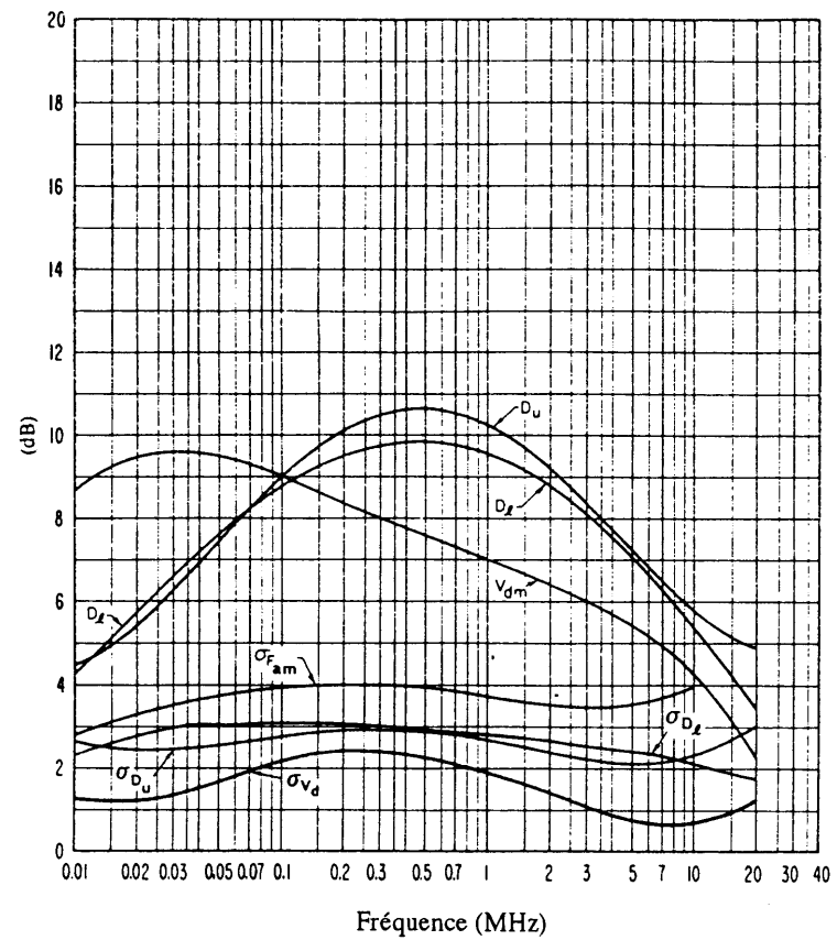
FIGURE 21c – Données sur la variabilité et le caractère du bruit (Printemps; 0000-0400 heure locale)
