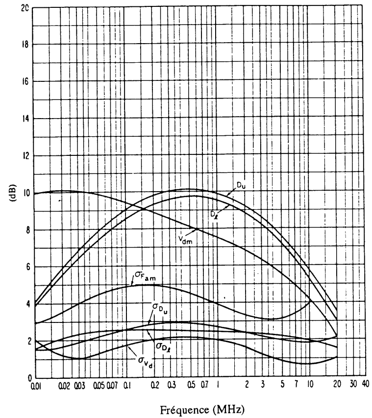
FIGURE 33c – Données sur la variabilité et le caractère du bruit (Automne; 0000-0400 heure locale)
