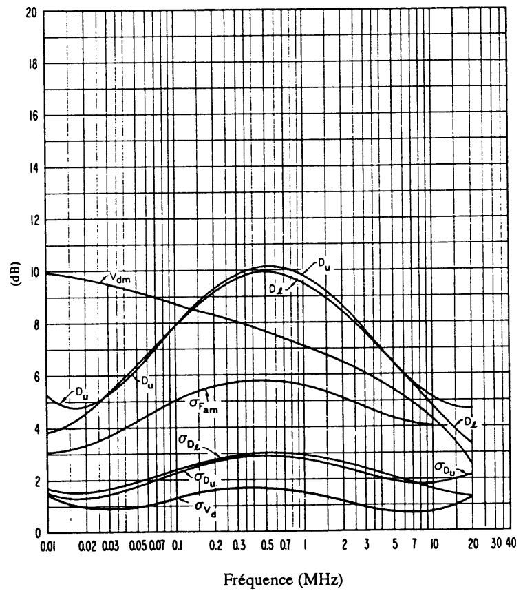
FIGURE 27c – Données sur la variabilité et le caractère du bruit (Eti; 0000-0400 heure locale)
