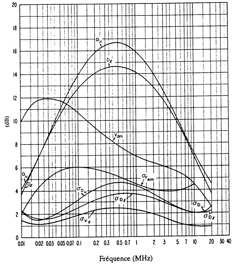
FIGURE 34c – Données sur la variabilité et le caractère du bruit (Automne; 0400-0800 heure locale)
