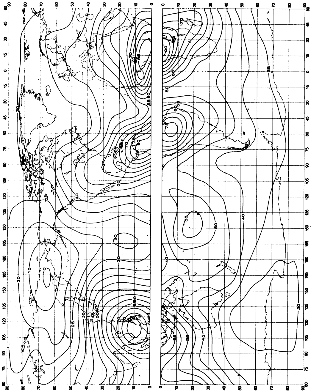
FIGURE 36a - Valeurs attendues du bruit atmospherique radioelectrique, F_{fm} , en dB au-dessus de kT_0b à 1 MHz (Automne; 1200-1600 heure locale)
