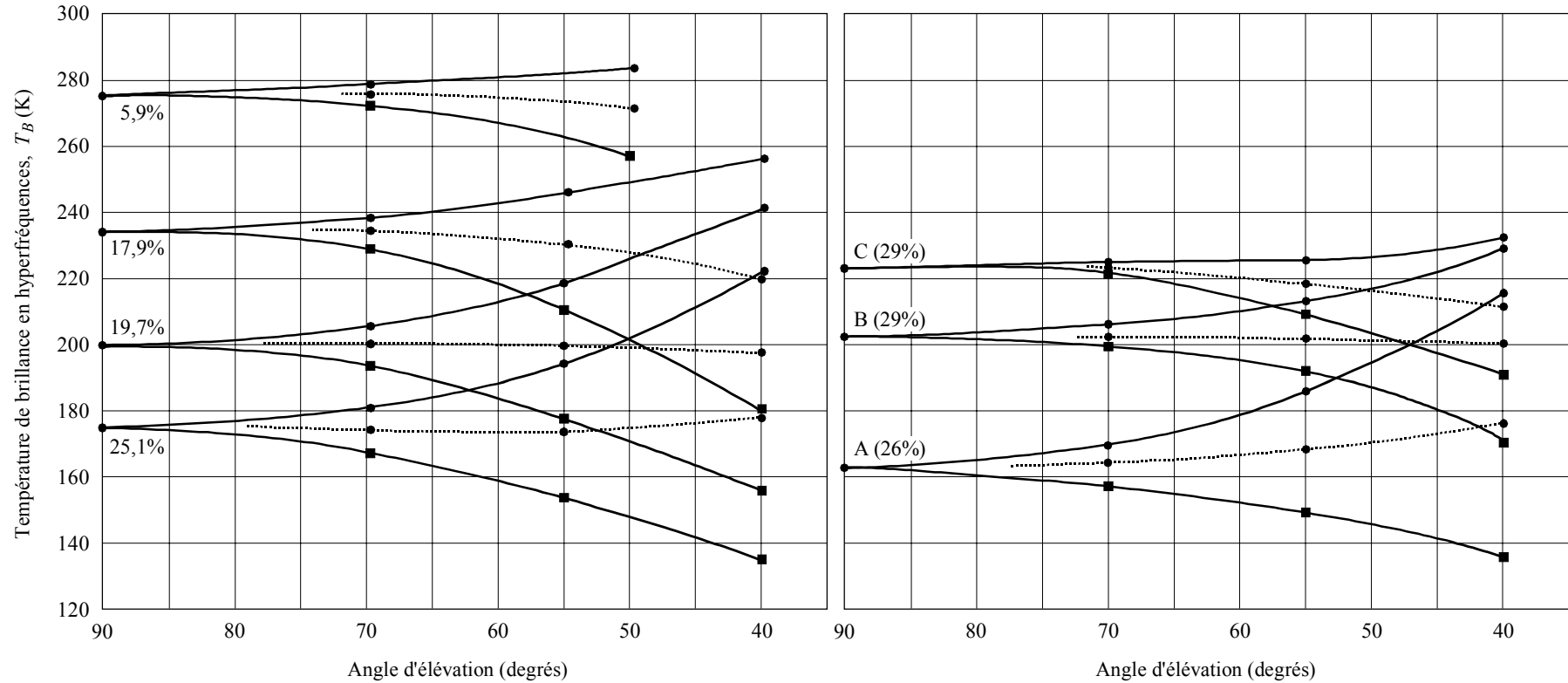
Température de brillance du sol (terre ferme) à 1 430 MHz en fonction de l'angle d'élévation
