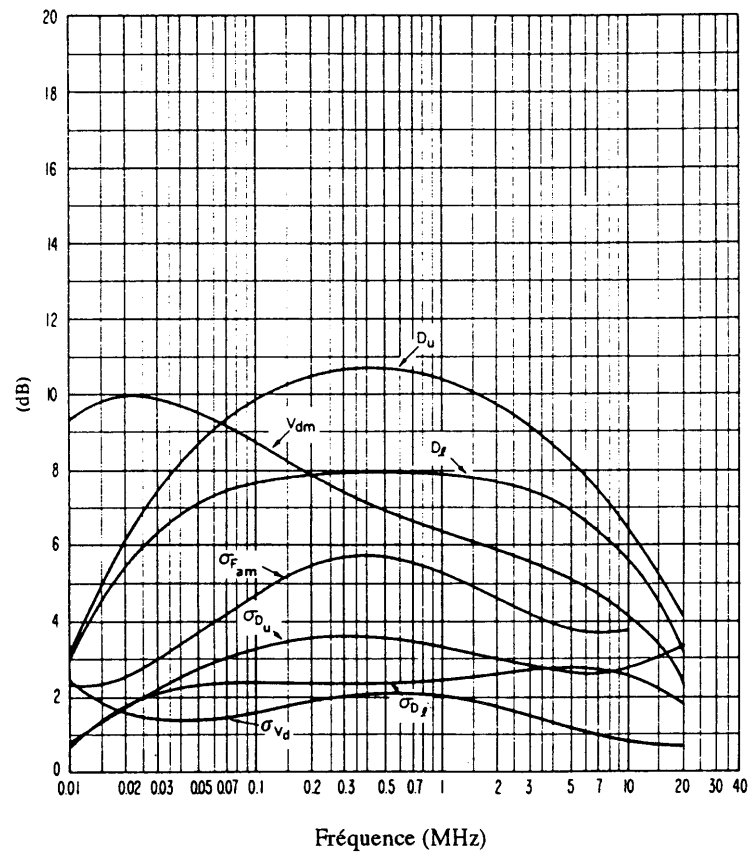
FIGURE 20c – Données sur la variabilité et le caractère du bruit (Hiver; 2000-2400 heure locale)
