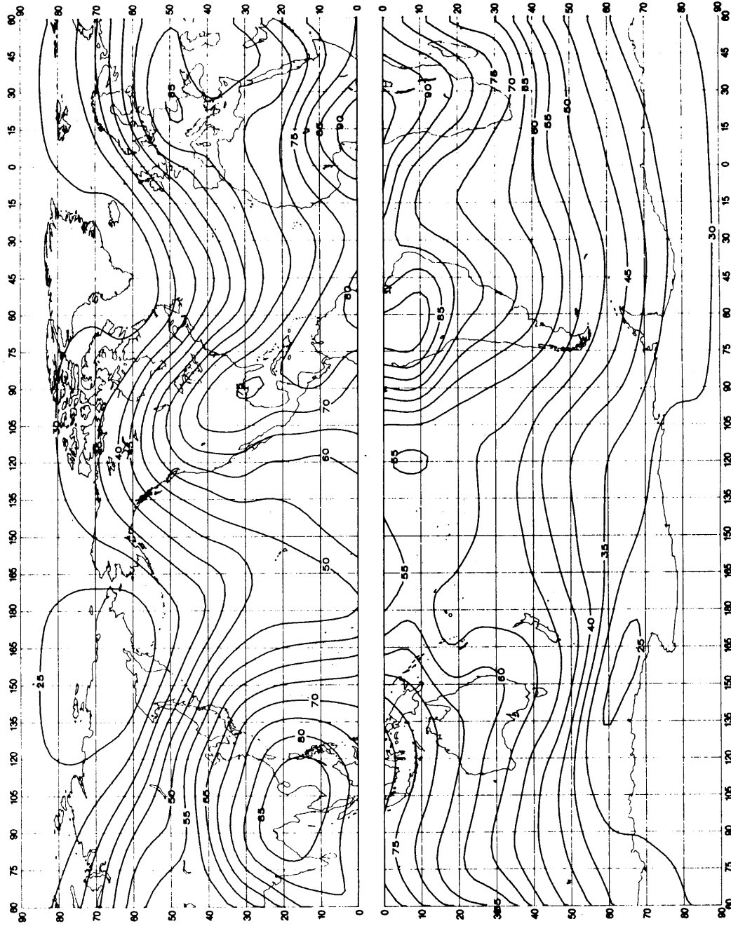
FIGURE 25a – Valeurs attendues du bruit atmosphérique radioélectrique, F_{em} , en dB au-dessus de kT_0b à 1 MHz (Printemps; 1600-2000 heure locale)
