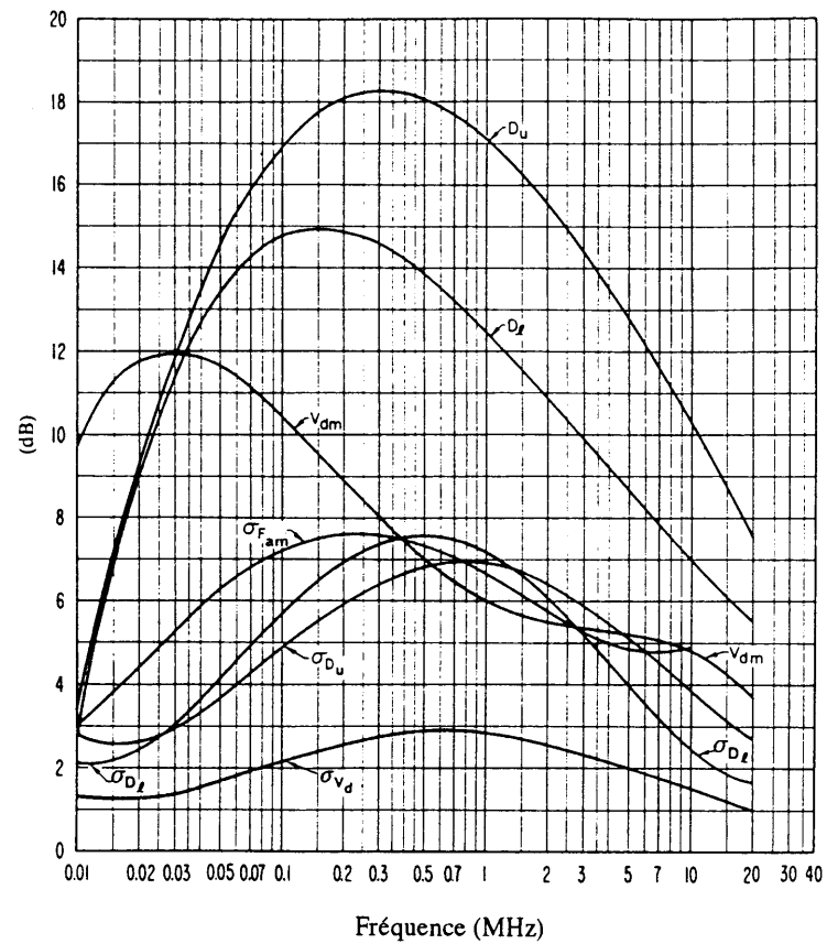
FIGURE 24c – Données sur la variabilité et le caractère du bruit (Printemps; 1200-1600 heure locale)
