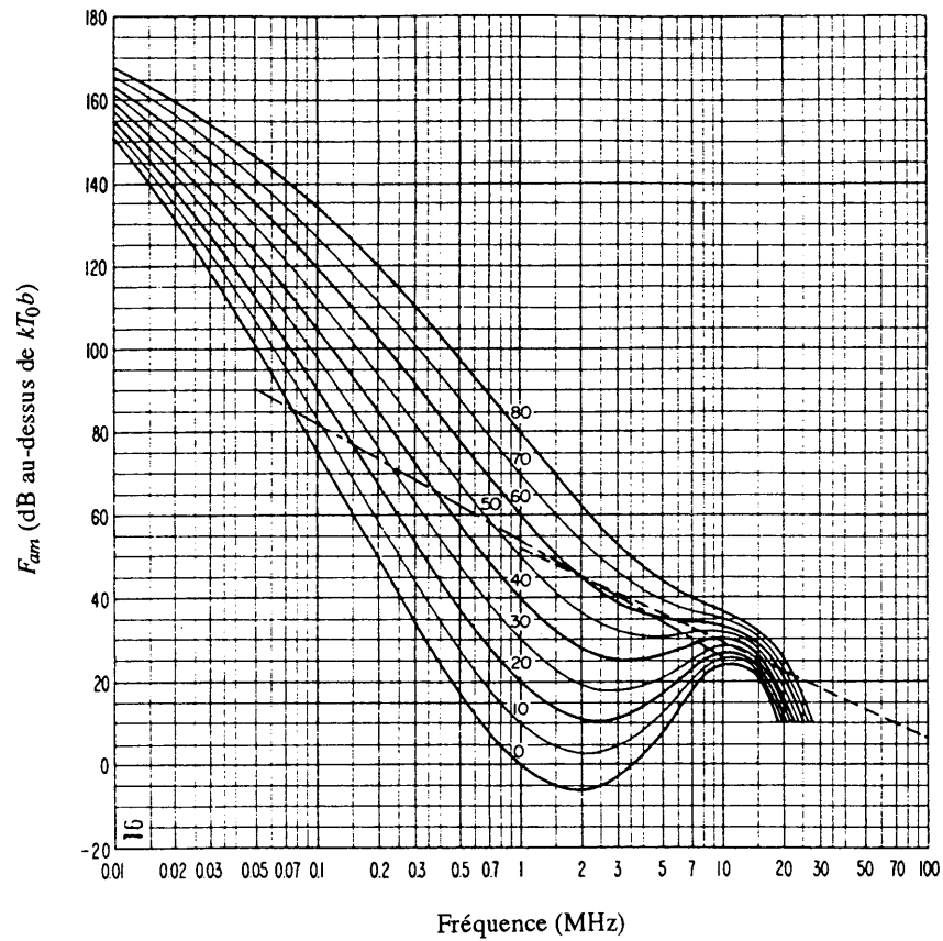
FIGURE 29b – Variation du bruit radioélectrique en fonction de la fréquence (Eté; 0800-1200 heure locale)
