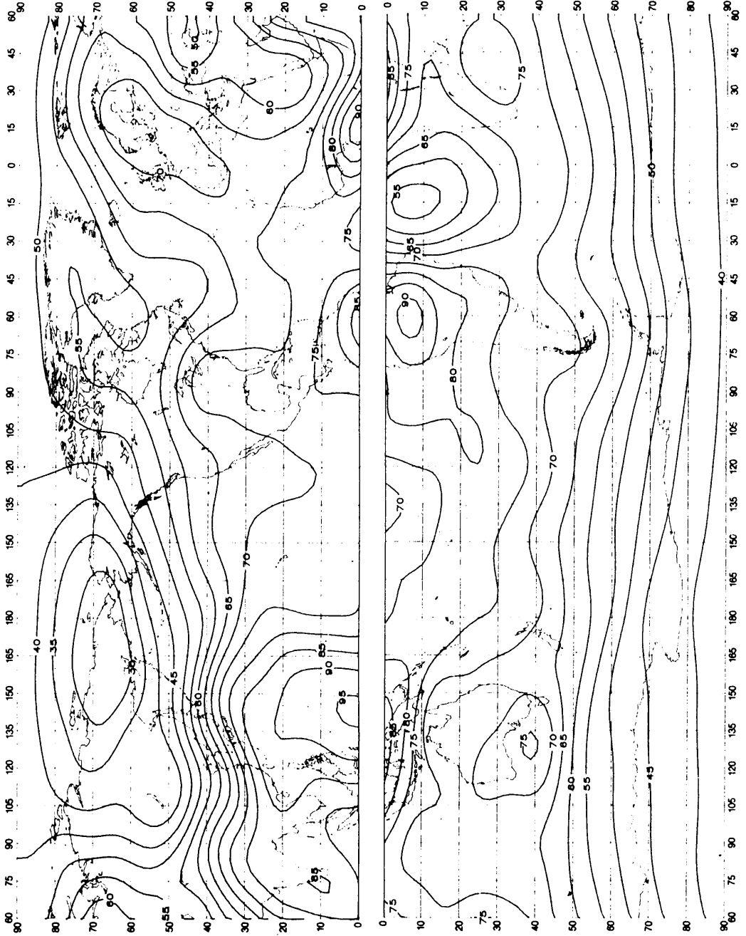
FIGURE 15a — Valeurs attendues du bruit atmospherique radioelectrique, F_{0.1m} , en dB au-dessus de kT_{0b} à 1 MHz (Hiver: 0000-0400 heure locale)
