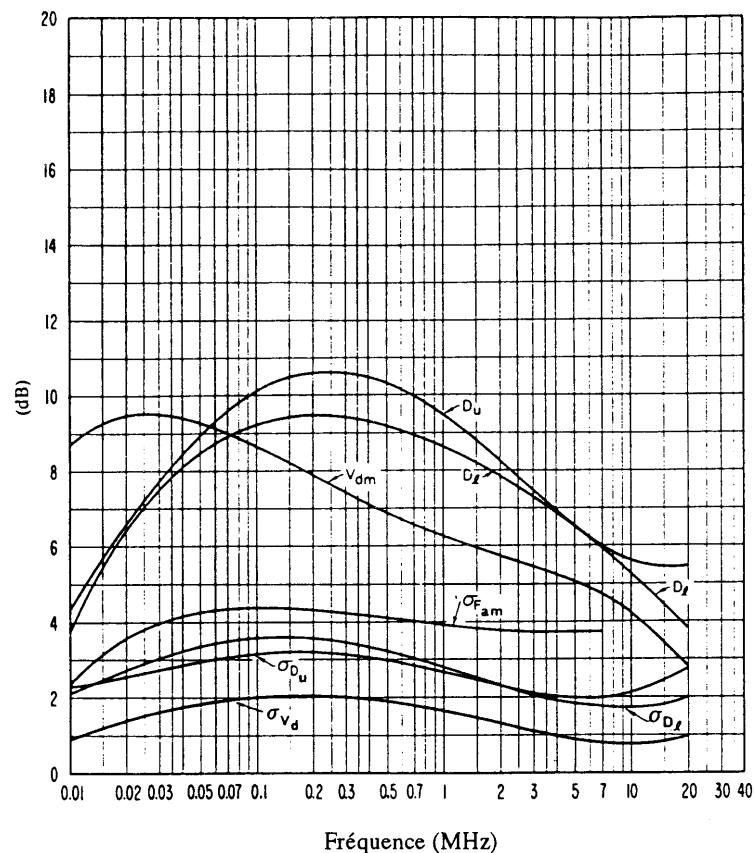
FIGURE 26c – Données sur la variabilité et le caractère du bruit (Printemps; 2000-2400 heure locale)
