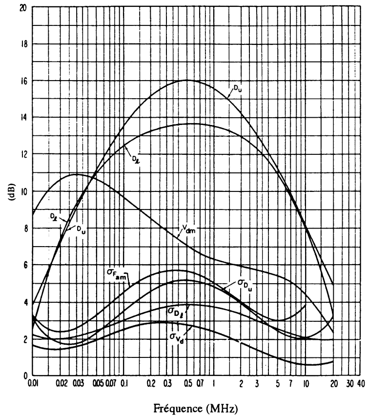
FIGURE 22c – Données sur la variabilité et le caractère du bruit (Printemps; 0400-0800 heure locale)
