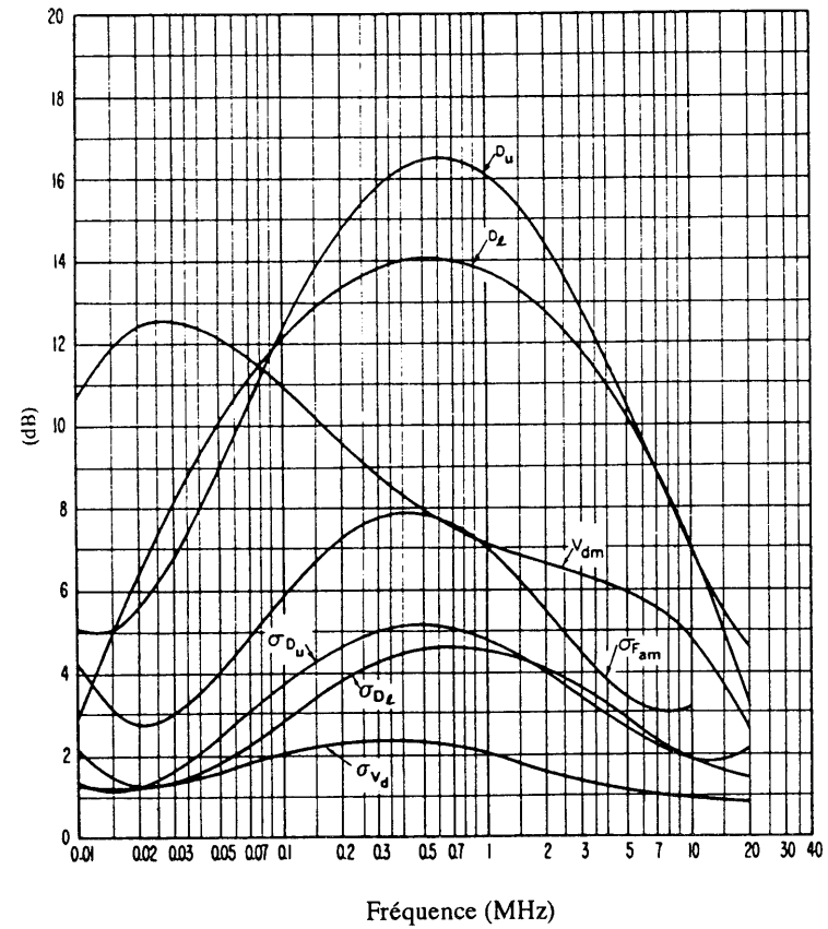
FIGURE 28c – Données sur la variabilité et le caractère du bruit (Eté; 0400-0800 heure locale)
