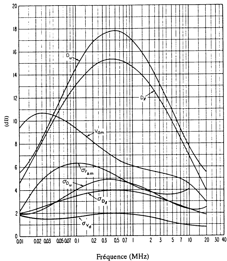
FIGURE 37c – Données sur la variabilité et le caractère du bruit (Automne; 1600-2000 heure locale)
