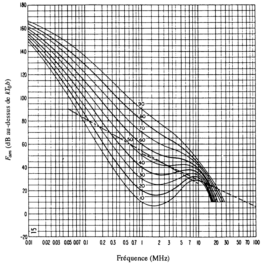
FIGURE 28b – Variation du bruit radioélectrique en fonction de la fréquence (Eté; 0400-0800 heure locale)
