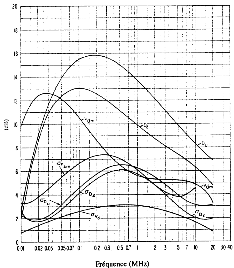
FIGURE 23c – Données sur la variabilité et le caractère du bruit (Printemps; 0800-1200 heure locale)
