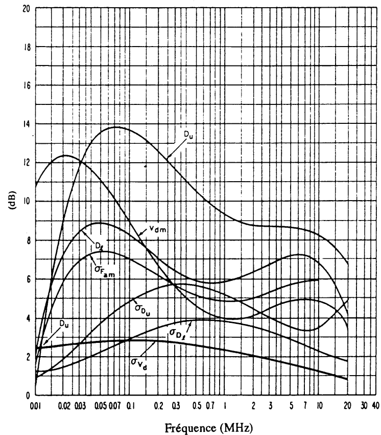
FIGURE 18c – Données sur la variabilité et le caractère du bruit (Hiver; 1200-1600 heure locale)
