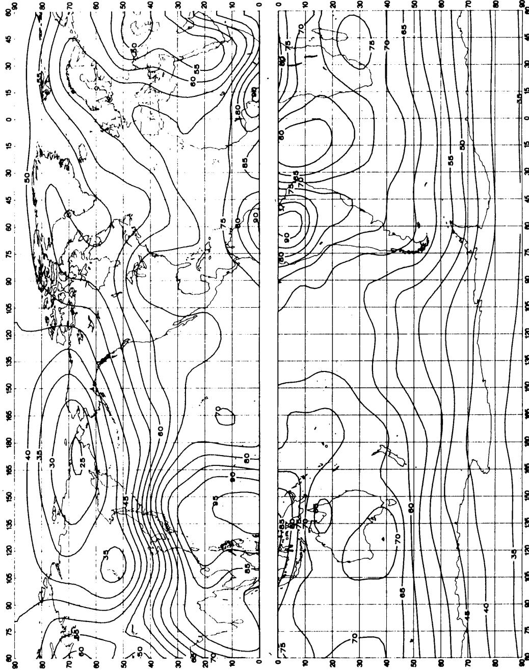
FIGURE 20a – Valeurs attendues du bruit atmosphérique radioélectrique, F_{0b} , en dB au-dessus de kT_0b à 1 MHz (Hiver; 2000-2400 heure locale)
