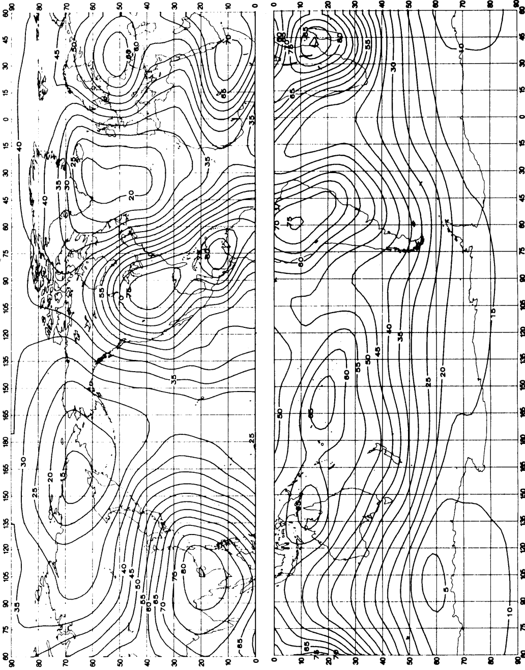
FIGURE 30a – Valeurs attendues du bruit atmosphérique radioélectrique, F_{0.1} , en dB au-dessus de kT_{0b} à 1 MHz (Eie; 1200-1600 heure locale)
