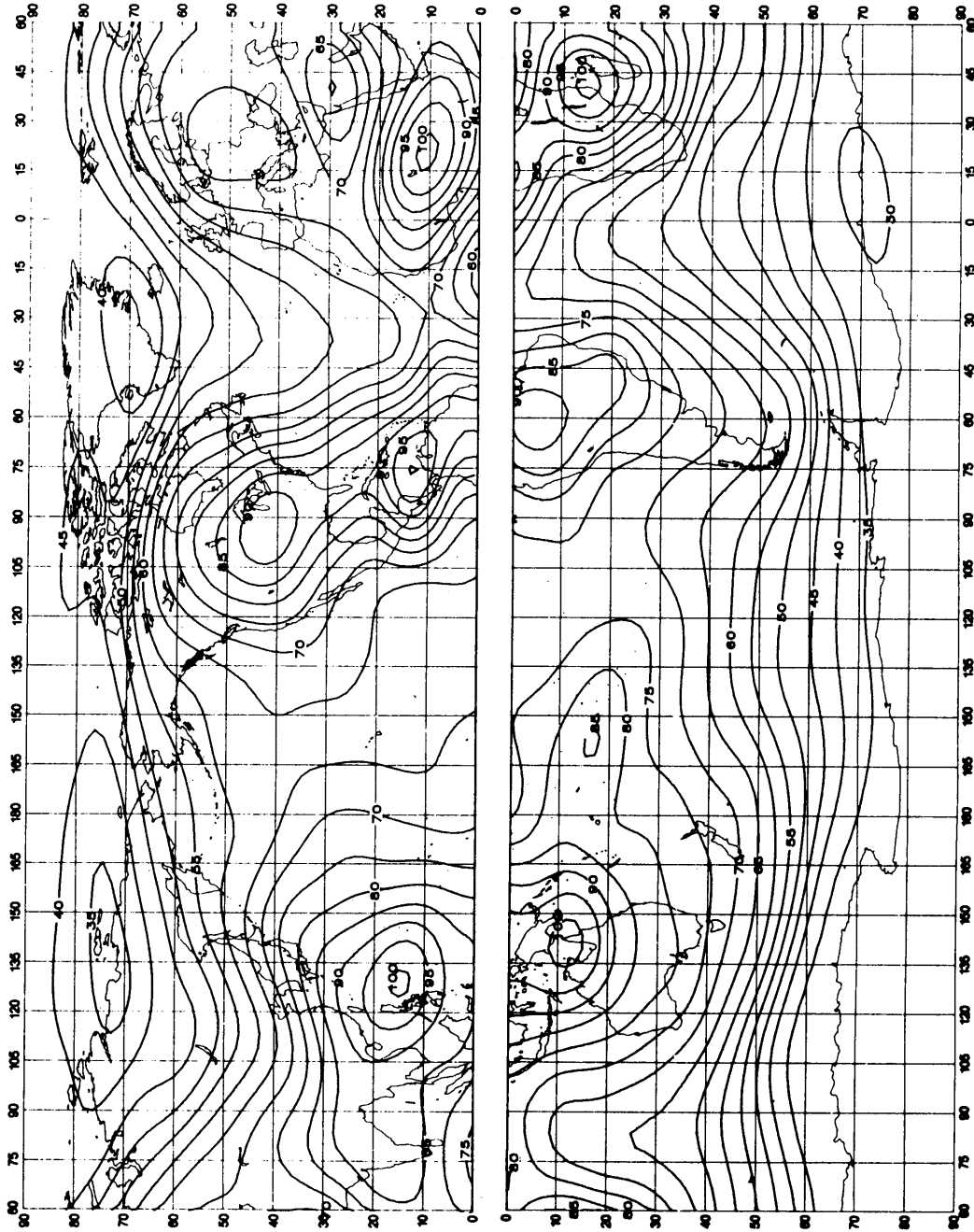
FIGURE 32a -- Valeurs attendues du bruit atmosphérique radioélectrique, F_{0.1M} , en dB au-dessus de kT_{0b} à 1 MHz (Eté; 2000-2400 heure locale)
