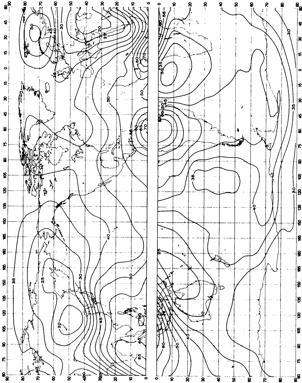
FIGURE 18a – Valeurs attendues du bruit atmosphérique radioélectrique, F_{0.1} , en dB au-dessus de kT_{0b} à 1 MHz (Hiver, 1200-1600 heure locale)
