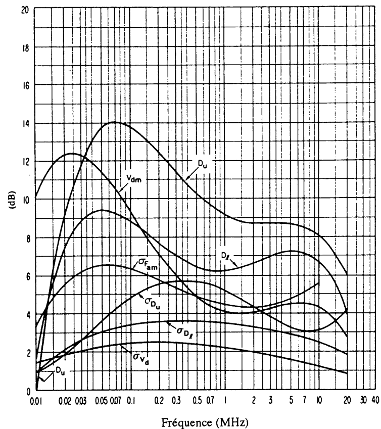
FIGURE 17c – Données sur la variabilité et le caractère du bruit (Hiver; 0800-1200 heure locale)
