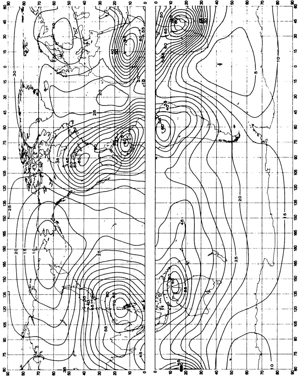
FIGURE 29a – Valeurs attendues du bruit atmosphérique radioélectrique, F_{am} , en dB au-dessus de kT_0b à 1 MHz (Eié; 0800-1200 heure locale)
