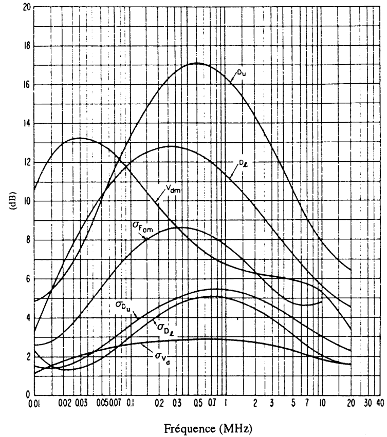
FIGURE 29c – Données sur la variabilité et le caractère du bruit (Eté; 0800-1200 heure locale)
