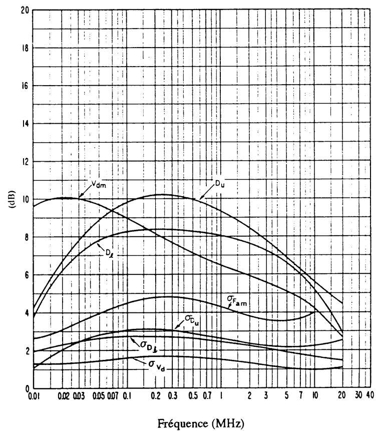
FIGURE 38c – Données sur la variabilité et le caractère du bruit (Automne; 2000-2400 heure locale)
