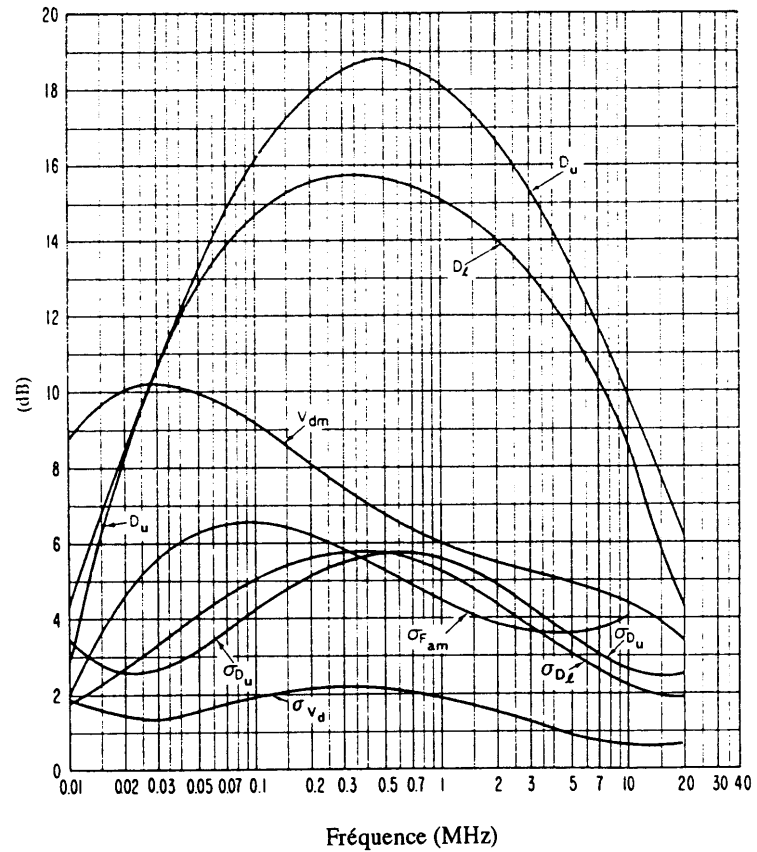
FIGURE 25c – Données sur la variabilité et le caractère du bruit (Printemps; 1600-2000 heure locale)
