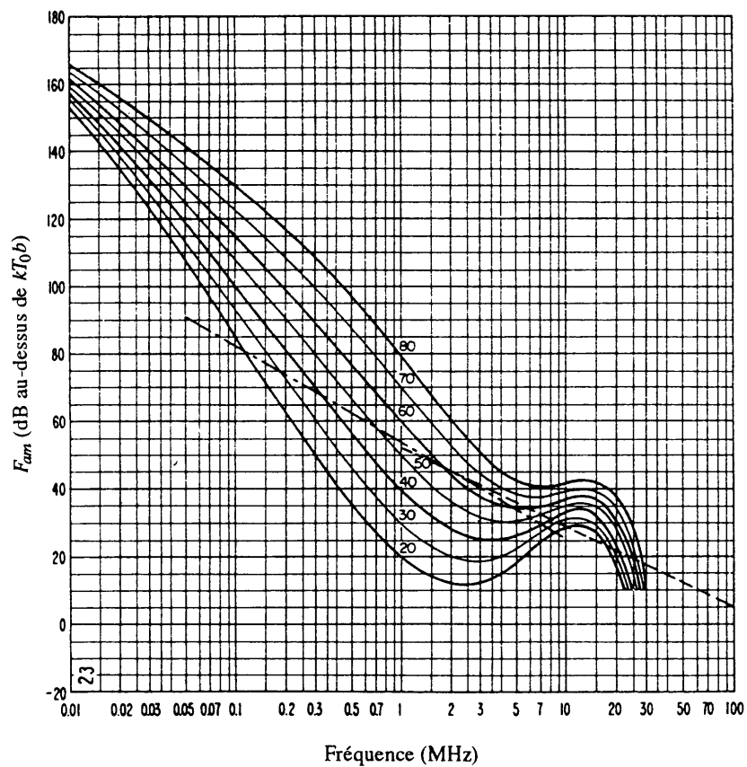
FIGURE 36b – Variation du bruit radioélectrique en fonction de la fréquence (Automne; 1200-1600 heure locale)
