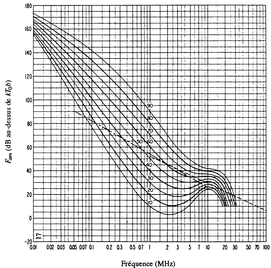
FIGURE 30b – Variation du bruit radioélectrique en fonction de la fréquence (Eté; 1200-1600 heure locale)
