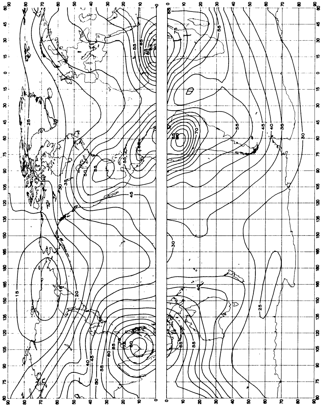
FIGURE 24a - Valeurs attendues du bruit atmosphérique radioélectrique, F_{am} , en dB au-dessus de kT_0b à 1 MHz (Printemps; 1200-1600 heure locale)
