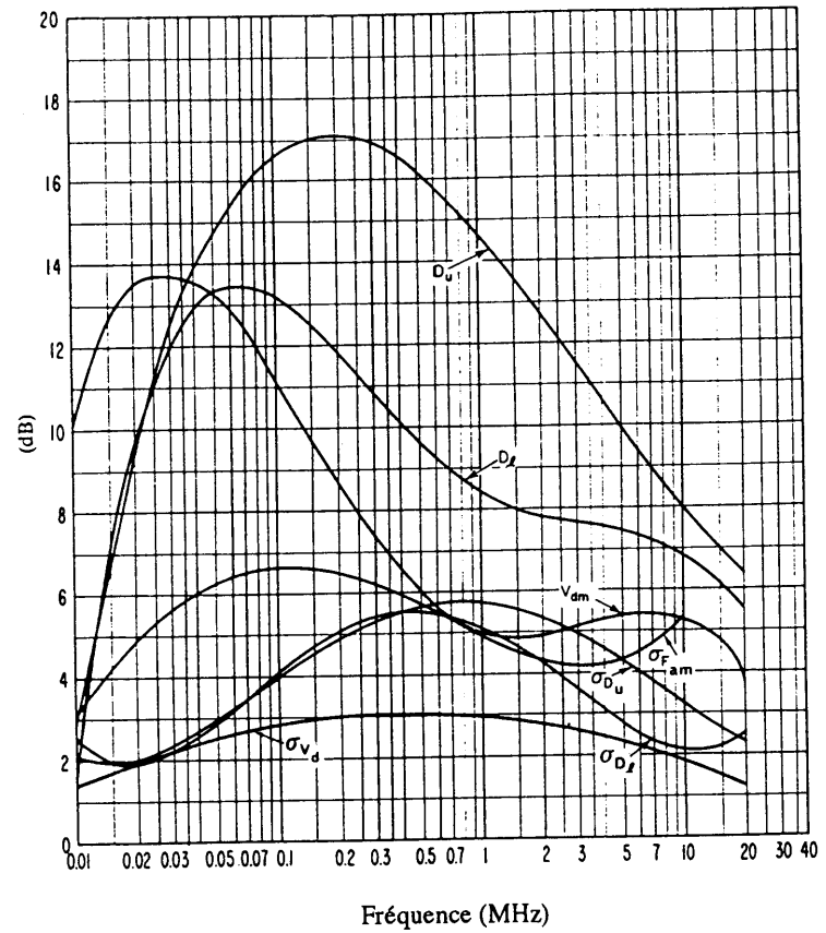
FIGURE 35c – Données sur la variabilité et le caractère du bruit (Automne; 0800-1200 heure locale)
