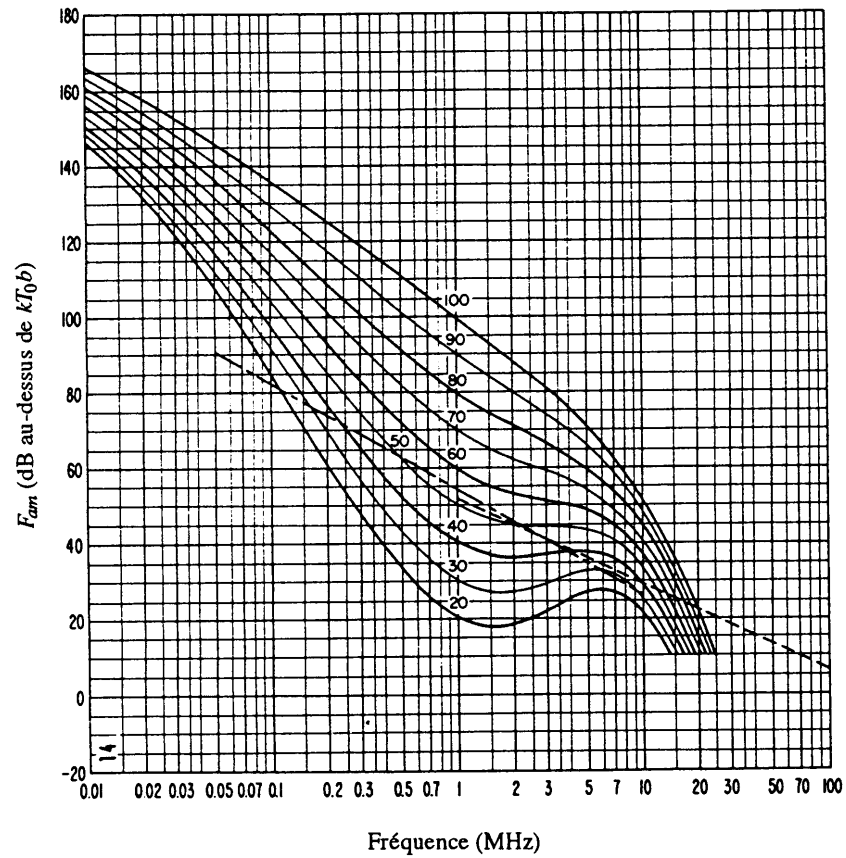
FIGURE 27b – Variation du bruit radioélectrique en fonction de la fréquence (Eti; 0000-0400 heure locale)
