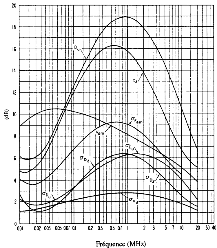
FIGURE 30c – Données sur la variabilité et le caractère du bruit (Eté; 1200-1600 heure locale)
