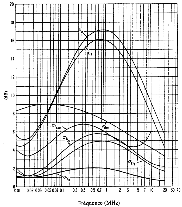
FIGURE 31c – Données sur la variabilité et le caractère du bruit (Eté; 1600-2000 heure locale)
