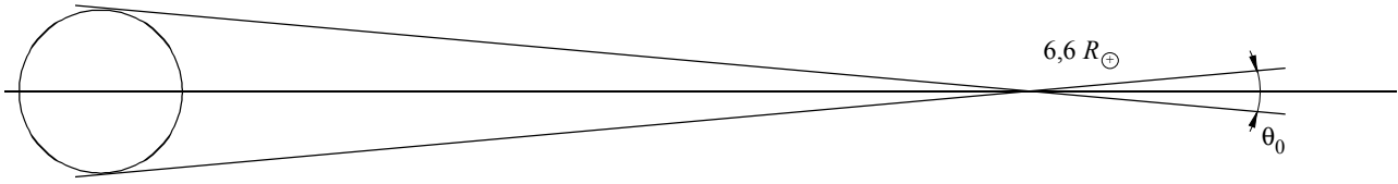
Tierra a) La órbita de los satélites geostacionarios vista desde la Tierra mostrando \theta_0 ( R_{\oplus} : radio medio de la Tierra)
