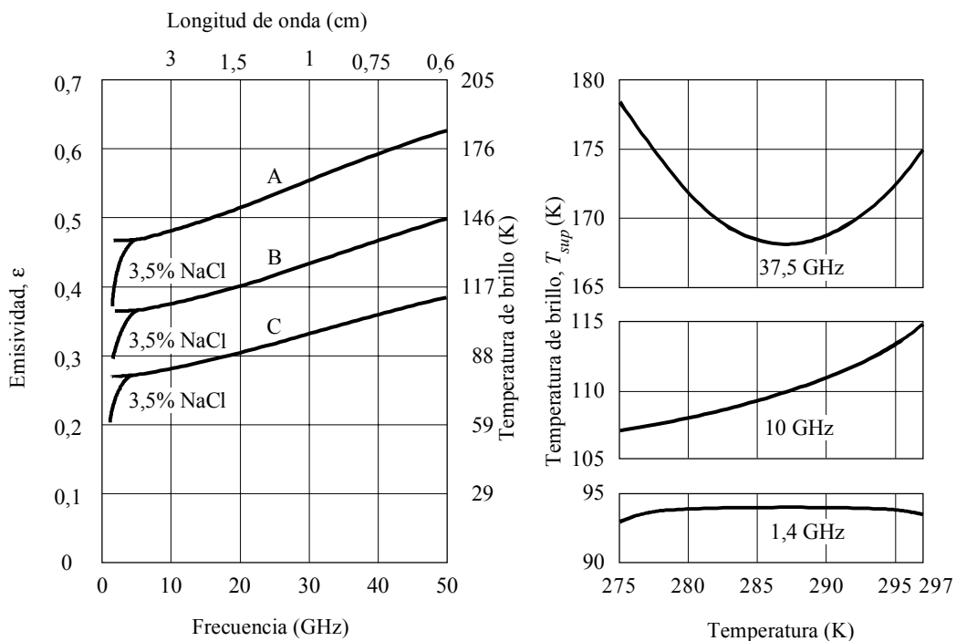
a) Emisividad de una superficie de agua lisa
