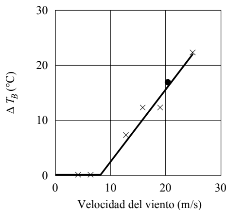
d) Incremento de la temperatura de brillo de la superficie del océano a 19,35 GHz debido a la velocidad del viento
