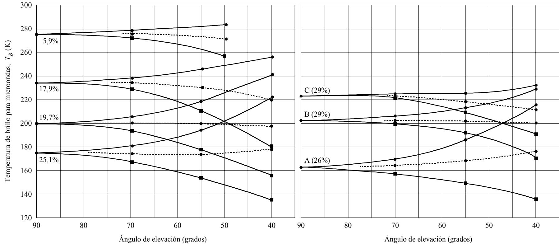
Temperatura de brillo del suelo a 1 430 MHz, en función del ángulo de elevación
