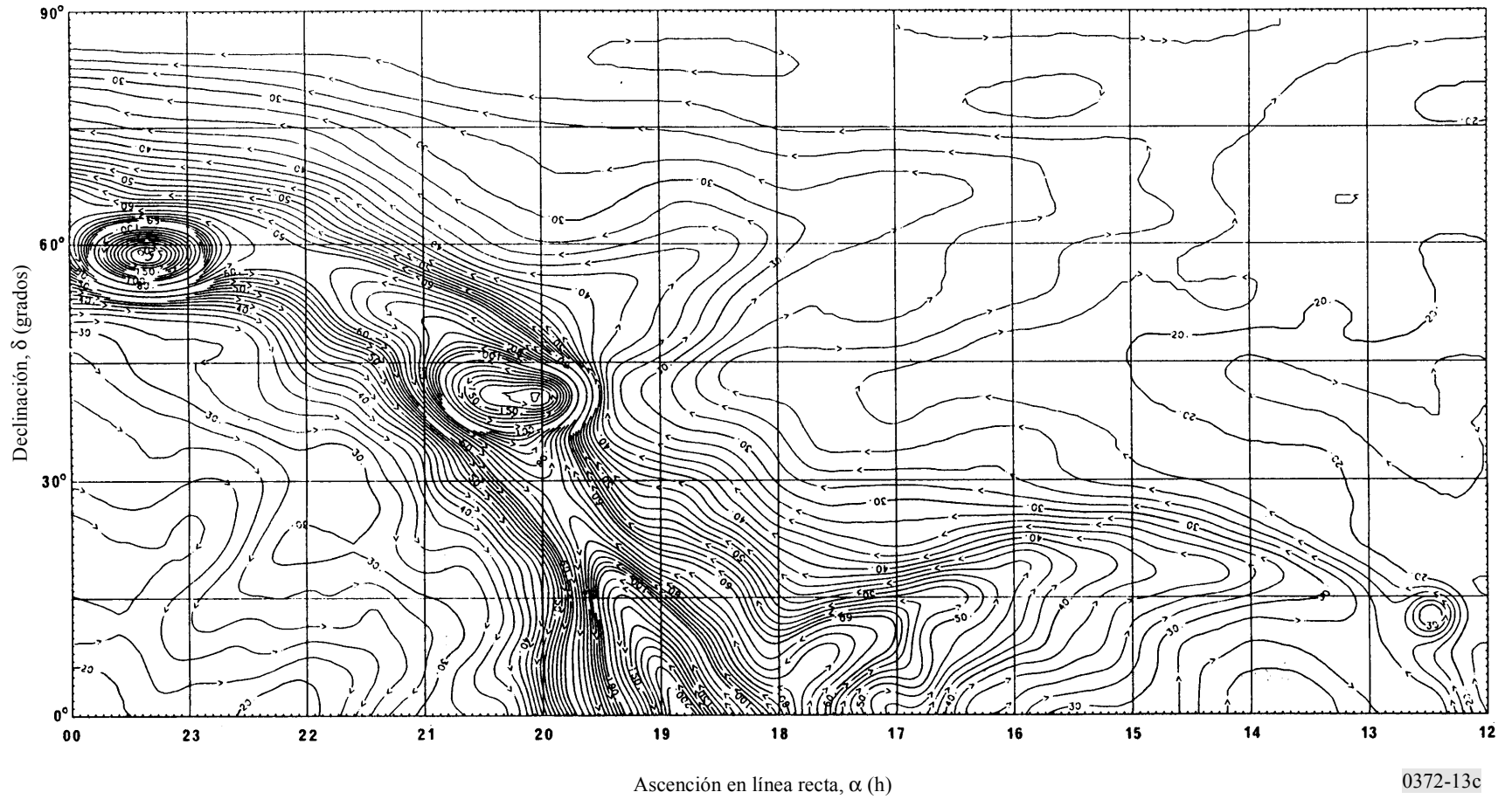
FIGURA 13c Temperatura del cielo radioelctrico a 408 MHz
