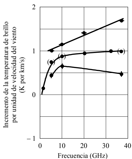
c) Espectro del incremento de la temperatura de brillo causado por el viento en la superficie del océano
