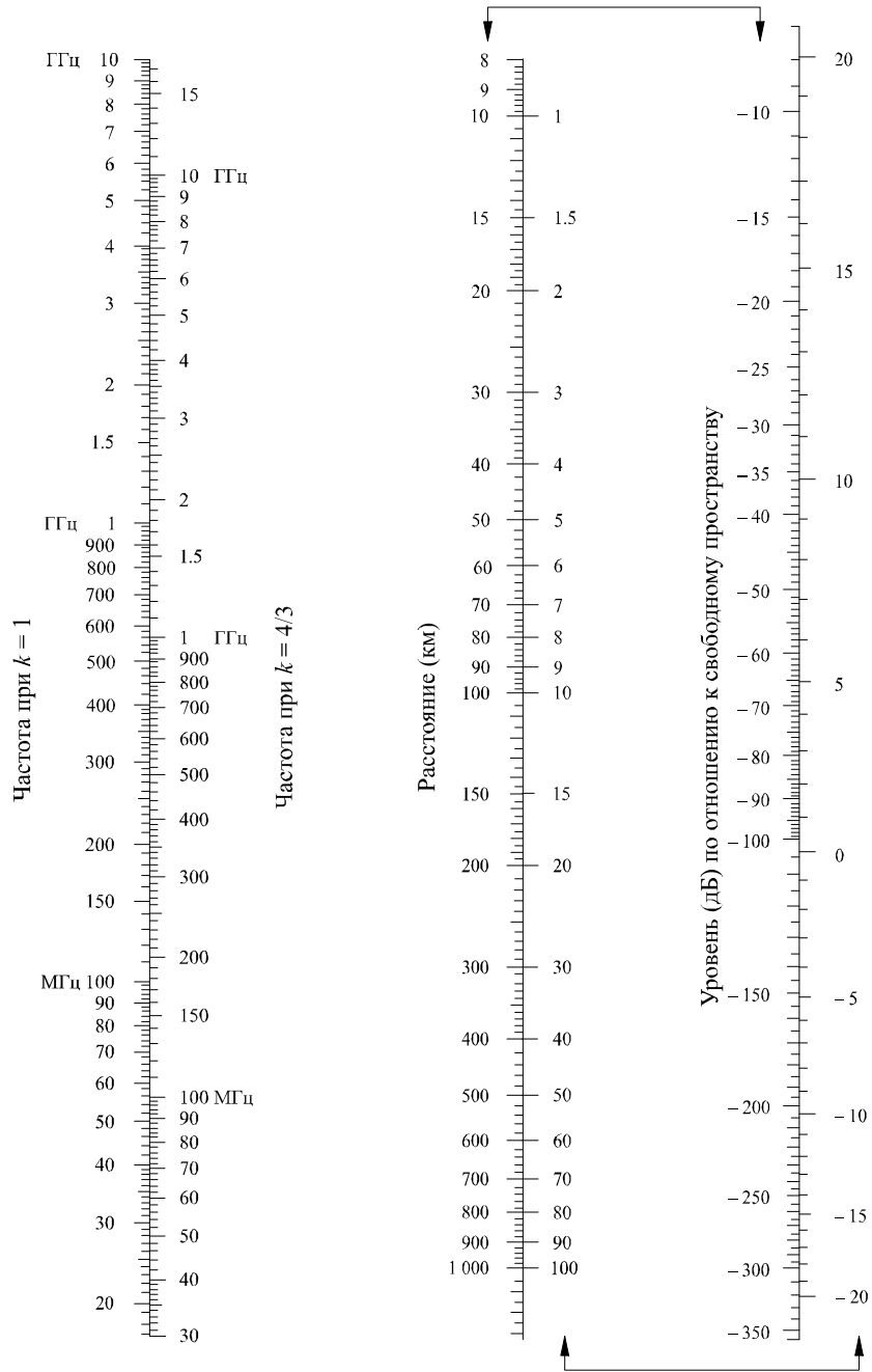
РИСУНОК 3 Дифракция над сферической Землей – влияние расстояния
