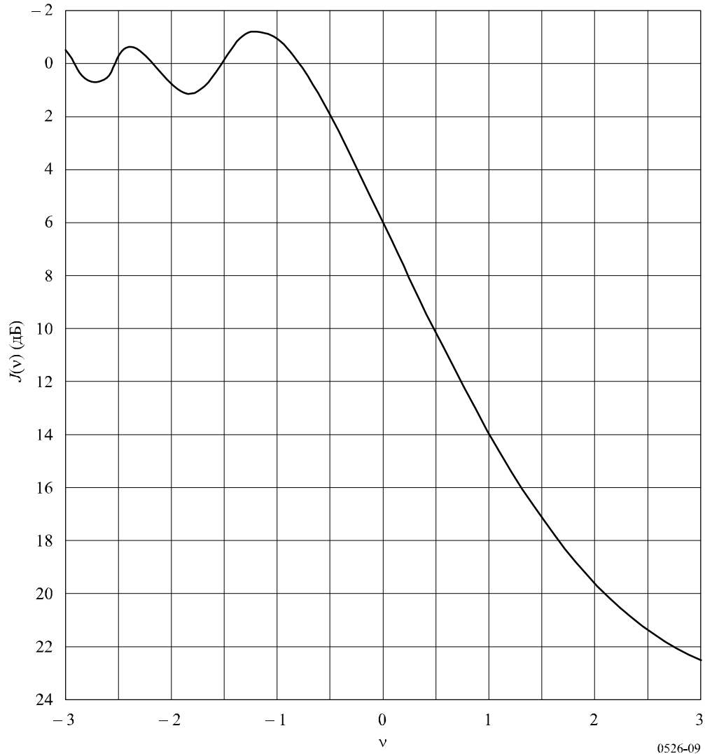
Дифракционные потери на клиновидном препятствии
