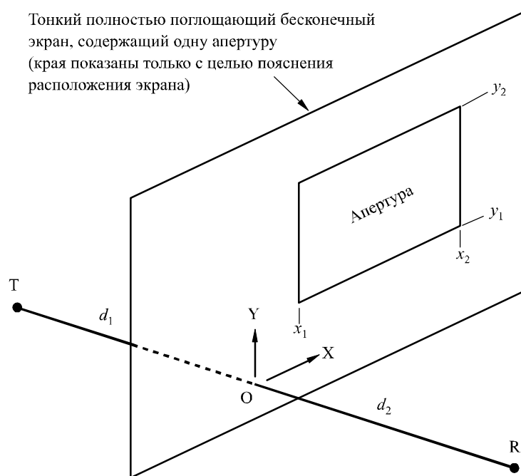
Геометрия для единичной прямоугольной апертуры
