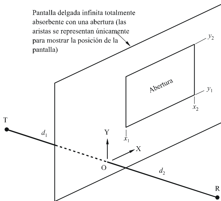
Geometría para una abertura rectangular única
