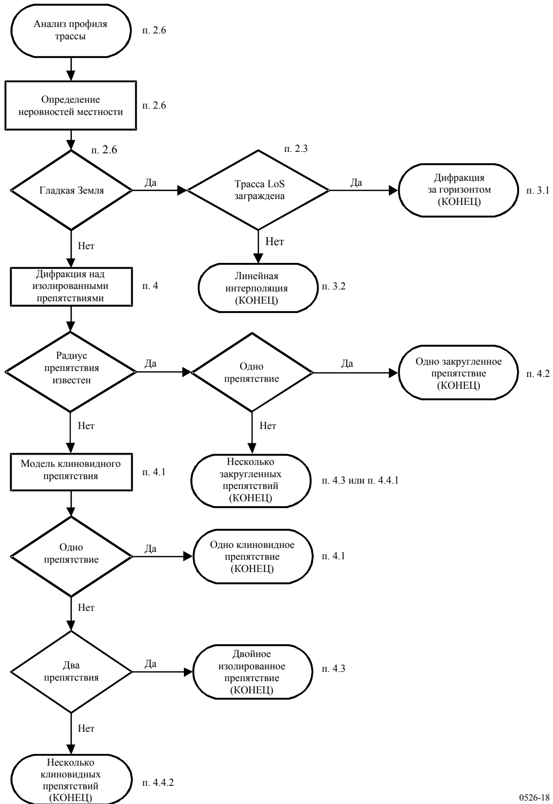
РИСУНОК 18 Руководство по распространению путем дифракции
