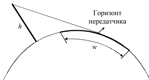
РИСУНОК 1 Определение ширины области полутени
