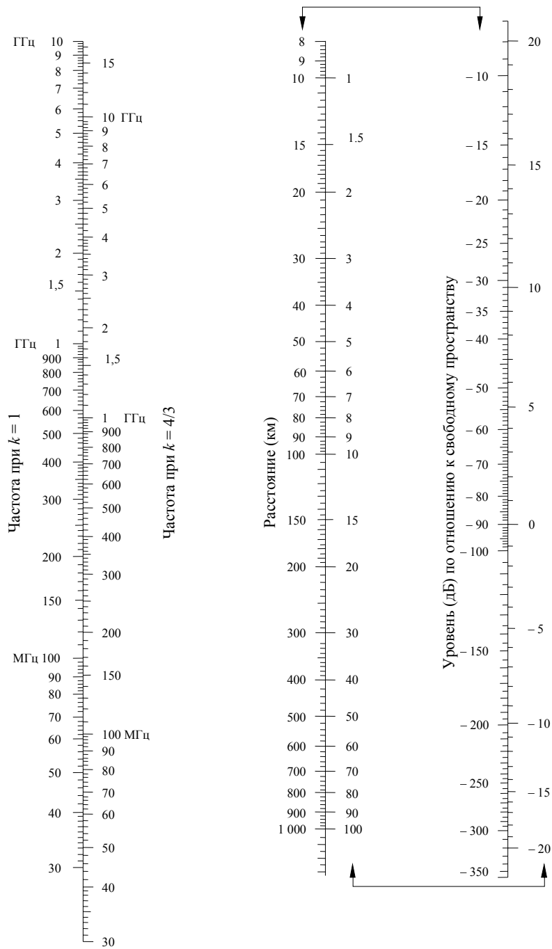
РИСУНОК 5 Дифракция над сферической Землей – влияние расстояния
