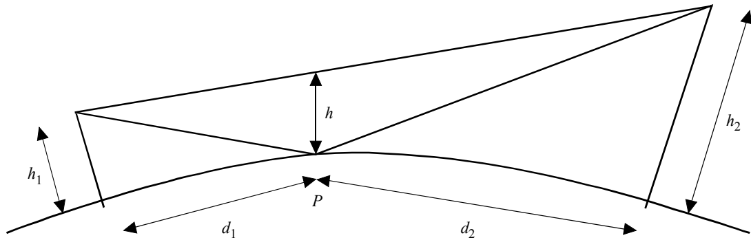
РИСУНОК 7 Просвет трассы
