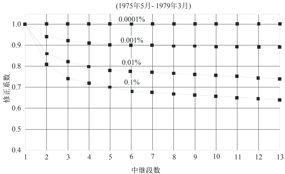
图7 对于每一链路的几种超过概率水平，每中继段长度约为4.6 km的一 系列串接中继段的总雨衰的修正系数
