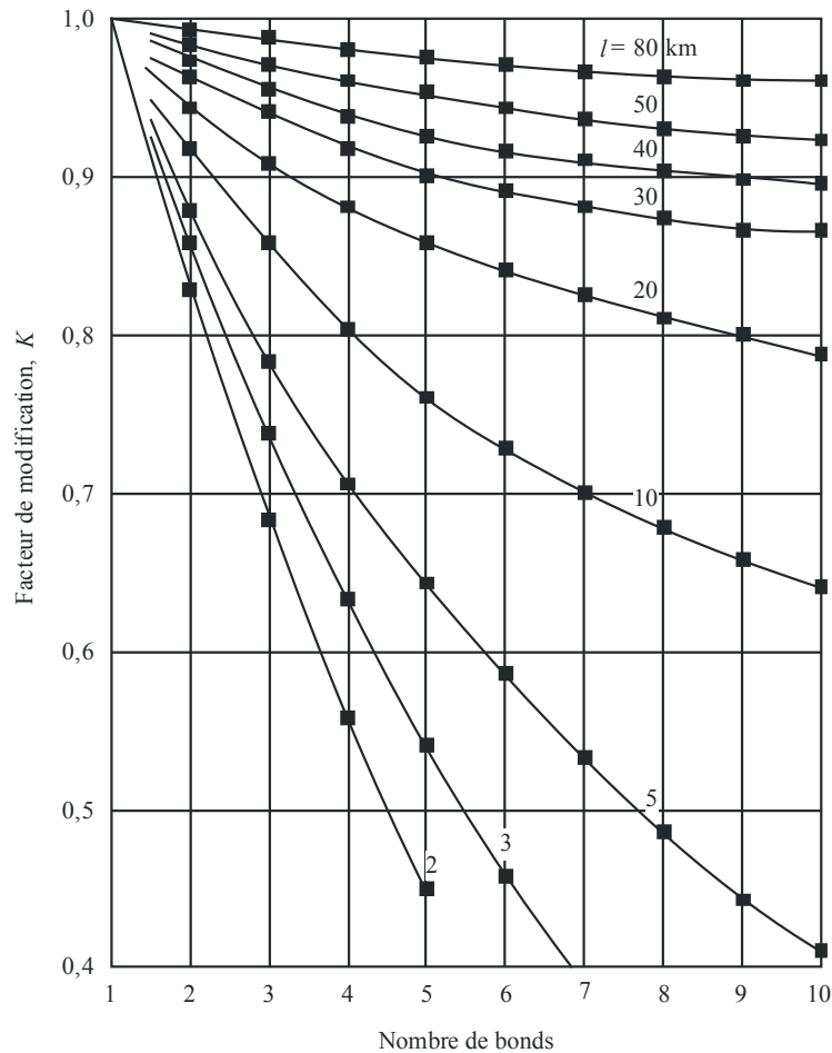
FIGURE 5 Facteur de modification pour l'affaiblissement conjoint dû à la pluie pour une série de bonds en cascade, tous de même longueur, l pour une probabilité de dépassement de 0,03% pour chaque bond
